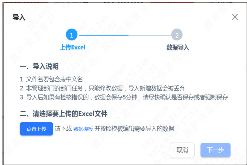
图 3-39 导入
