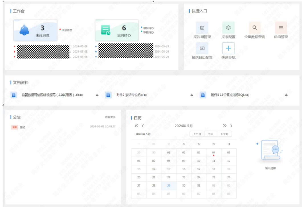
图 3-2 体系首页
