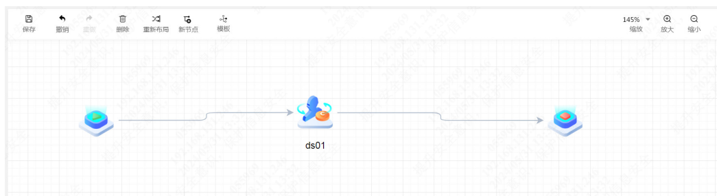
图 3-118 流程图
