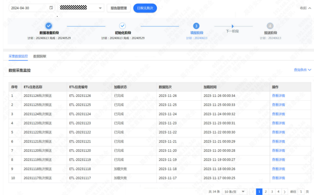
图 3-11 管理工作台
