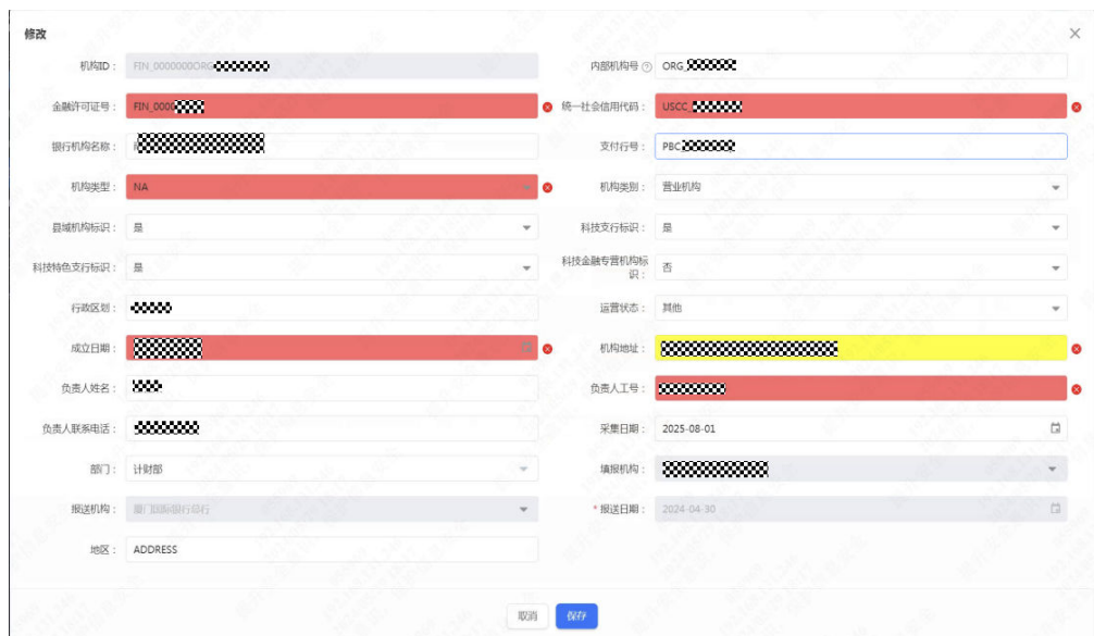
图 3-36 修改
