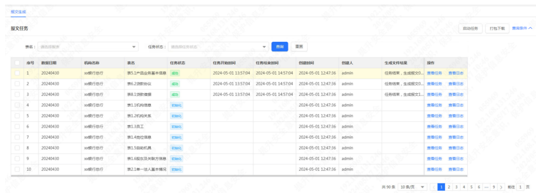
图 3-32 报送任务
