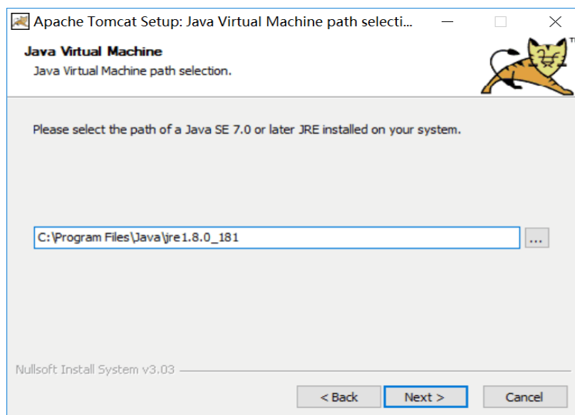
图 3-11 继续安装
