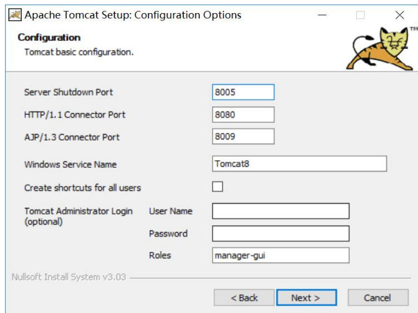
图 3-10 Next
