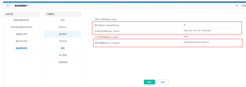
图 3-21 参数配置 3
