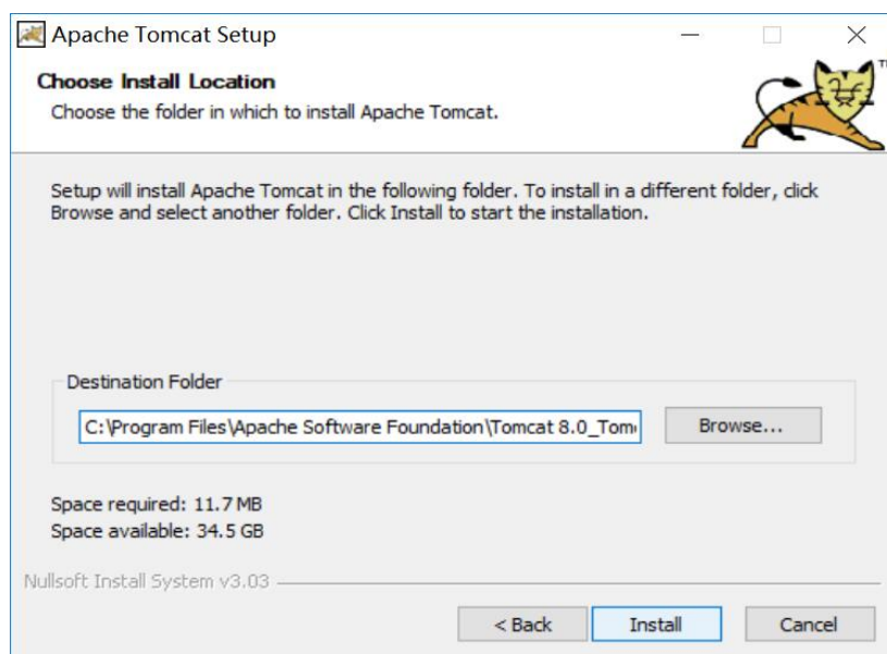
图 3-12 Next
