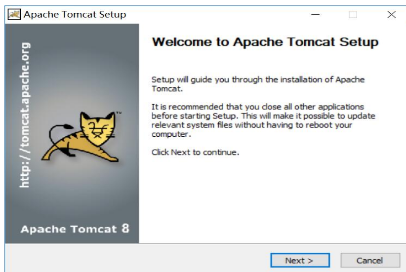
图 3-7 Tomcat8 安装
