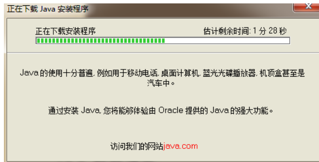
图 3-2 JDK 安装 2
