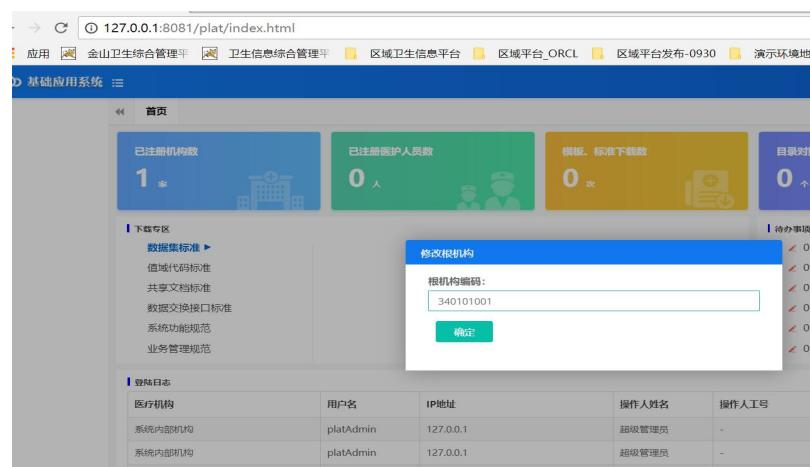
图 3-19 参数配置 1
