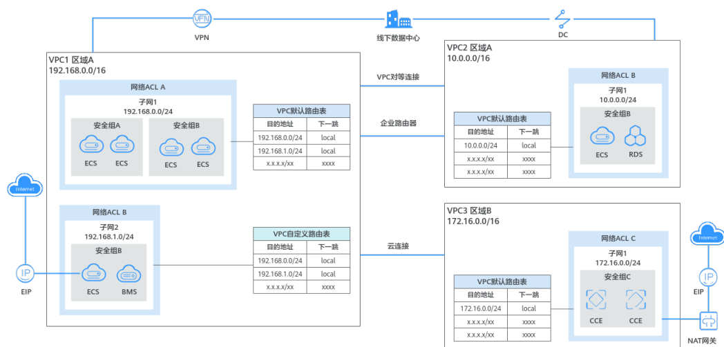
图 3-1 VPC 产品架构
