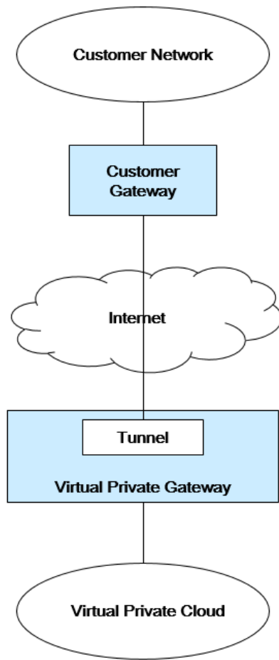
图 8-26 VPN 网络示意图
