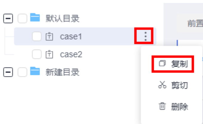
图 6-16 复制用例
