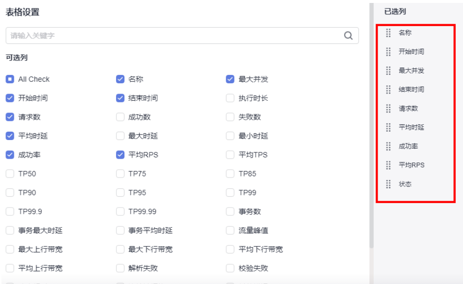
图 8-2 表格设置
