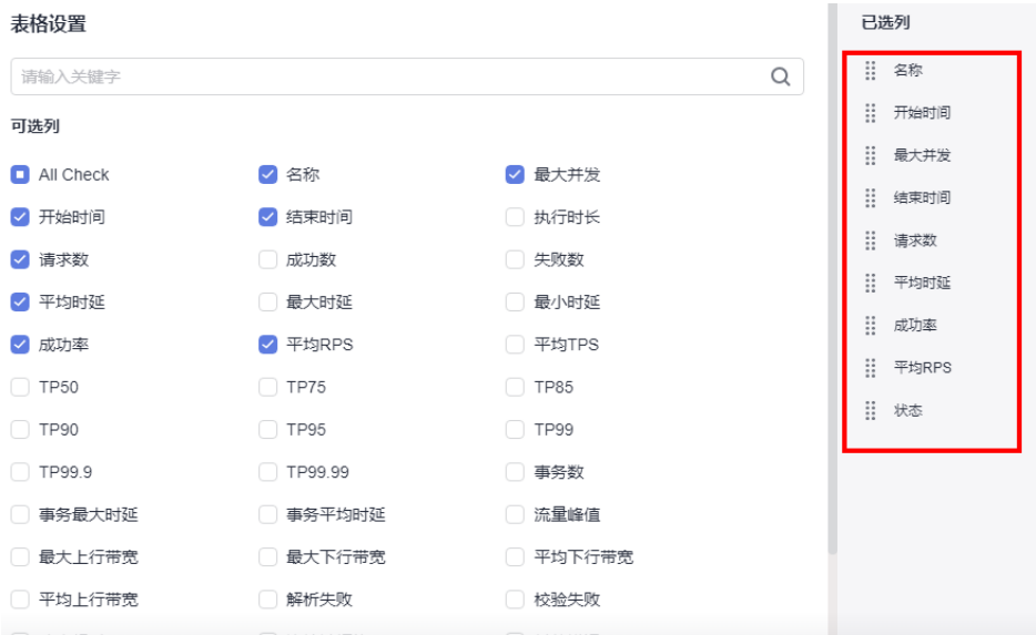
图 8-1 表格设置
