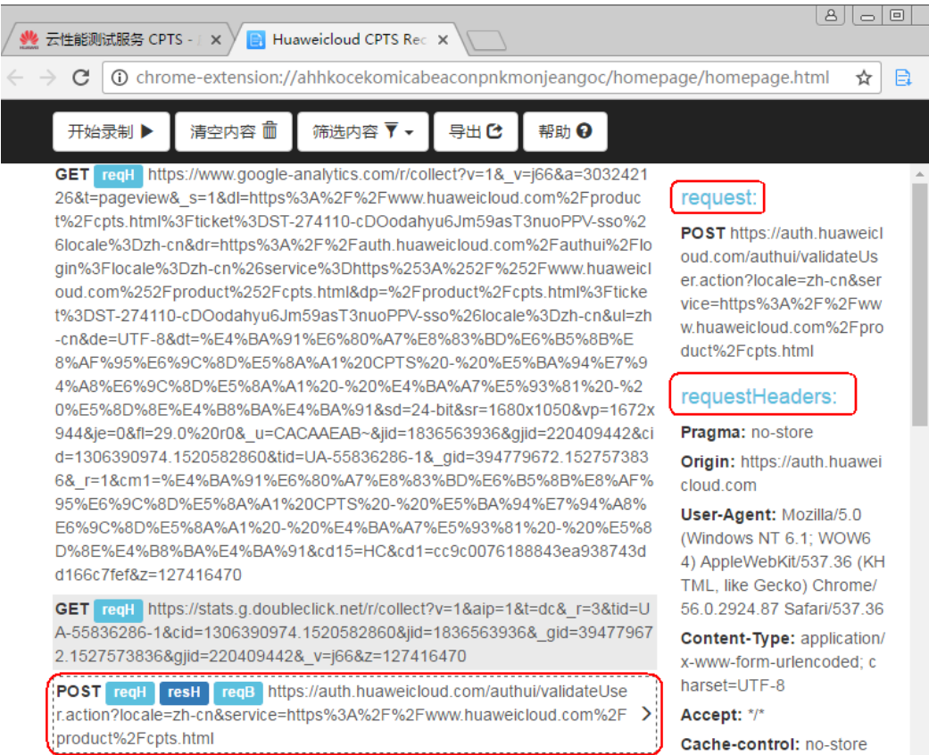
图 9-3 选择请求
