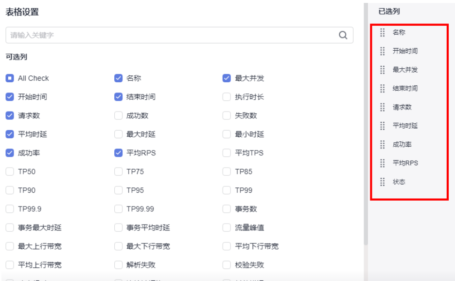
图 10-4 表格设置
