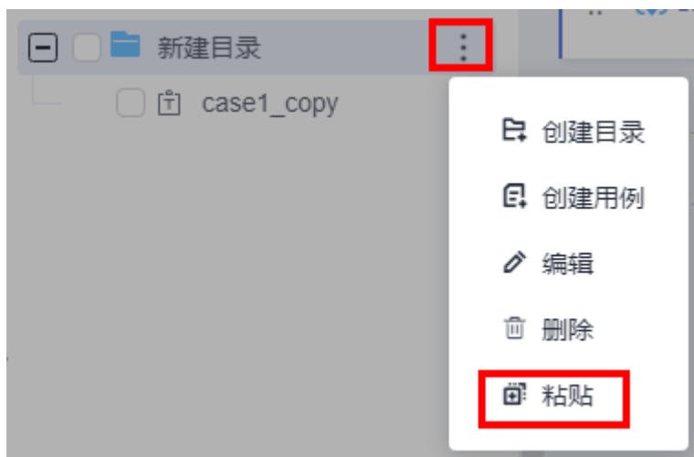
图 6-17 粘贴用例
