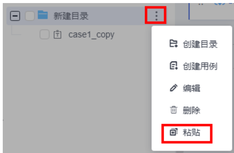
图 6-19 粘贴用例
