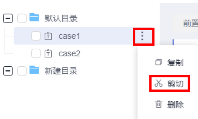
图 6-18 剪切用例
