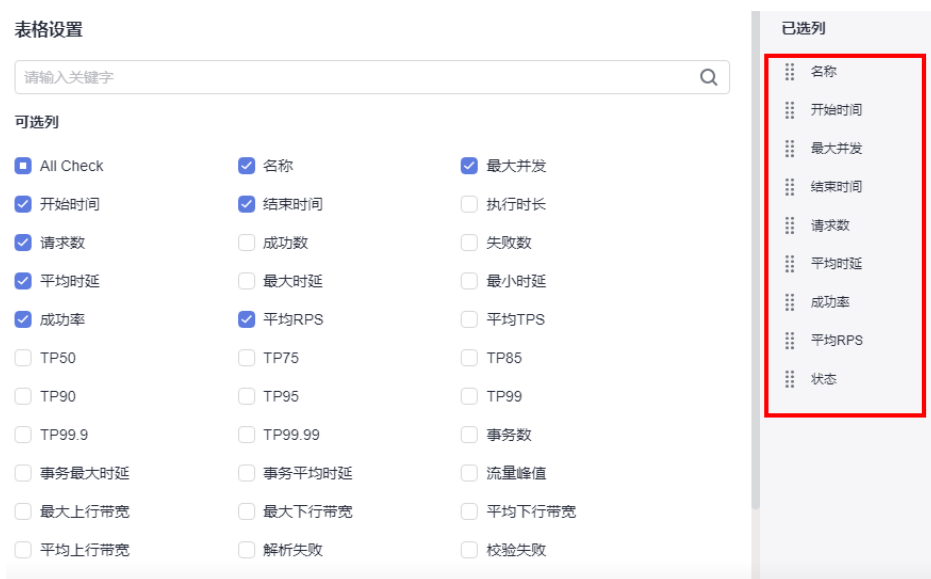
图 10-3 表格设置
