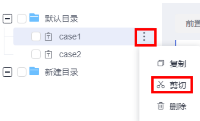
图 6-23 剪切用例
