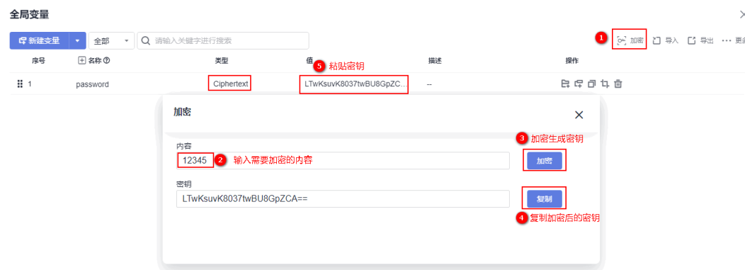
图 6-16 变量加密
