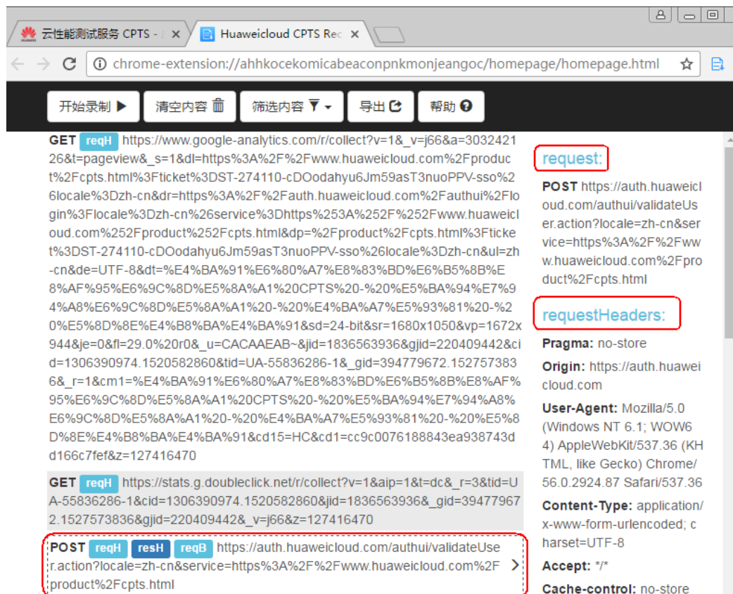
图 9-3 选择请求
