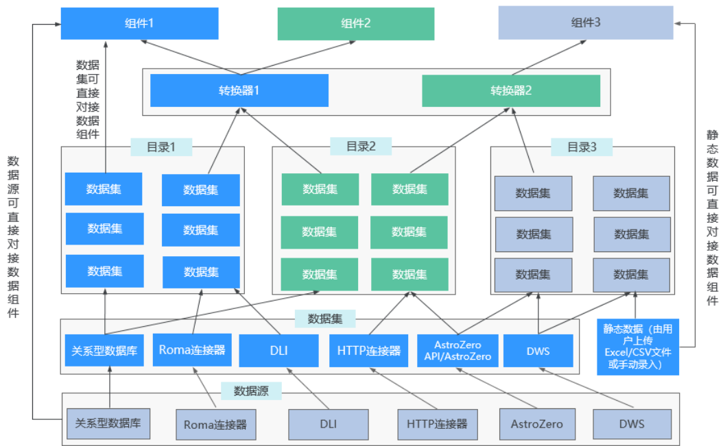
图 1-3 数据源、数据集、转换器、目录之间的关系图
