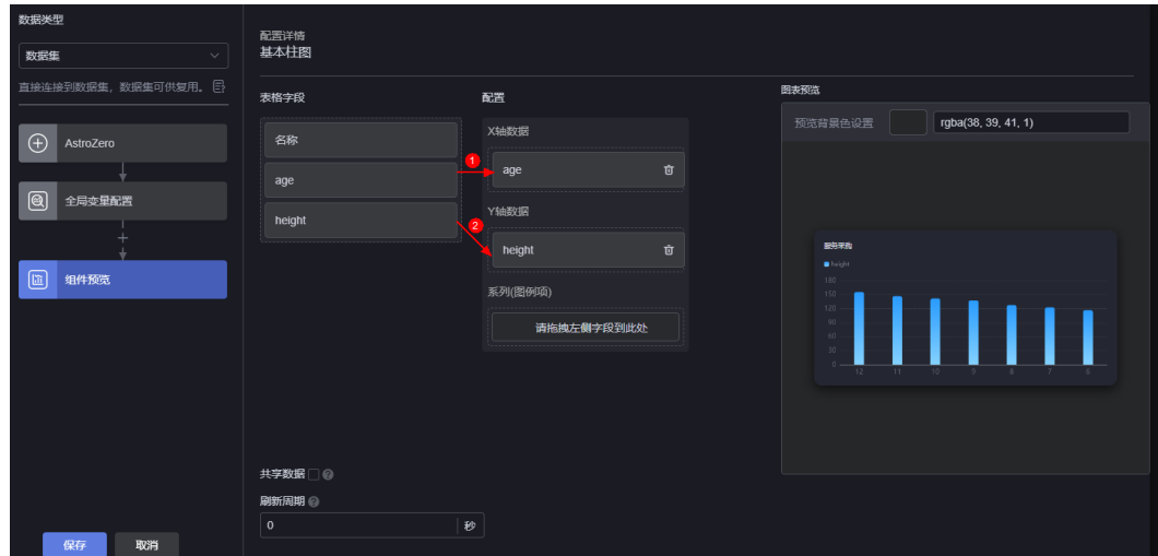
图 15-53 拖拽字段到坐标轴
