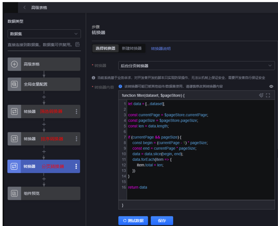
图 20-74 转换器添加顺序
