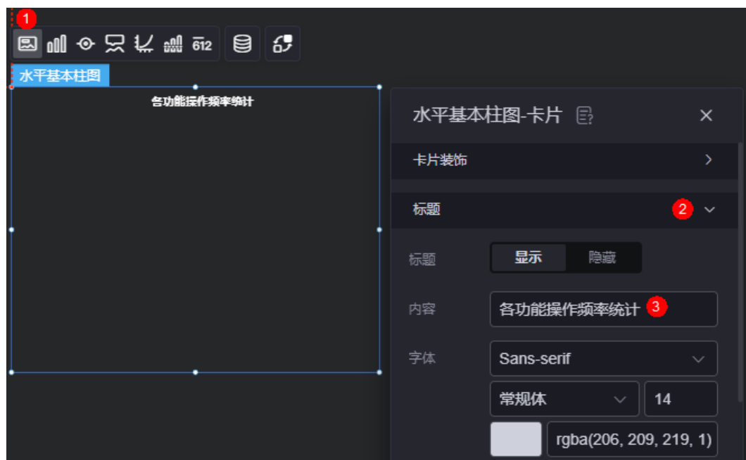
图 15-73 设置图表标题
