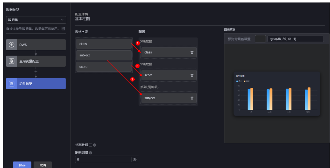
图 15-65 拖拽字段到坐标轴
