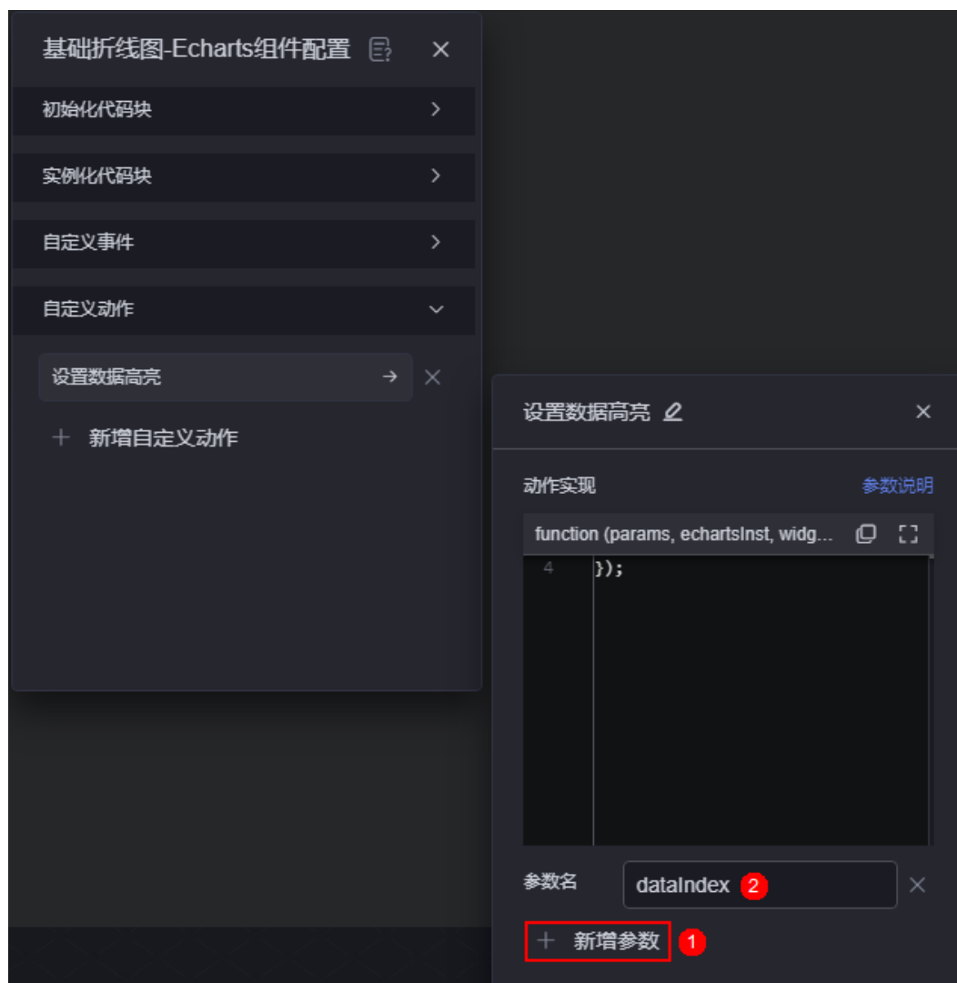
图 20-63 新增 dataIndex 字段
