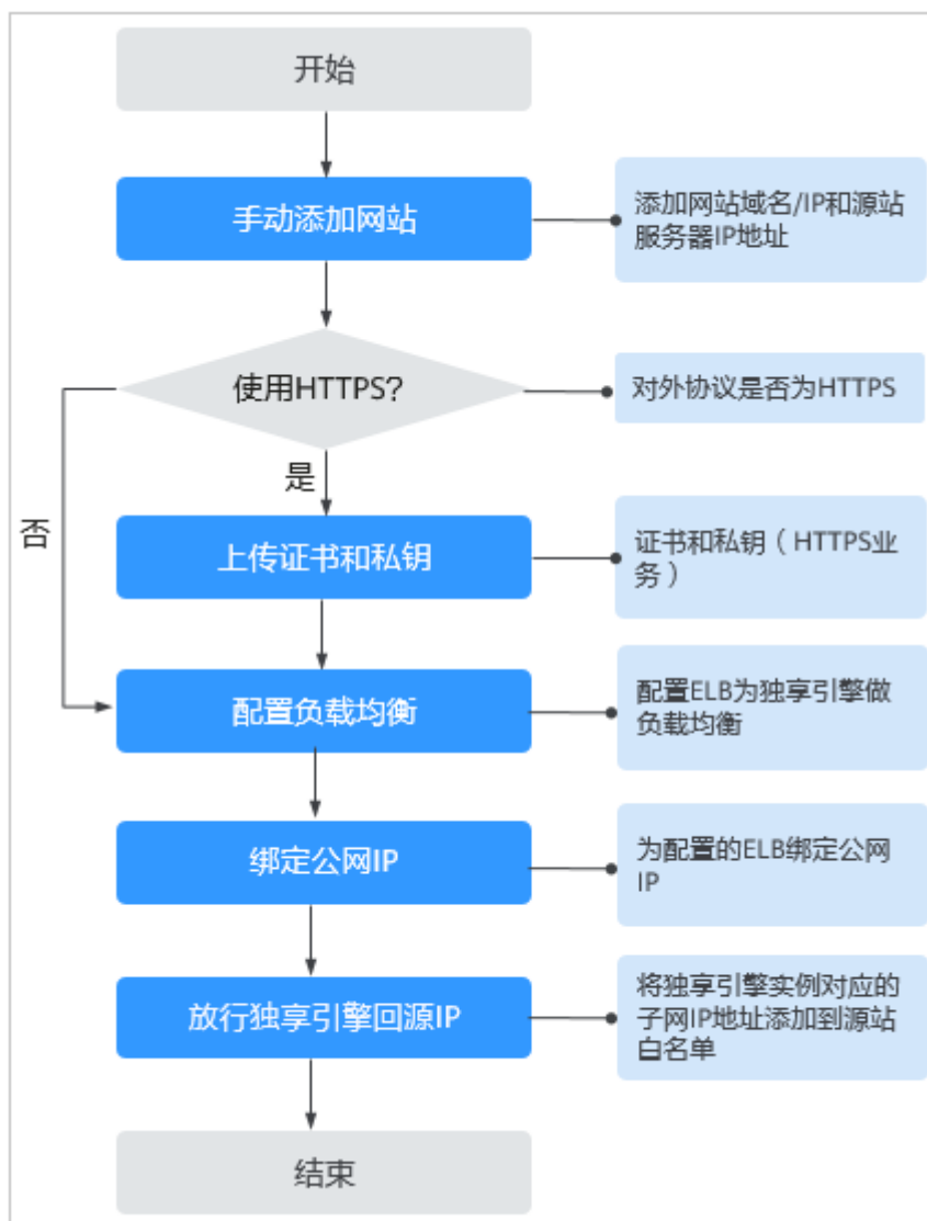
图 7-33 网站接入 WAF 的操作流程图-独享模式
