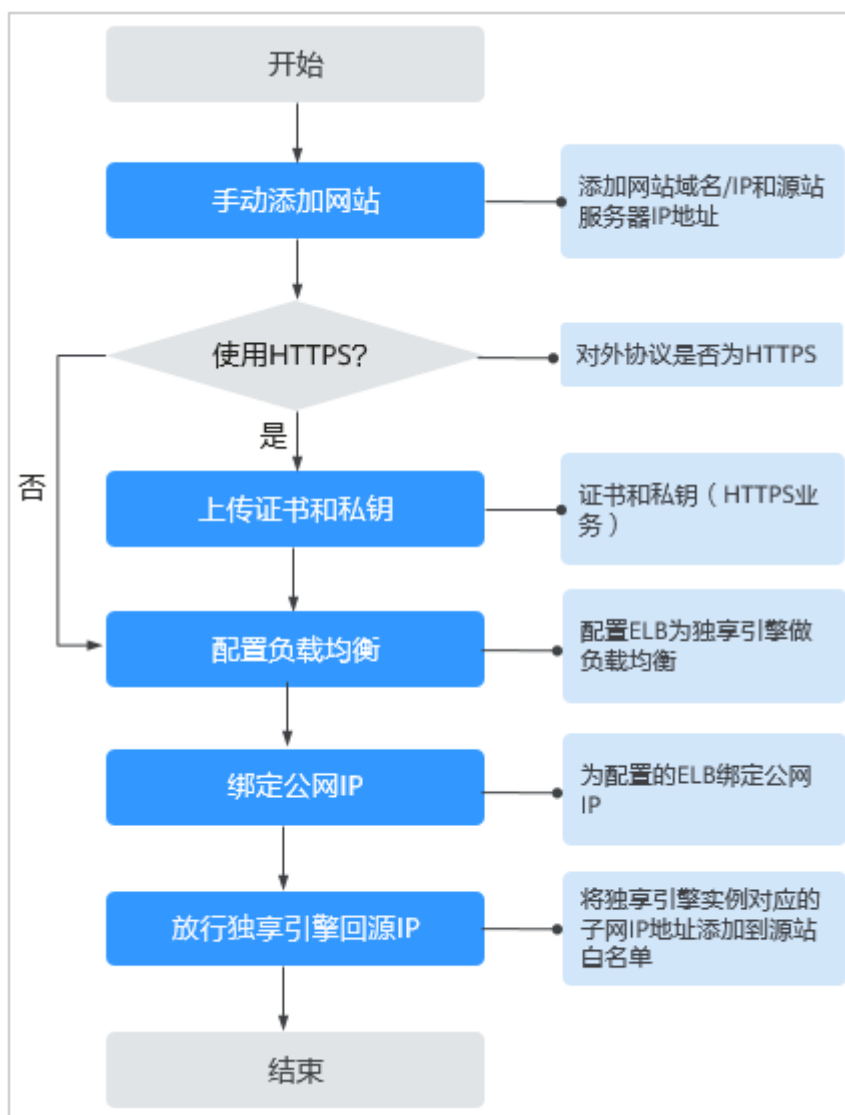
图 3-2 网站接入 WAF 的操作流程图-独享模式
