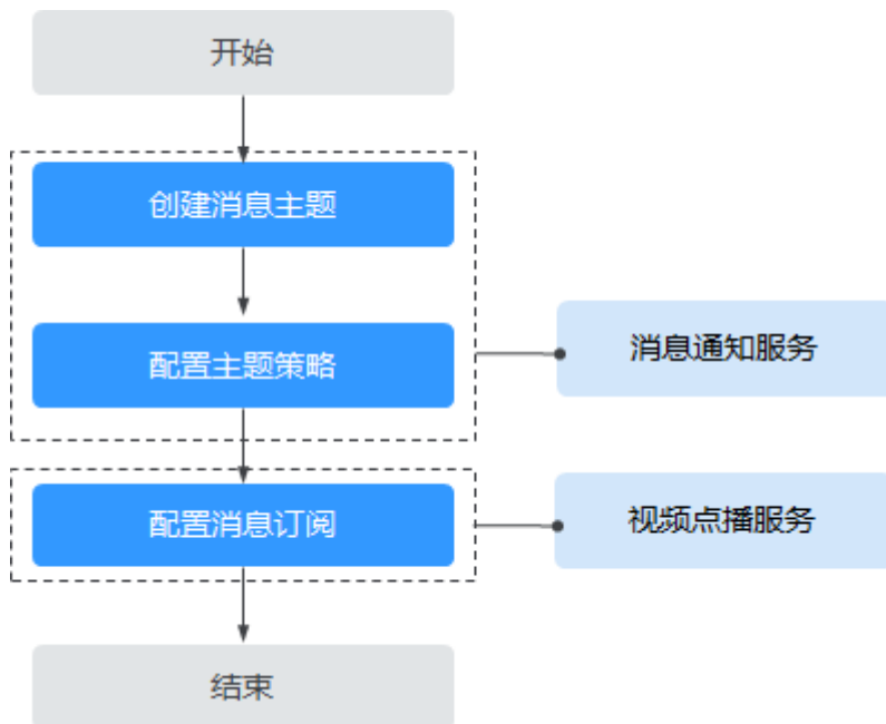
图 8-16 消息订阅配置流程图
