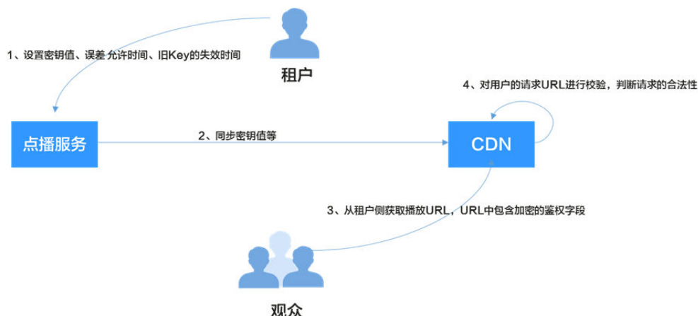
图 4-18 Key 防盗链实现原理
