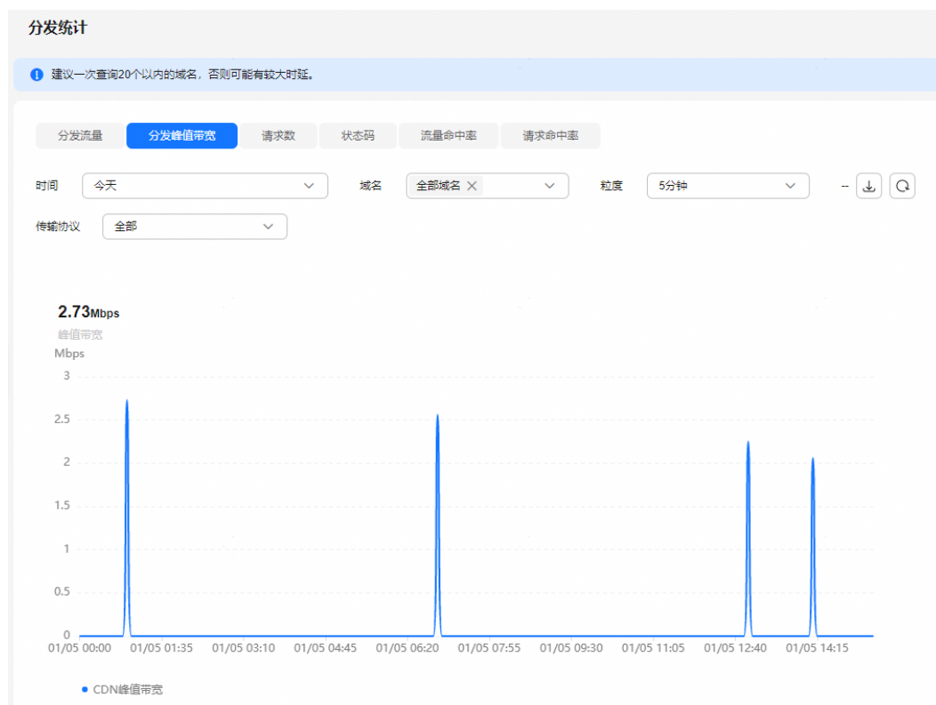
图 11-2 CDN 峰值带宽统计信息
