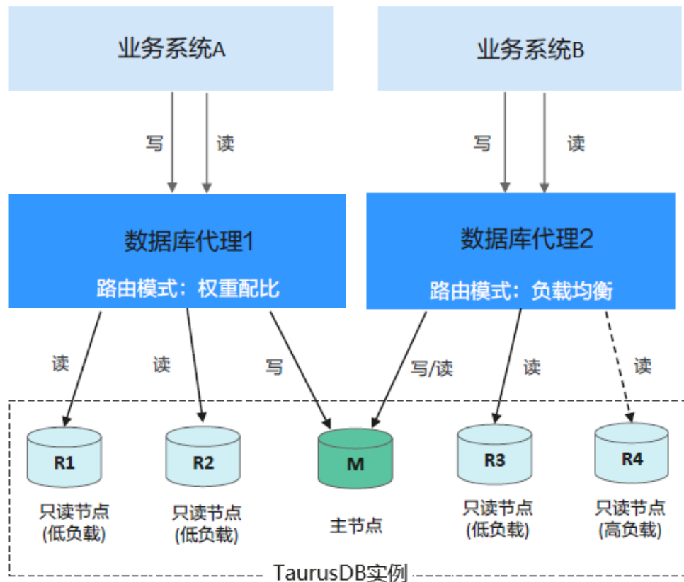
图 12-2 多个数据库代理读写分离
