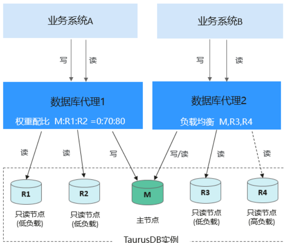
图 12-16 路由模式工作原理
