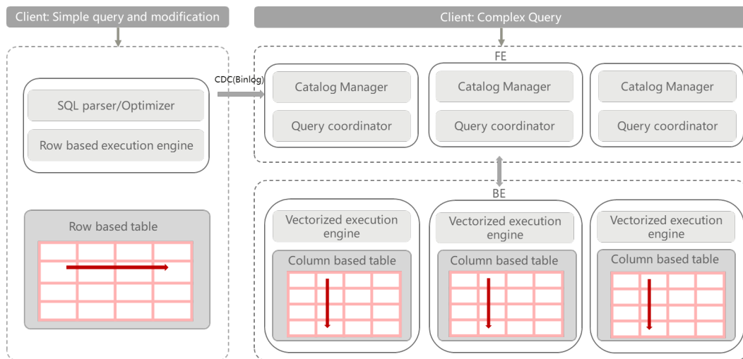
图 18-1 产品架构
