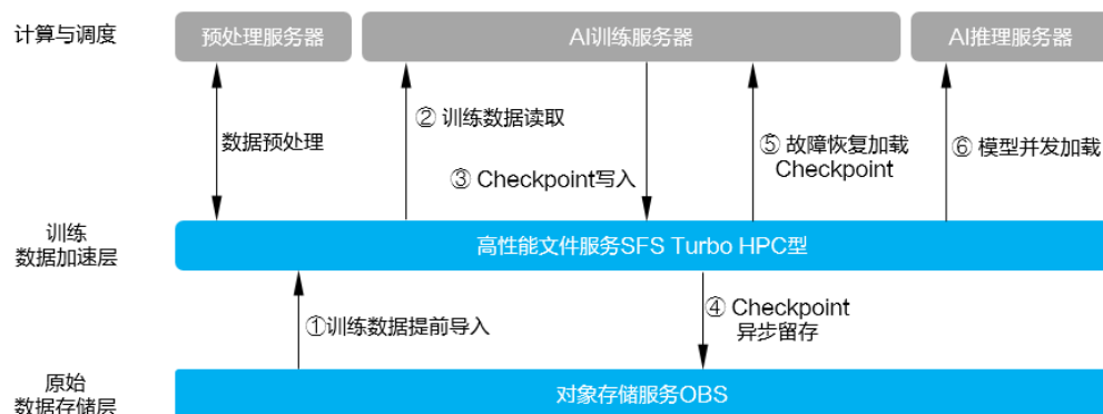
图 8-29 基于 OBS+SFS Turbo 的存储解决方案
