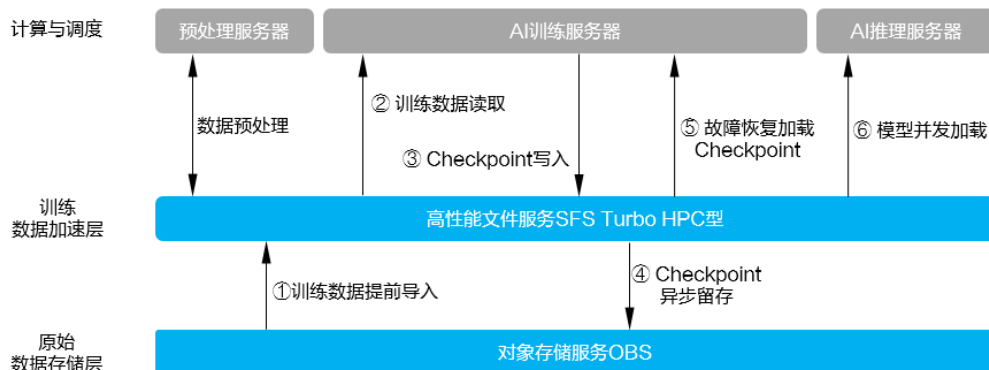
图 8-30 基于 OBS+SFS Turbo 的华为云 AI 云存储解决方案
