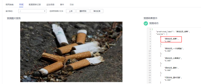
图 5-11 预测结果
