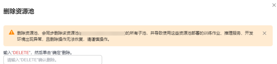
图 3-40 删除资源池
