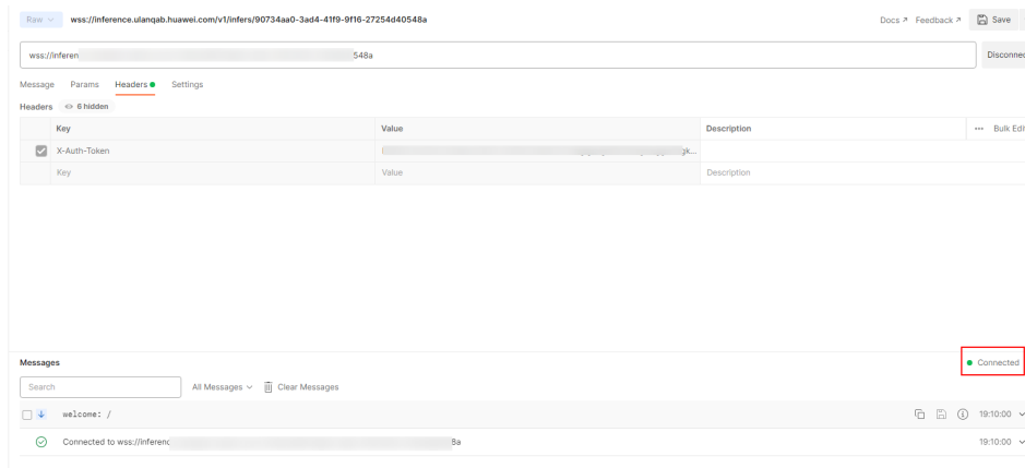
图 9-47 连接成功
