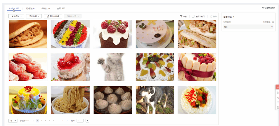
图 7-48 标注样例
