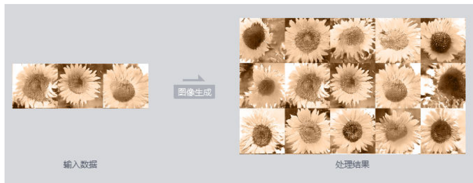
图 7-35 StyleGan 算子
