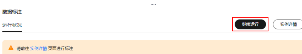
图 4-10 继续运行
