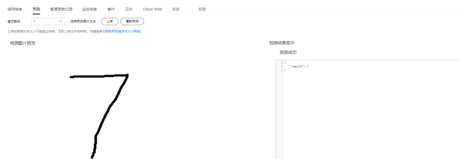
图 10-46 预测
