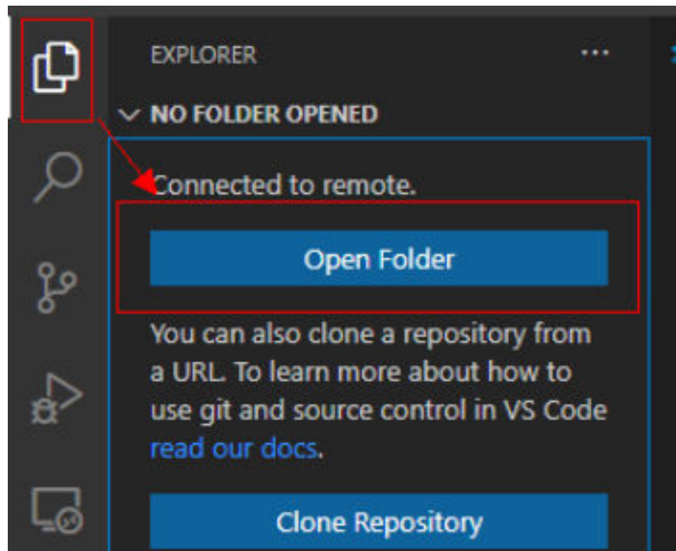
图 6-137 Open Folder
