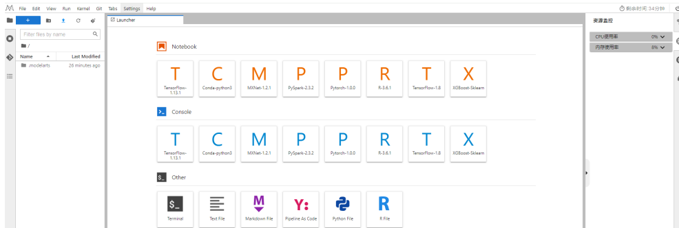
图 6-181 CodeLab 首页
