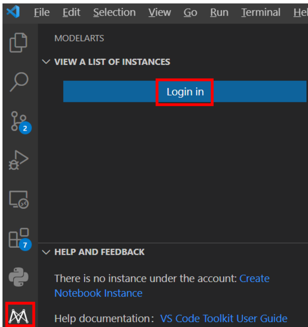
图 6-129 安装完成
