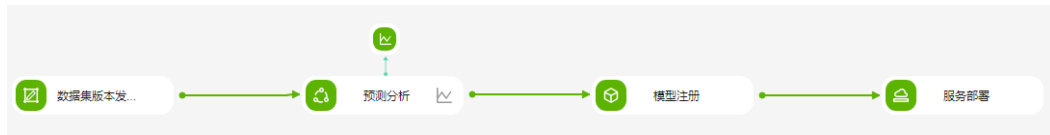
图 5-3 workflow
