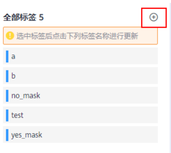
图 7-56 全部标签
