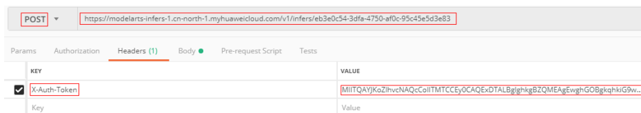
图 9-23 参数填写
