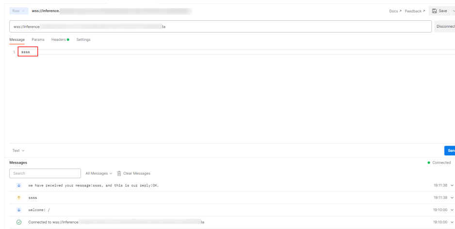
图 9-48 发送数据
