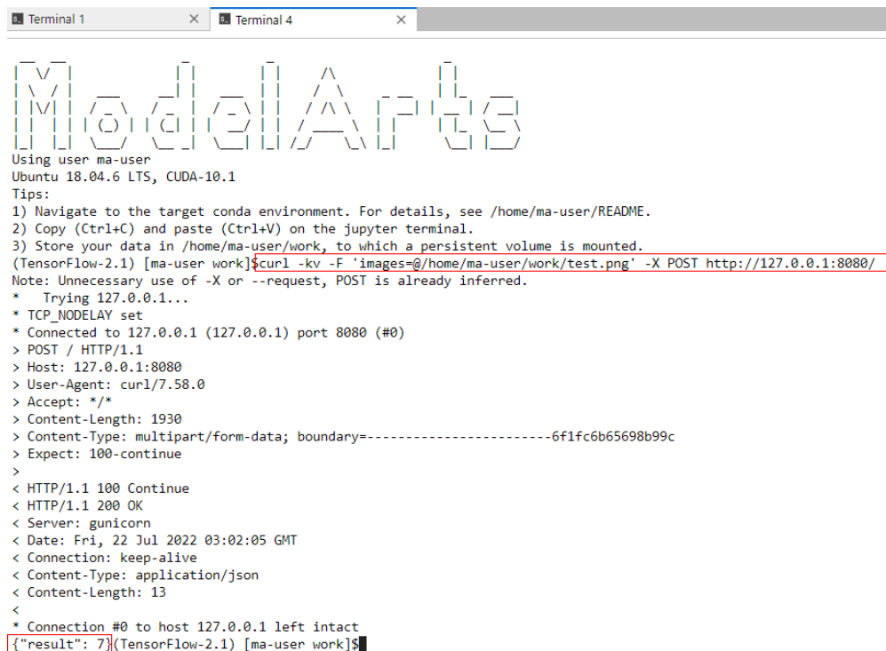
图 10-58 预测
