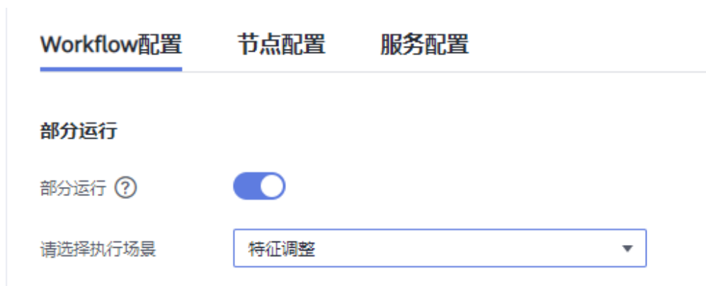
图 5-19 部分运行
