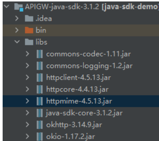
图 9-36 Java 依赖库
