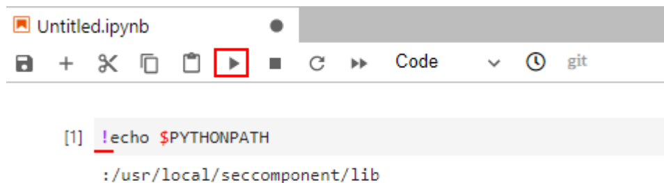
图 6-21 运行代码
