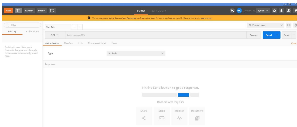
图 9-22 Postman 界面
