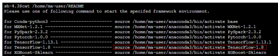
图 6-14 激活环境
