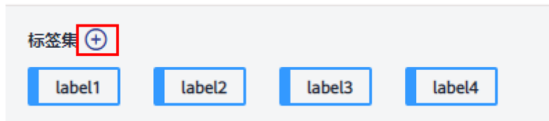
图 7-64 添加标签 (1)
