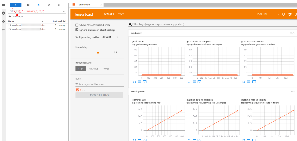
图 6-81 TensorBoard 界面 (1)
