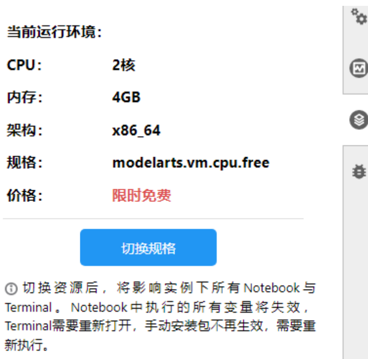
图 6-182 切换规格
