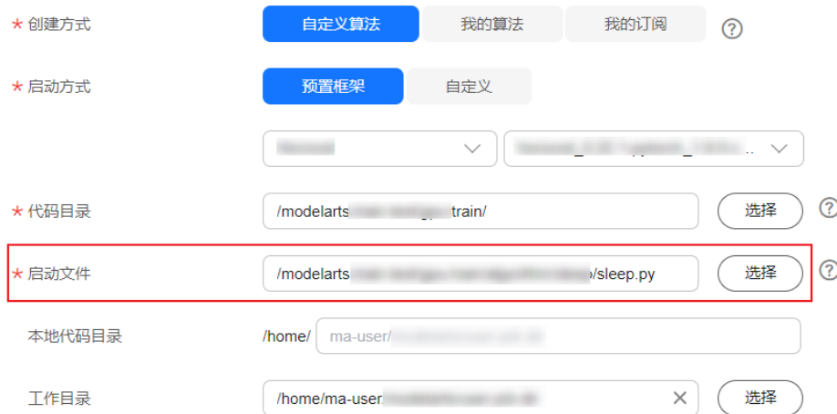
图 8-63 预置框架启动方式
