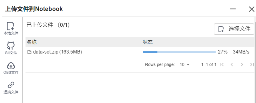
图 6-54 上传文件
