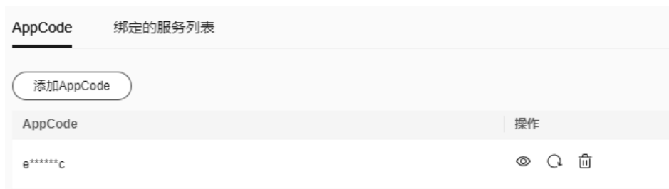
图 9-34 添加 AppCode
