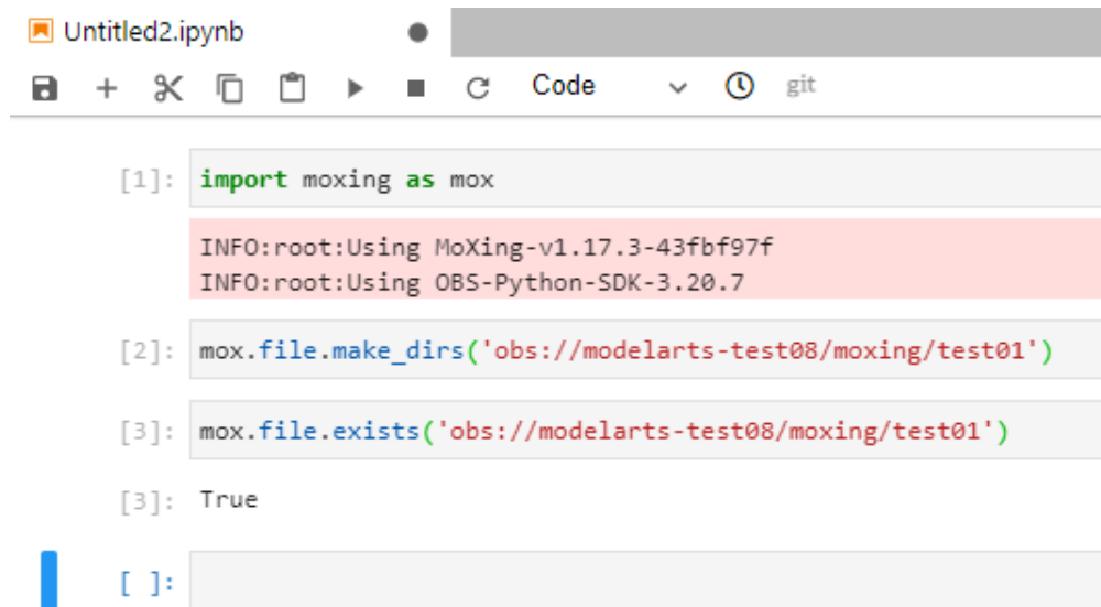
图 6-188 运行示例
