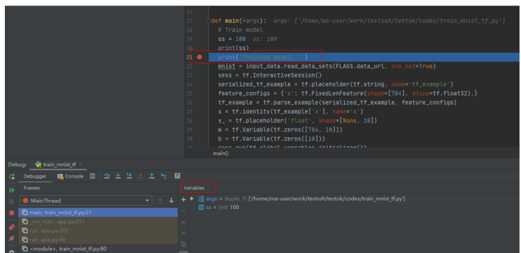
图 6-105 Debug 模式
