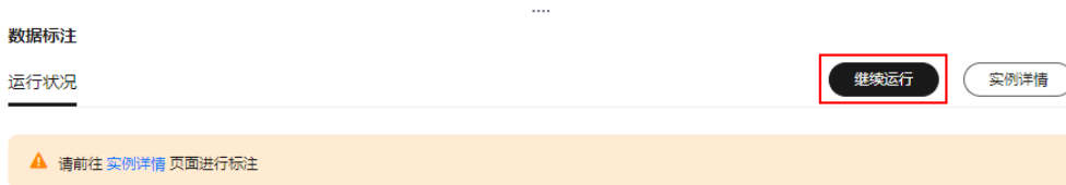
图 4-21 继续运行
