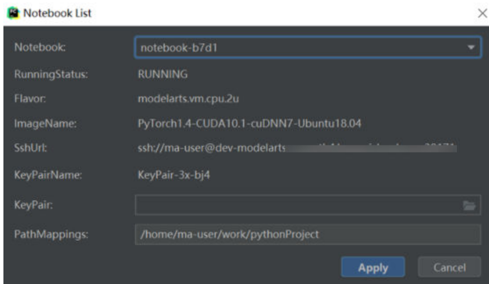
图 6-86 Notebook 列表
