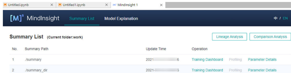
图 6-78 MindInsight 界面 ( 2 )
