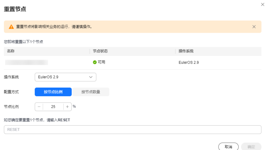
图 3-29 重置节点
