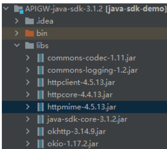
图 9-27 Java 依赖库
