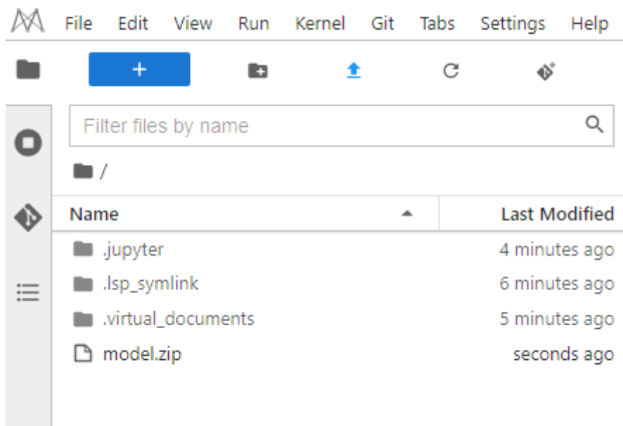
图 10-35 上传模型包
