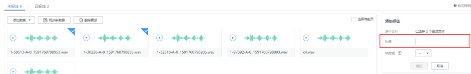
图 4-33 音频标注
