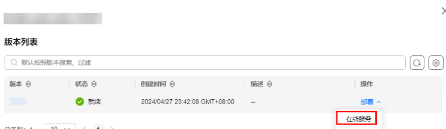
图 9-7 部署模型
