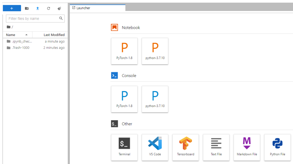
图 6-9 JupyterLab 主页
