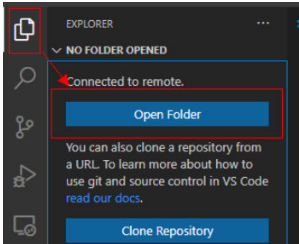
图 6-123 Open Folder
