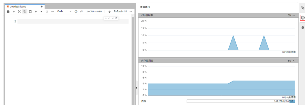
图 6-33 资源监控
