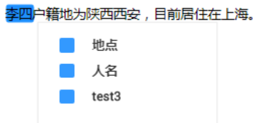
图 7-71 实体标注
