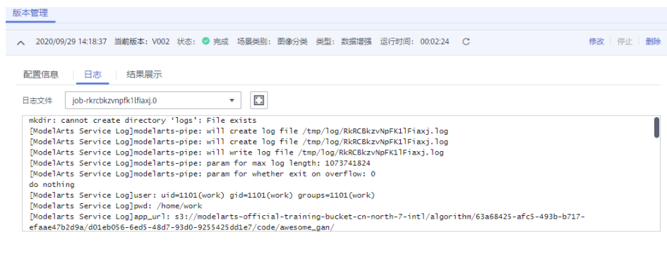
图 7-38 日志页面
