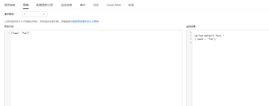
图 9-11 服务预测
