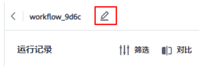
图 5-13 编辑 Workflow
