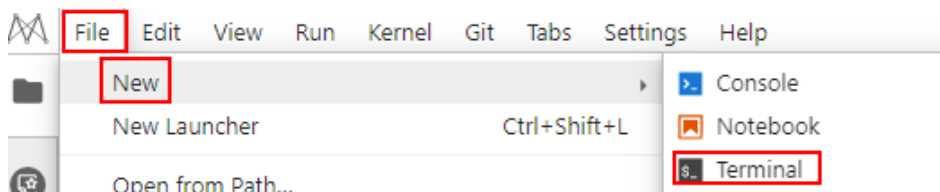
图 6-56 打开 Terminal
