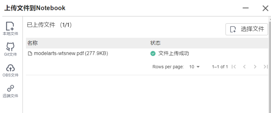
图 6-47 上传成功
