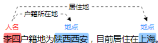
图 7-72 关系标注
