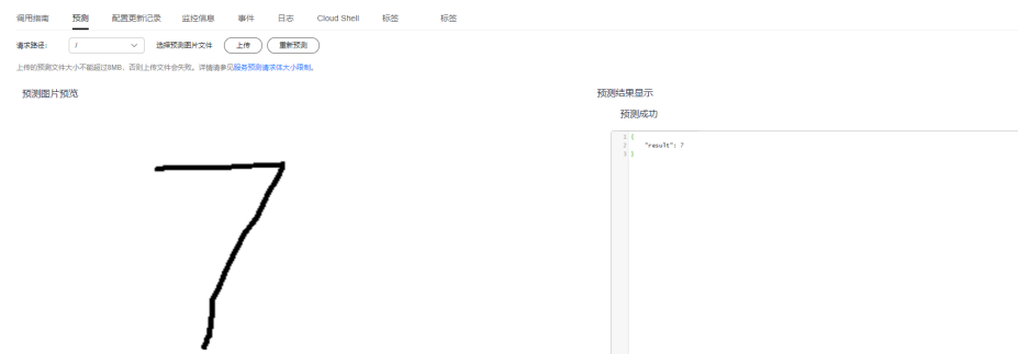
图 10-62 预测
