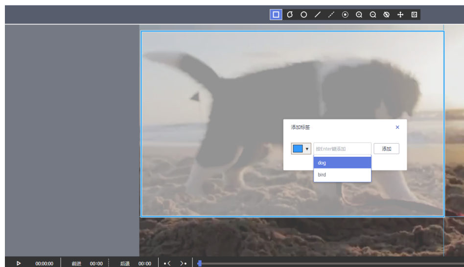
图 7-80 视频标注
