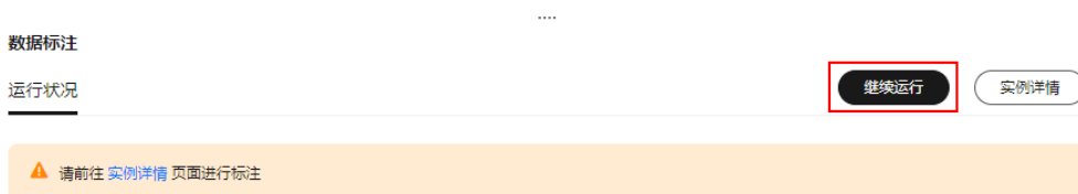
图 4-34 继续运行
