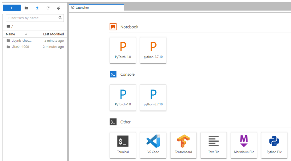
图 6-12 JupyterLab 主页
