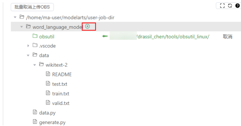
图 8-21 新建文件夹
