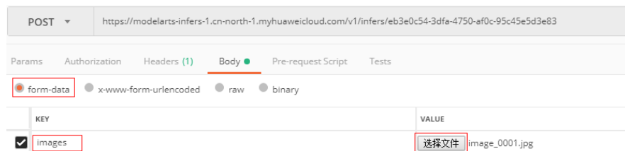
图 9-24 填写 Body
