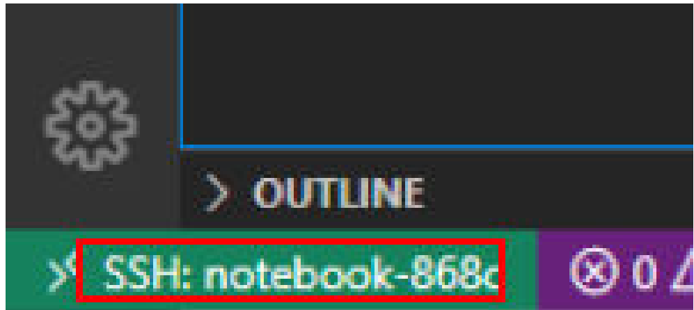
图 6-136 连接成功
