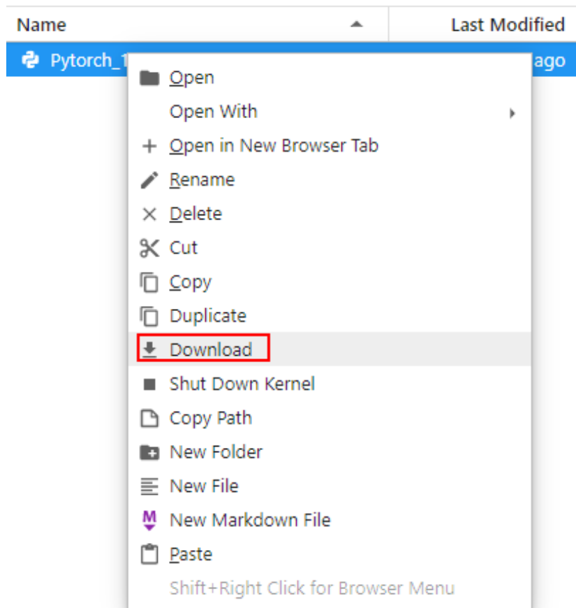
图 6-76 下载文件
