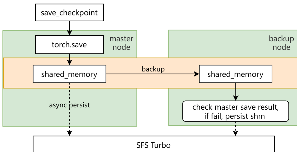
图 9-1 保存 checkpoint 流程
