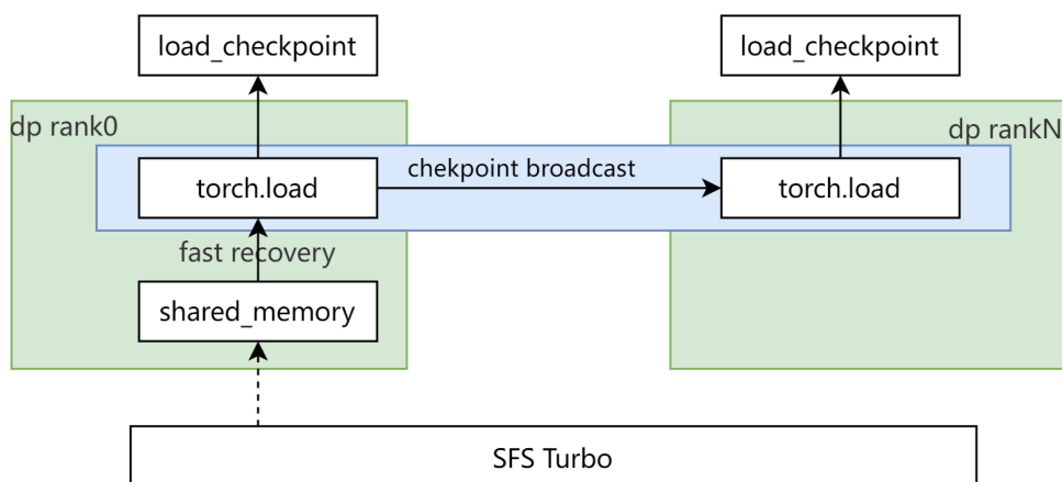
图 9-2 加载 checkpoint 流程
