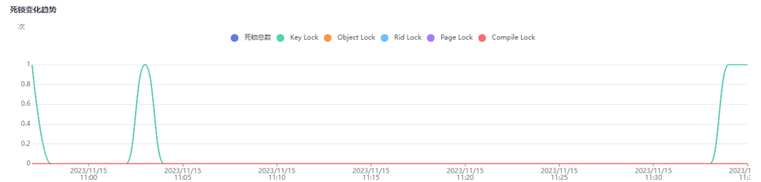
图 4-136 锁阻塞趋势
