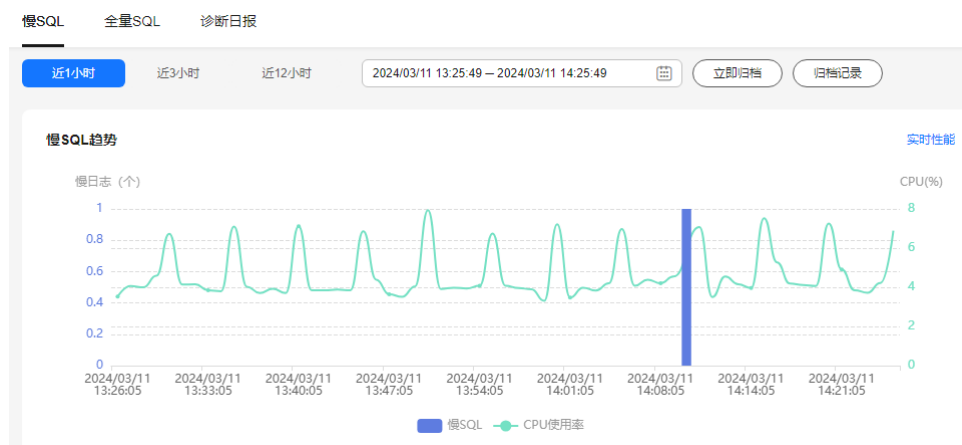
图 2-77 慢 SQL 趋势
