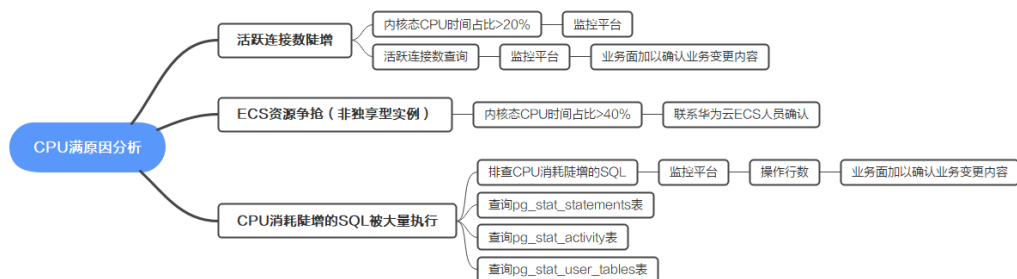
图 3-36 排查思路
