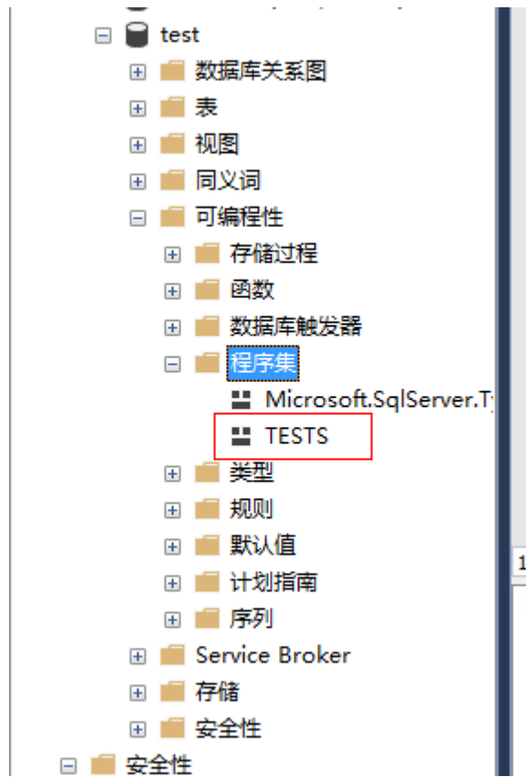
图 4-164 TESTS 程序集
