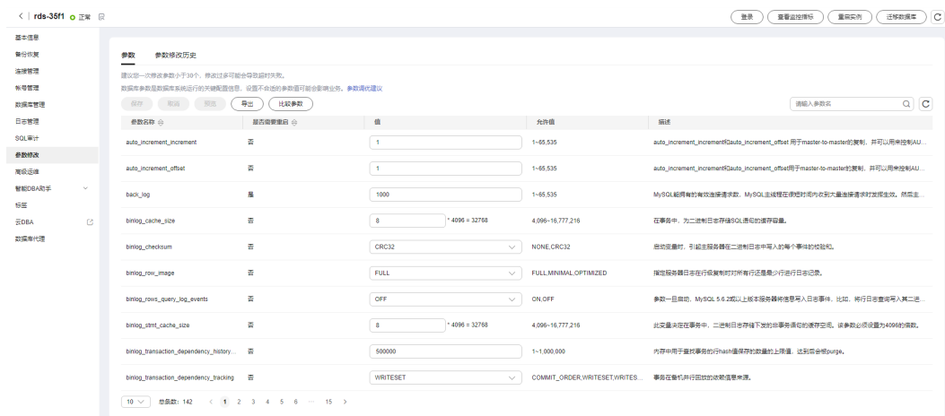
图 1-210 参数修改
