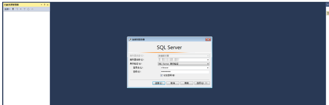
图 4-160 连接数据库
