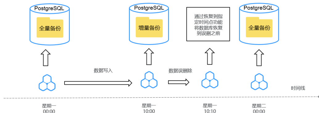
图 3-71 备份原理
