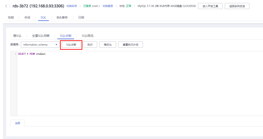
图 1-195 SQL 诊断
