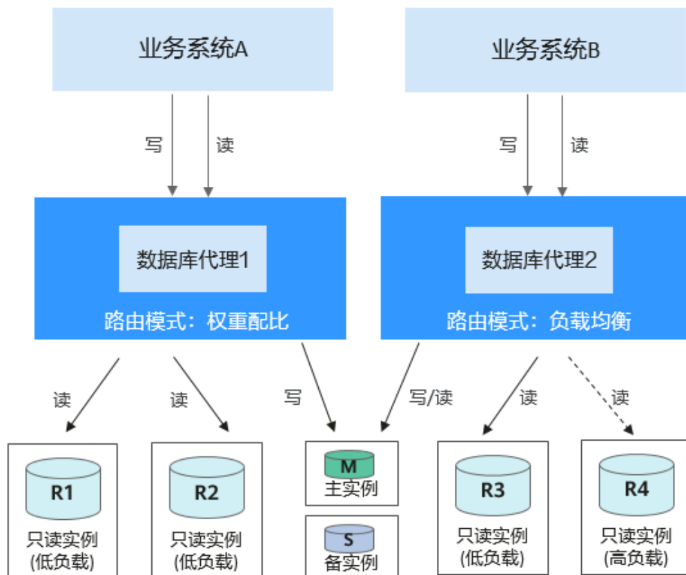
图 1-126 多个数据库代理原理图
