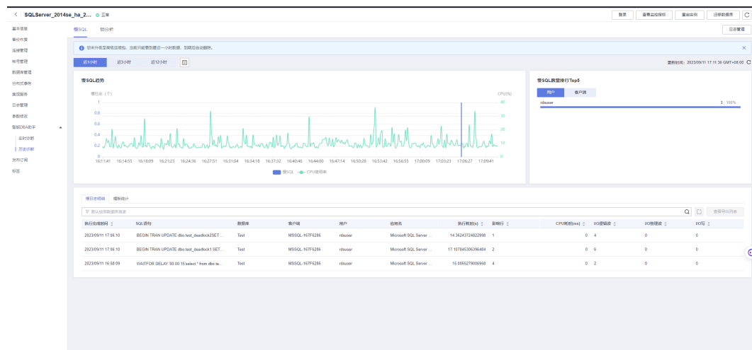
图 4-111 慢 SQL
