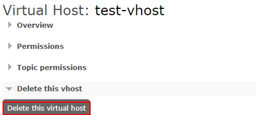
图 4-10 删除 Vhost
