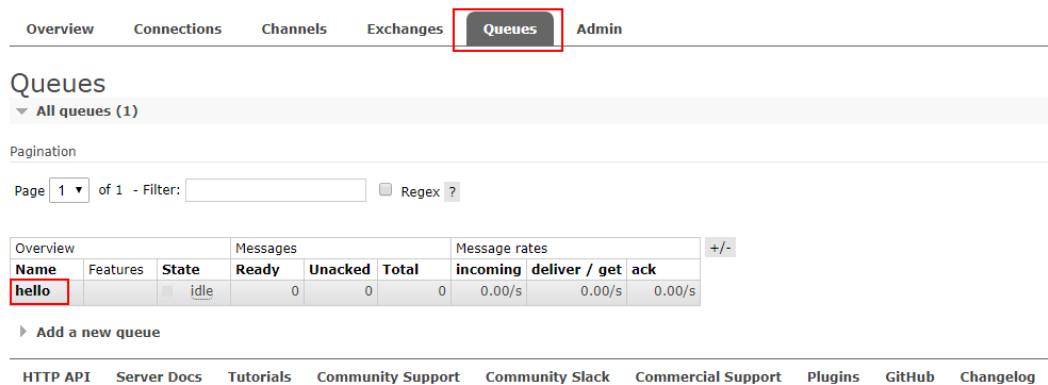
图 4-28 队列列表
