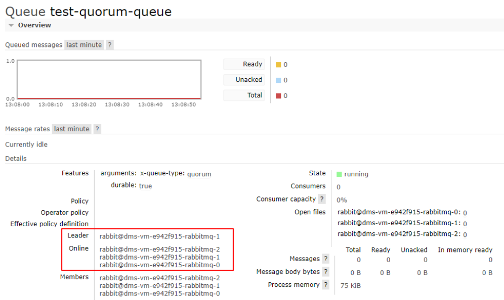
图 4-22 队列详情页
