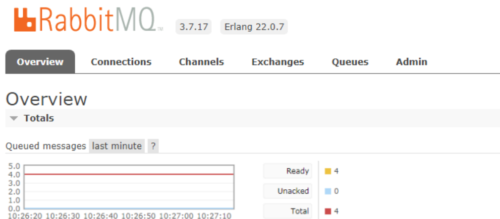
图 10-7 RabbitMQ WebUI
