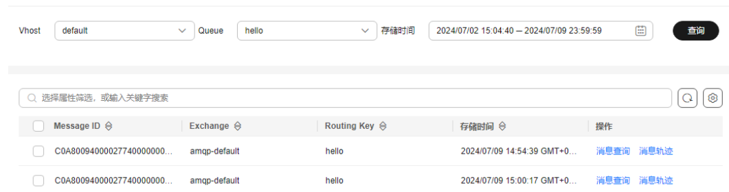
图 6-1 查询消息
