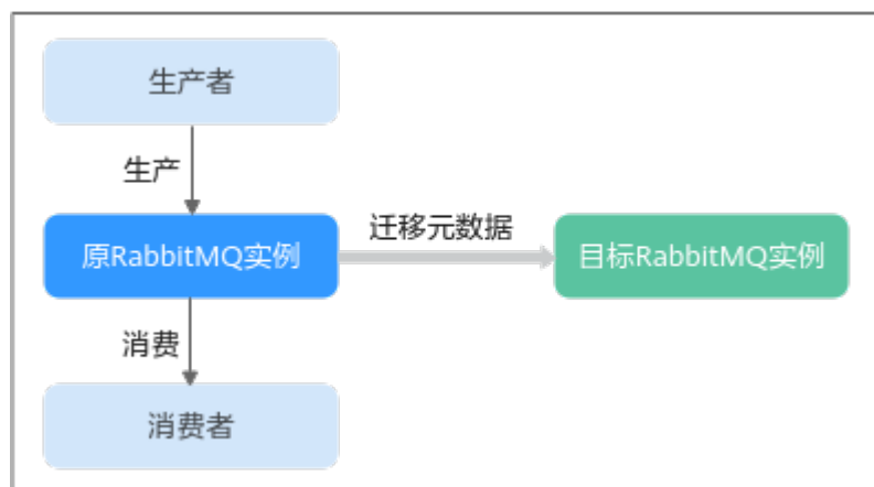
图 10-1 迁移元数据
