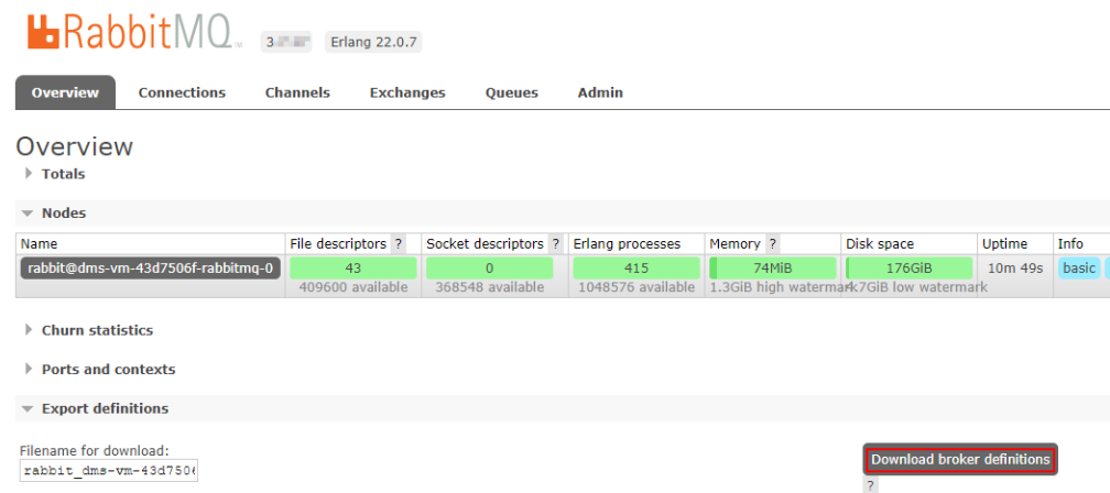
图 10-2 导出元数据
