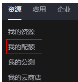
图 12-1 我的配额
