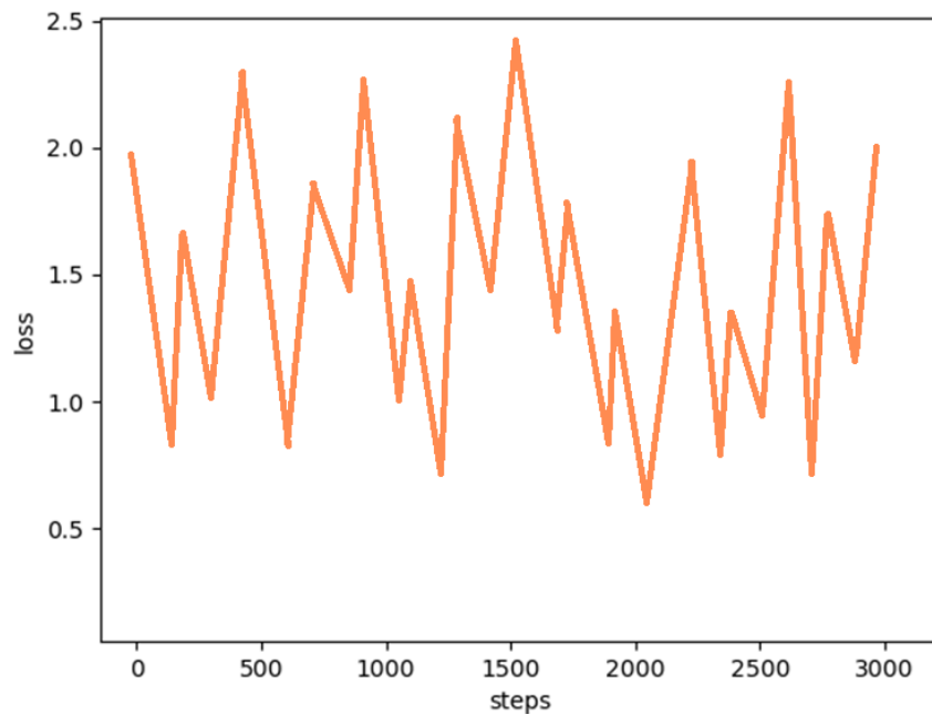
图 5-13 异常的 Loss 曲线：异常抖动
