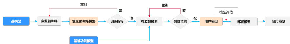
图 5-1 NLP 大模型训练方式与流程
