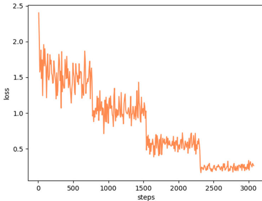
图 5-10 正常的 Loss 曲线：阶梯下降
