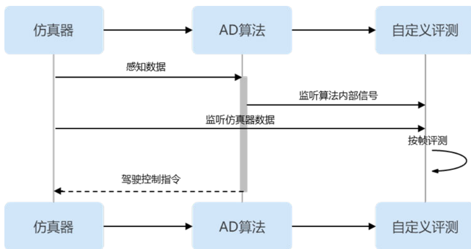
图 9-4 实时评测
