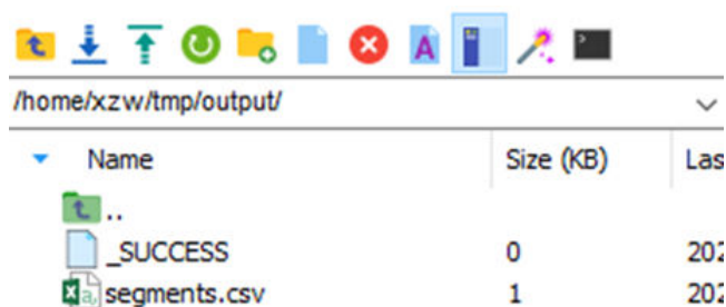
图 4-13 运行结果
