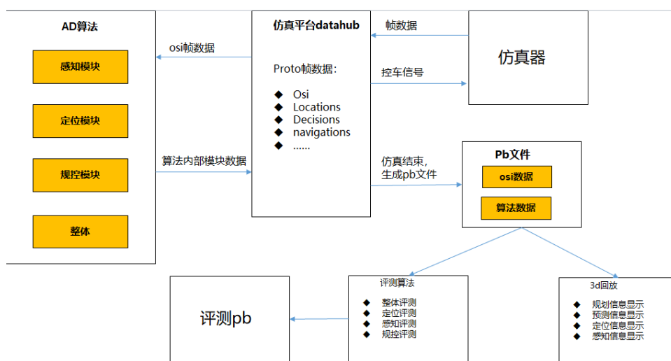
图 9-5 算法镜像
