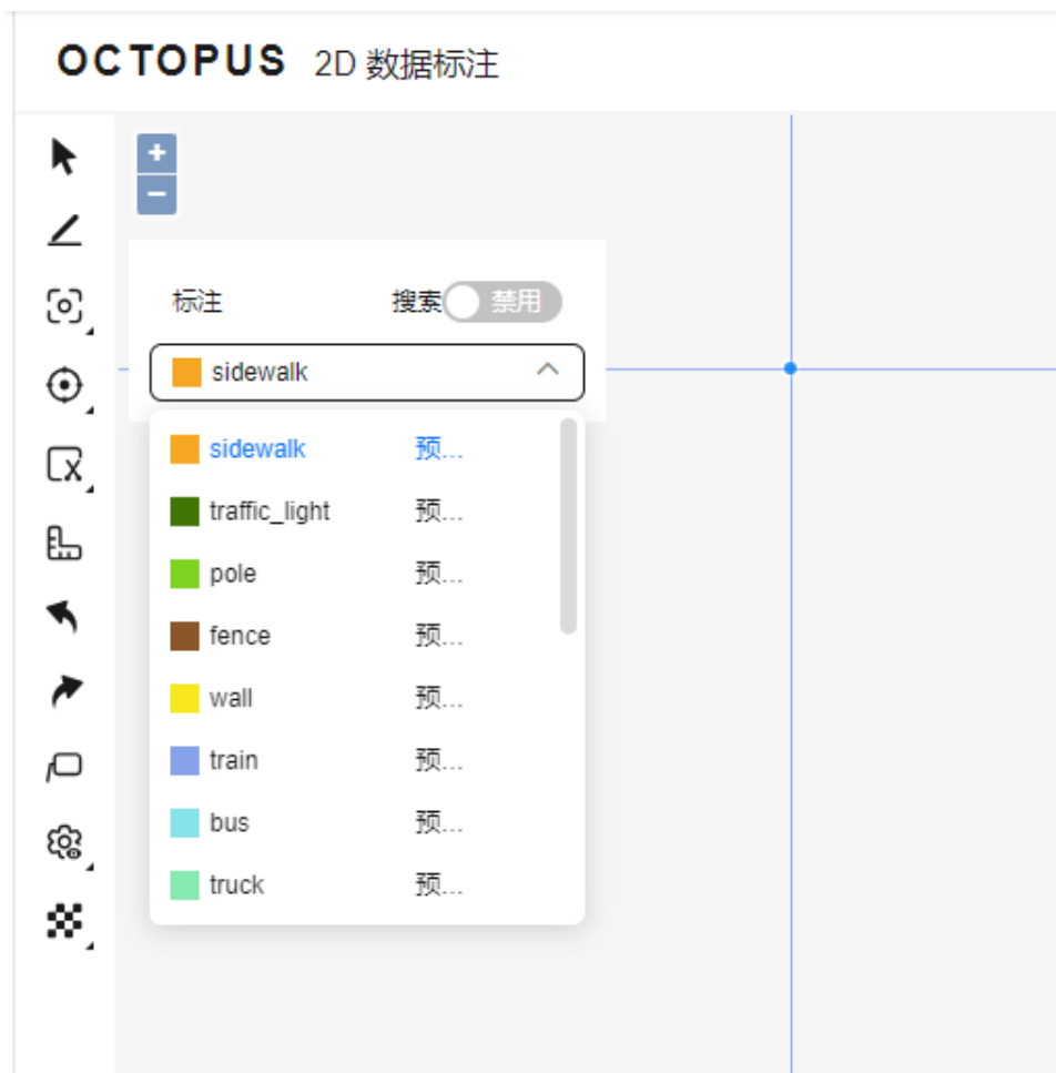
图 5-102 选择标注
