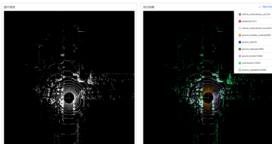
图 8-7 标注结果
