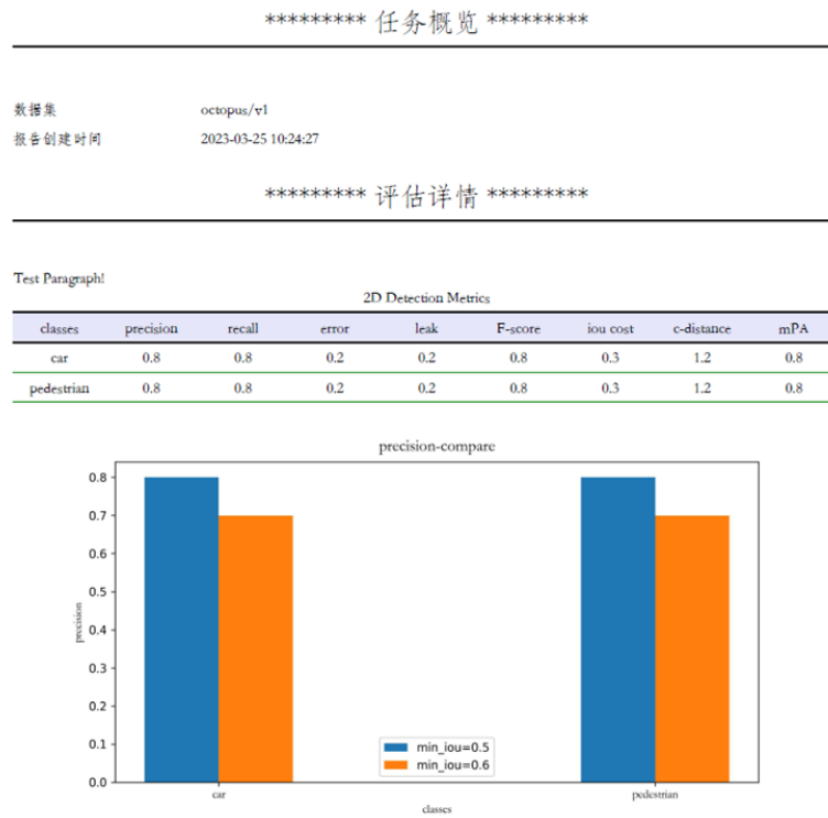
图 6-3 中文 pdf
