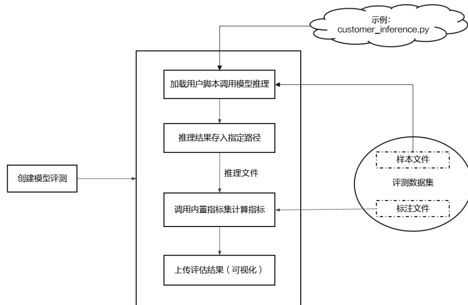
图 2-8 使用流程
