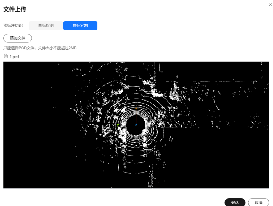
图 8-28 文件上传
