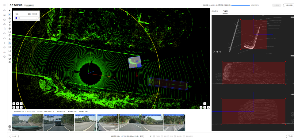
图 5-82 框选标注物
