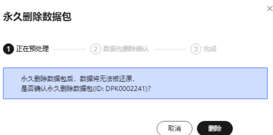
图 2-24 永久删除
