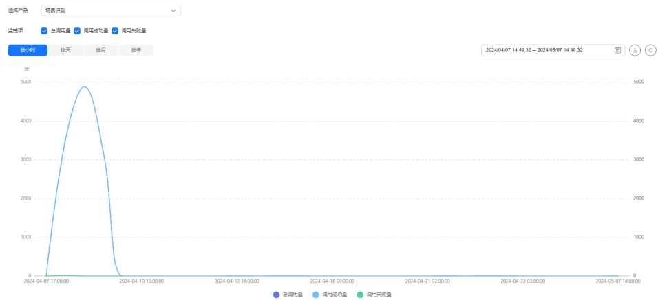
图 8-15 服务监控
