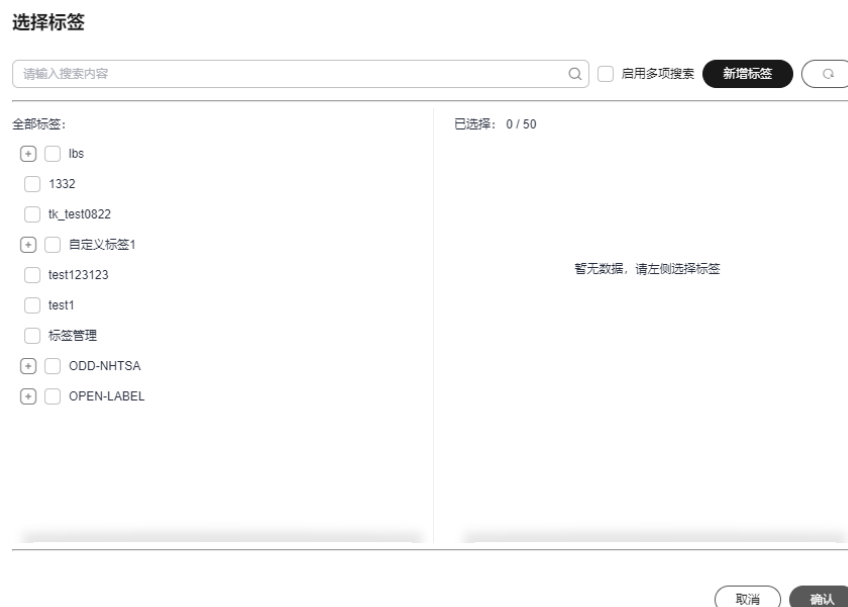
图 7-38 选择标签
