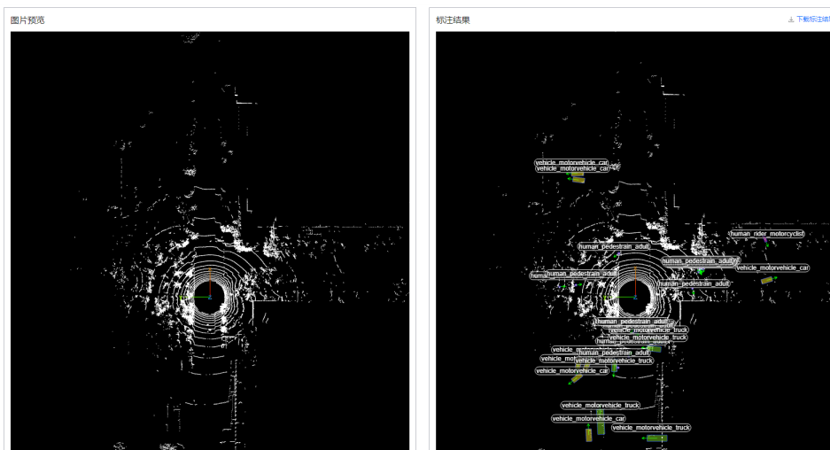
图 8-6 标注结果
