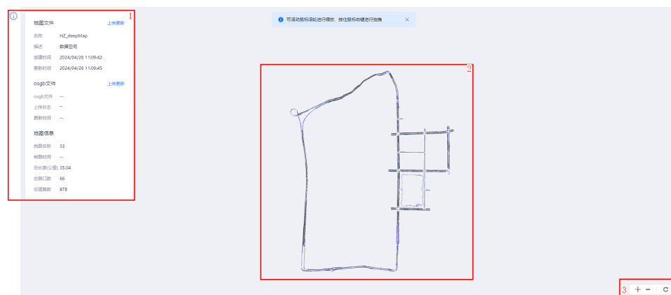
图 2-3 地图包详情
