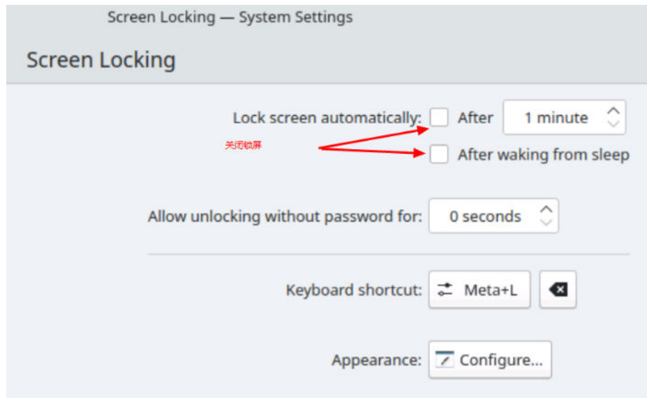
图 7-4 关闭锁屏
