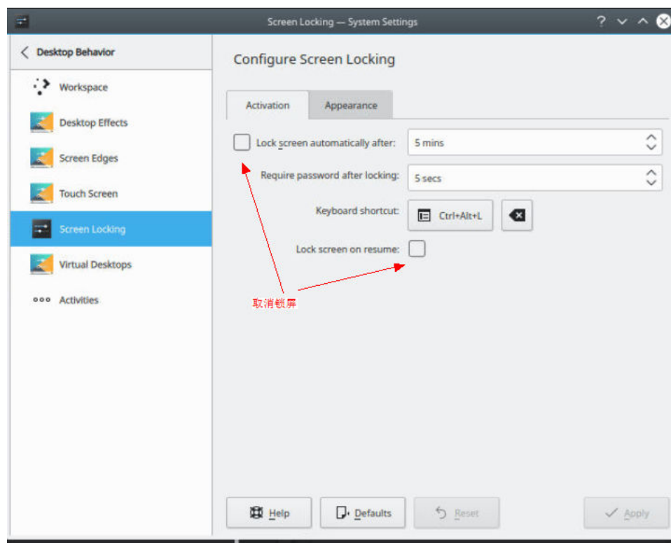
图 7-11 关闭锁屏
