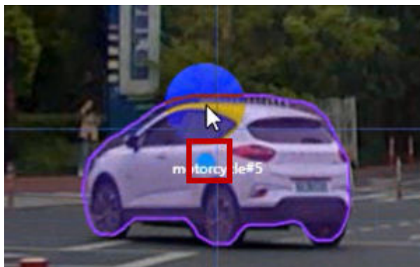
图 5-9 单击正点
