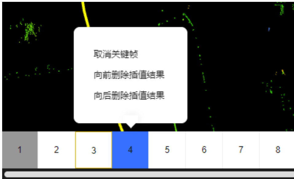
图 5-8 取消关键帧
