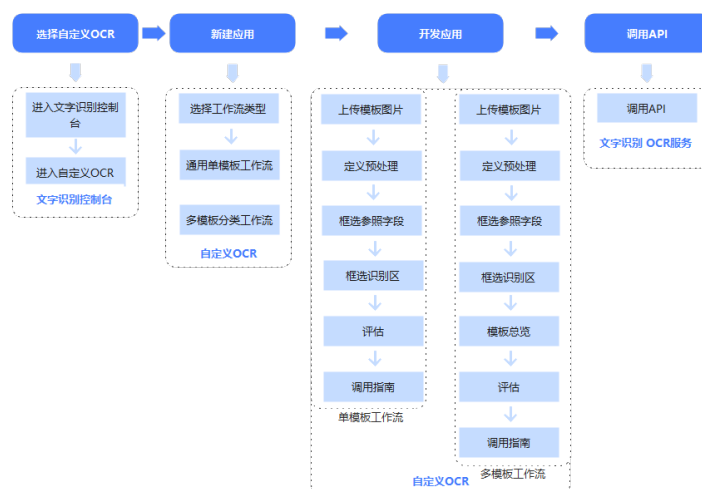
图 5-1 使用预置 workflow 开发应用
