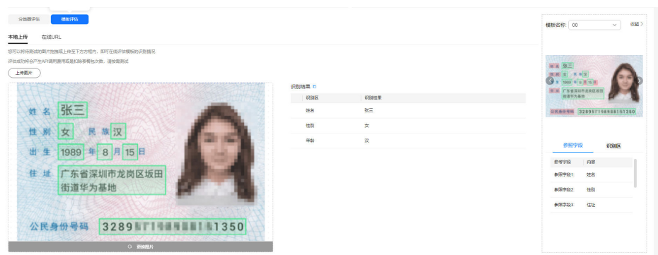
图 5-30 评估模板
