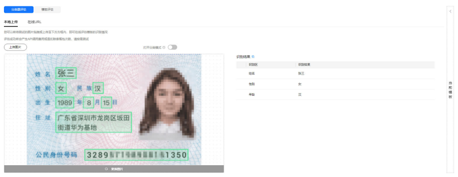
图 5-29 评估分类器
