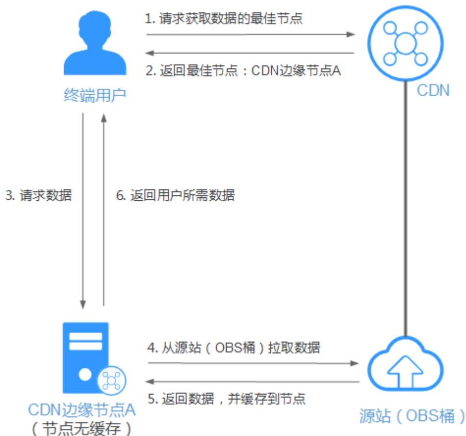
图 7-7 CDN 加速访问 OBS 示意图（CDN 节点无缓存）
