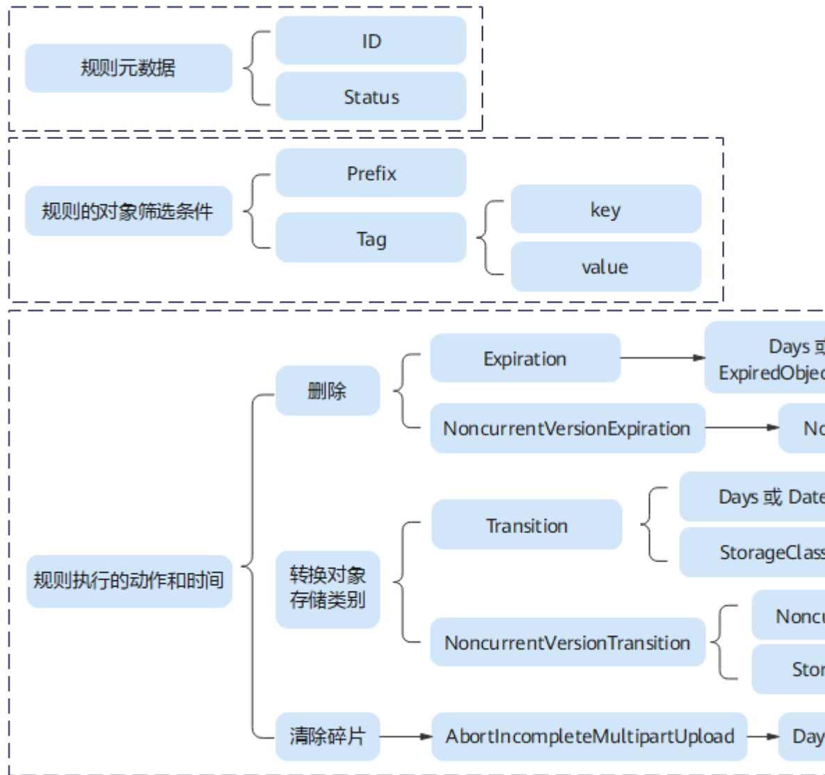
图 8-6 生命周期规则的组成元素
