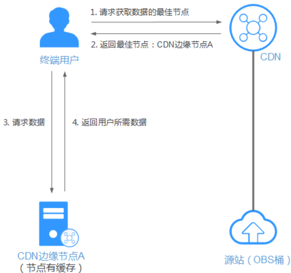
图 7-8 CDN 加速访问 OBS 示意图 (CDN 节点有缓存)
