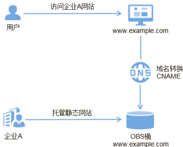
图 8-18 静态网站示意图
