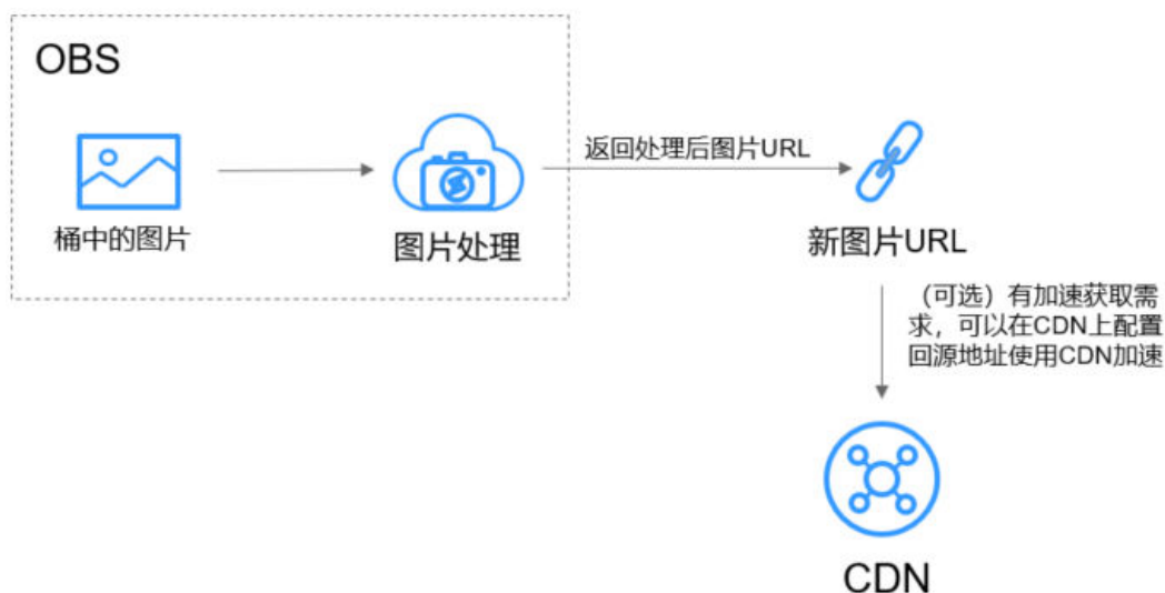
图 9-1 图片处理架构
