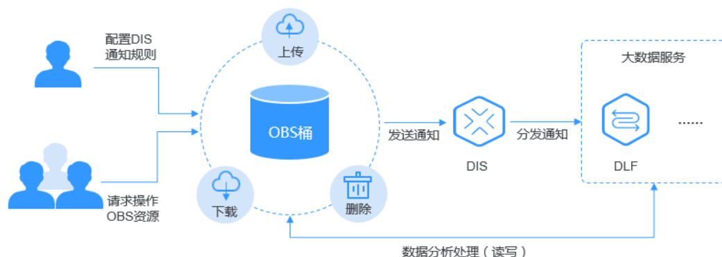
图 8-10 DIS 通知示意图
