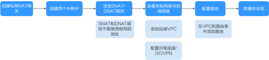
图 2-4 私网 NAT 网关使用流程
