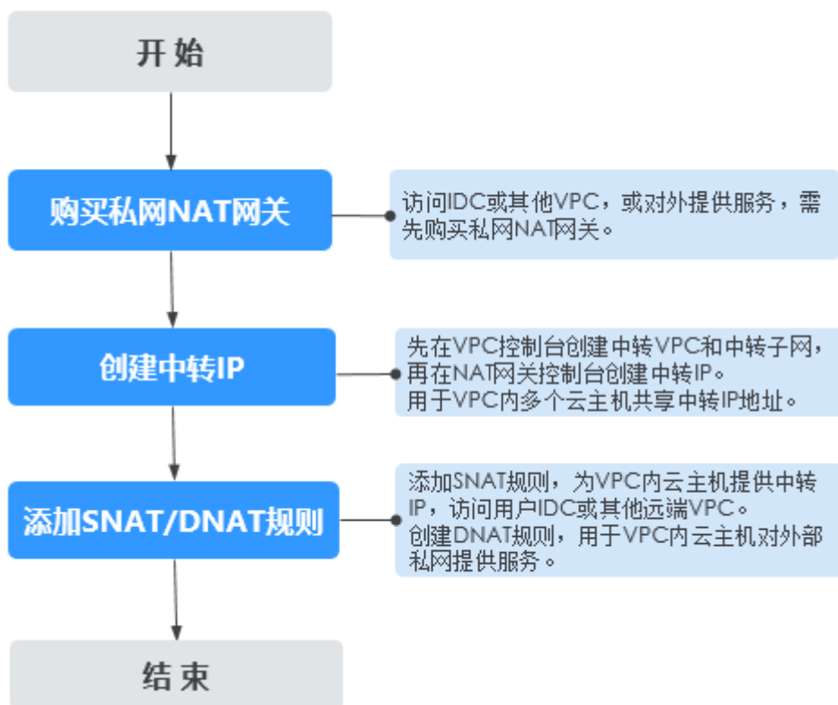
图 2-2 私有 NAT 使用流程
