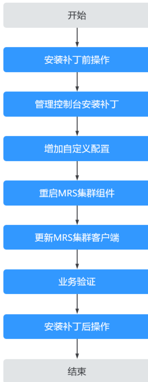
图 7-37 安装补丁流程
