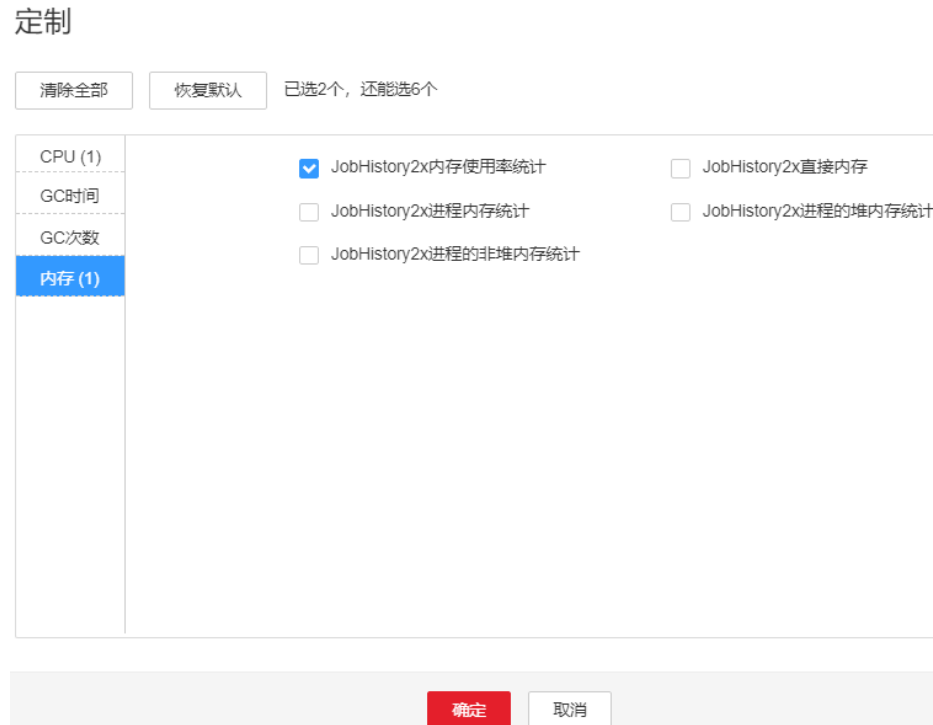
图 7-166 JobHistory2x 内存使用率统计
