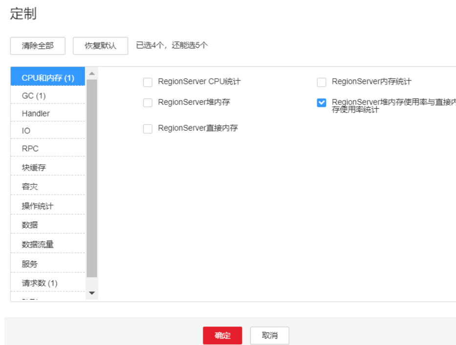
图 7-135 RegionServer 堆内存使用率与直接内存使用率统计
