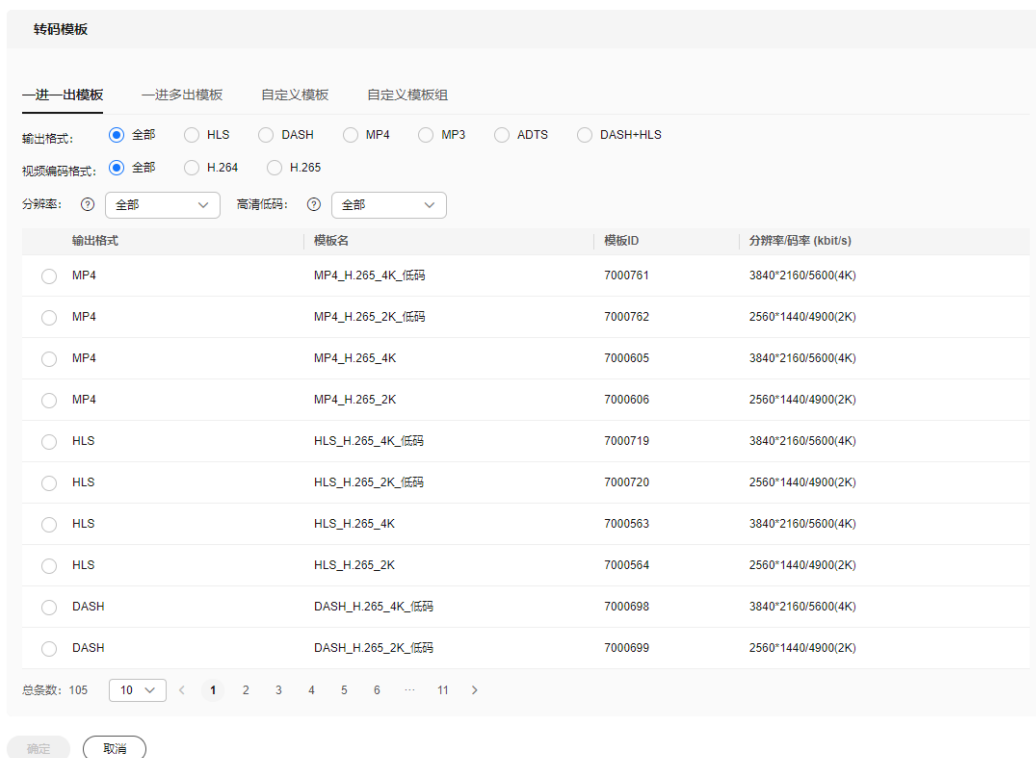
图 6-2 转码模板
