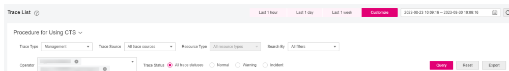
图 8-1 筛选框
