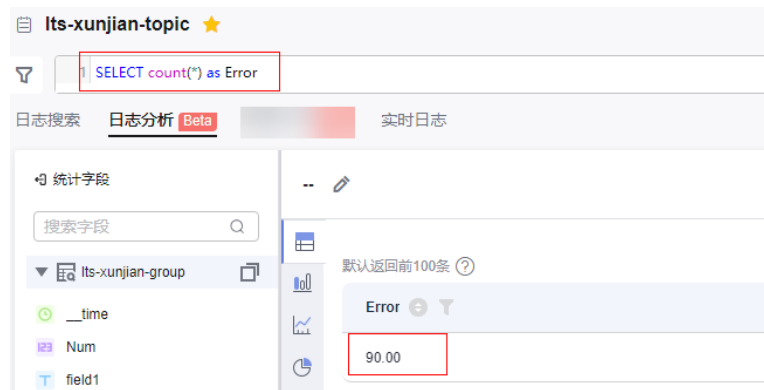
图 8-4 查询结果
