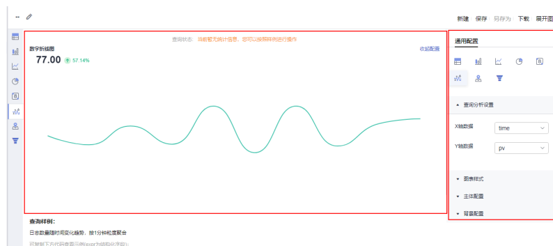
图 7-6 数字折线图
