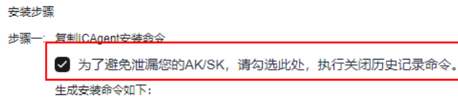
图 4-19 安装 ICAgent
