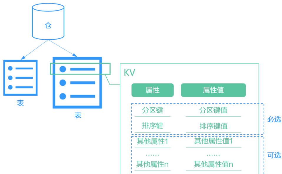
图 4-1 KV 简介
