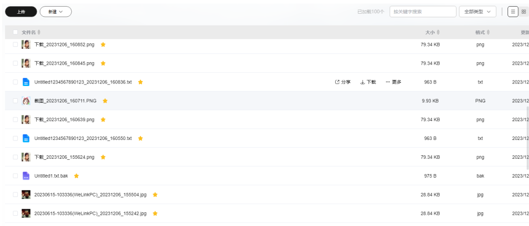
图 6-20 列表视图
