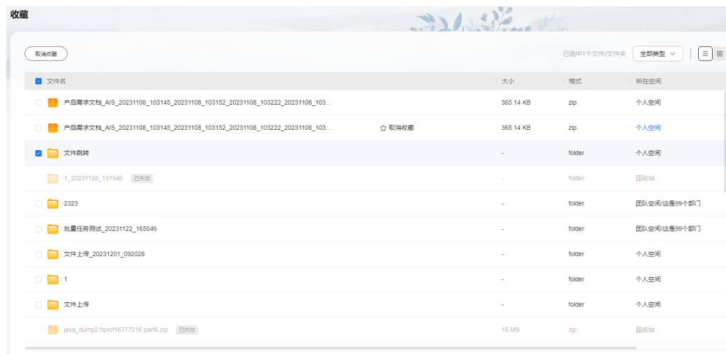
图 6-15 收藏页面
