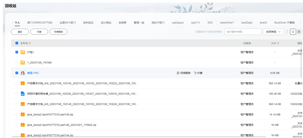
图 6-16 回收站页面
