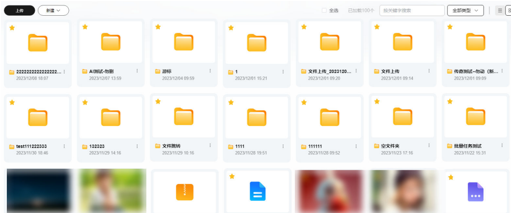
图 6-21 卡片视图
