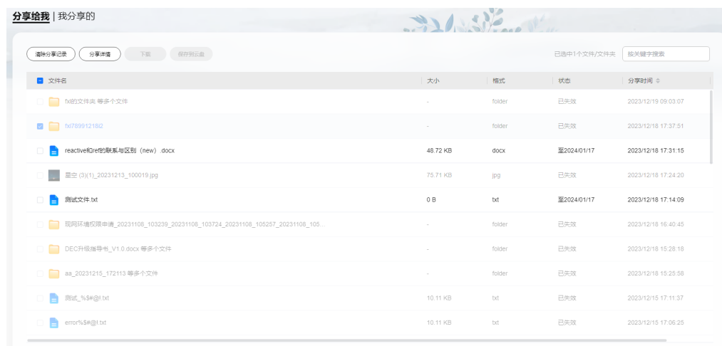
图 6-14 分享页面
