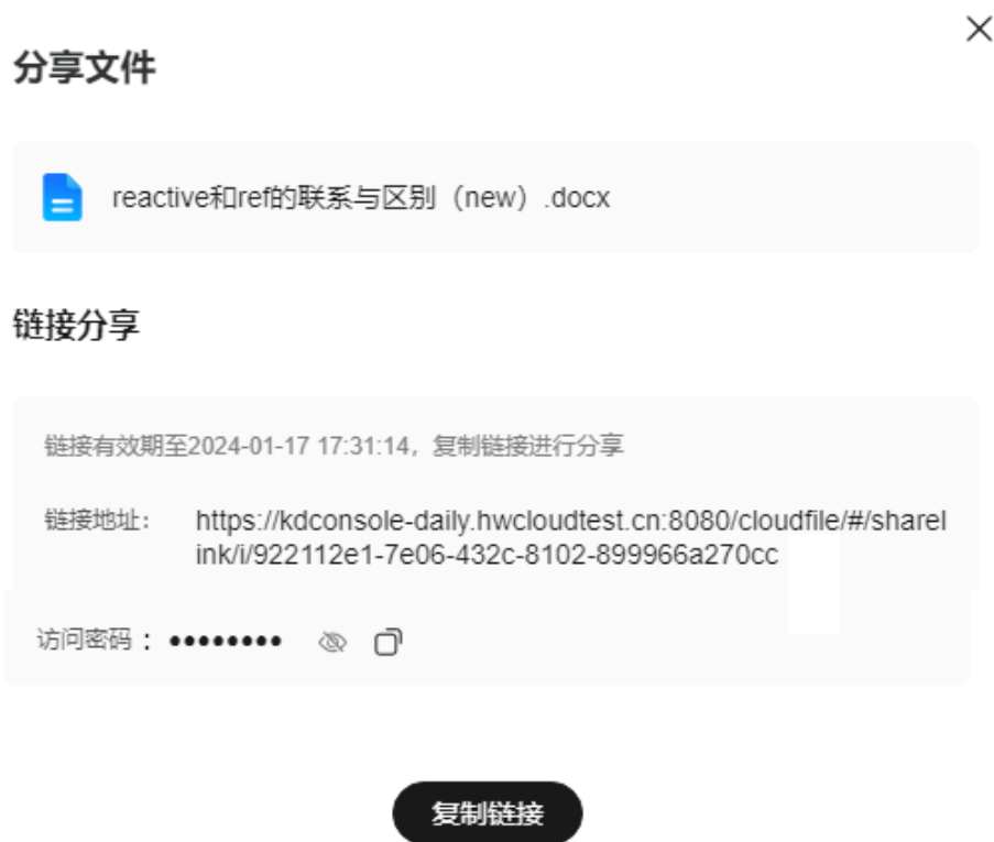
图 6-23 分享链接
