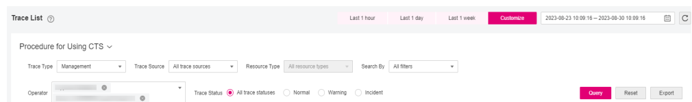
图 7-1 筛选框
