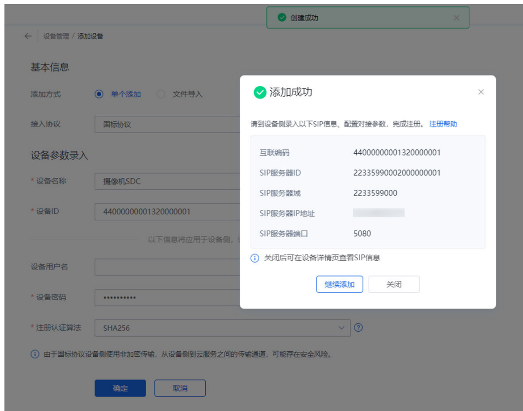
图 4-3 添加设备成功后展示的关键信息
