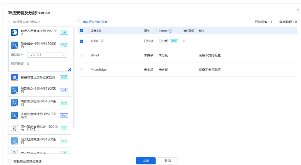
图 6-8 算法安装及分配 license
