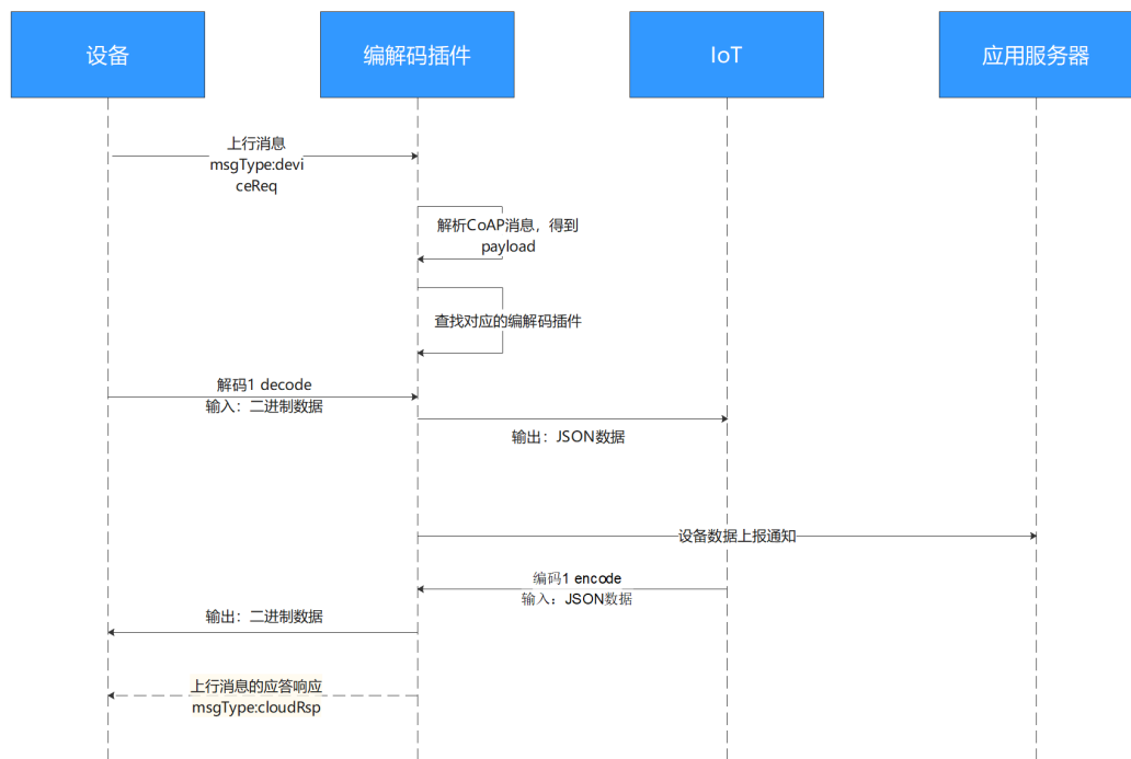
图 5-91 数据上报流程图
