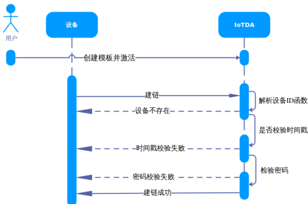
图 4-13 自定义模板鉴权流程图
