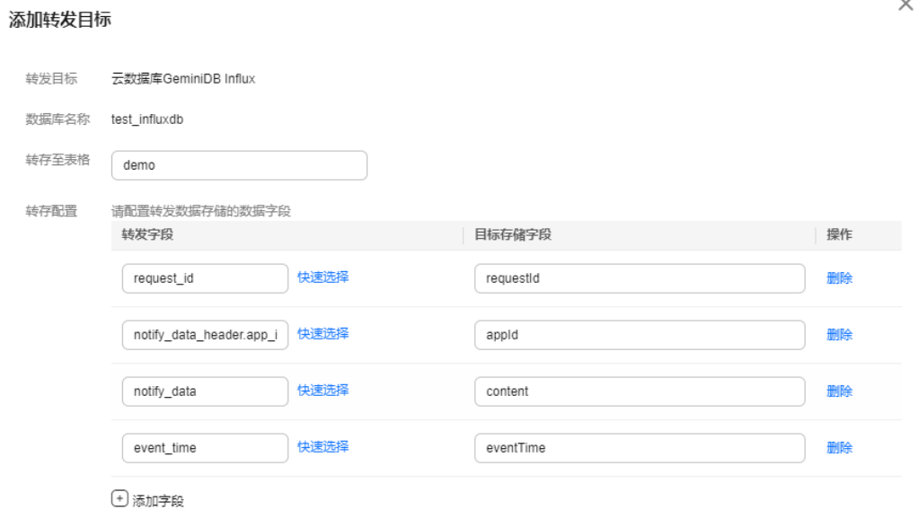
图 7-18 新建转发目标-设置 InfluxDB 字段映射
