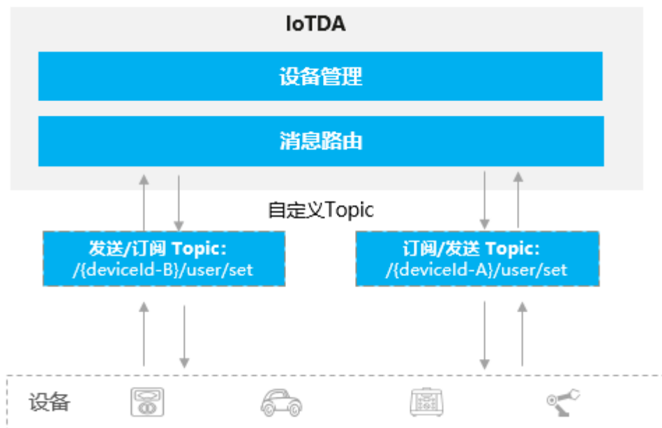
图 5-44 业务流程图
