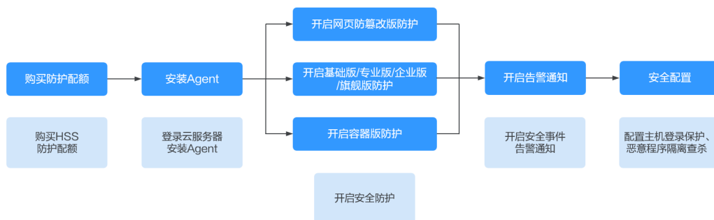
图 1-1 接入 HSS 流程
