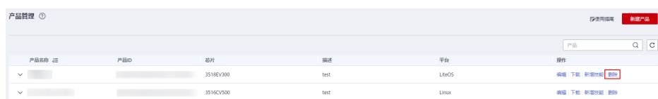
图 13-4 删除产品
