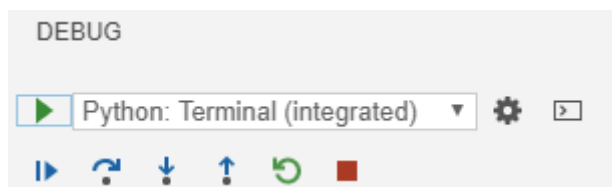
图 9-30 调试区
