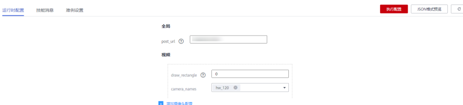
图 7-12 运行时配置-16
