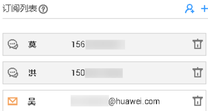
图 7-17 订阅列表
