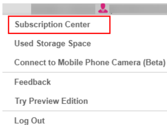
图 9-3 订购中心-24
