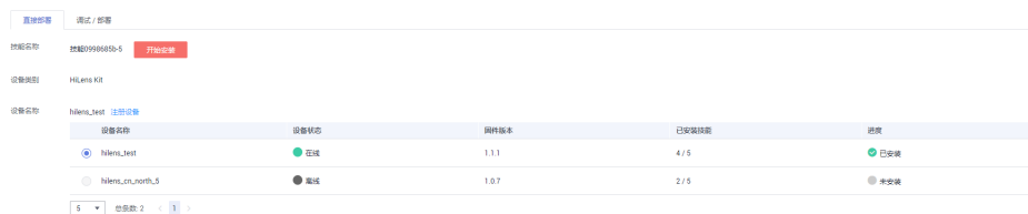
图 10-15 服务部署
