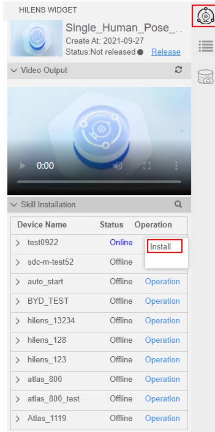
图 9-35 选择设备
