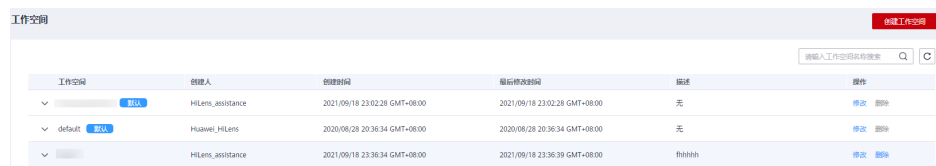
图 4-4 工作空间
