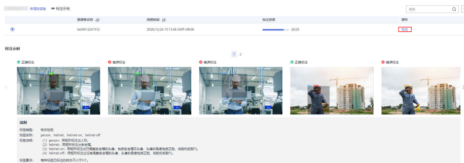
图 10-8 标注数据
