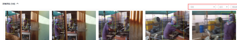
图 10-14 详细评估
