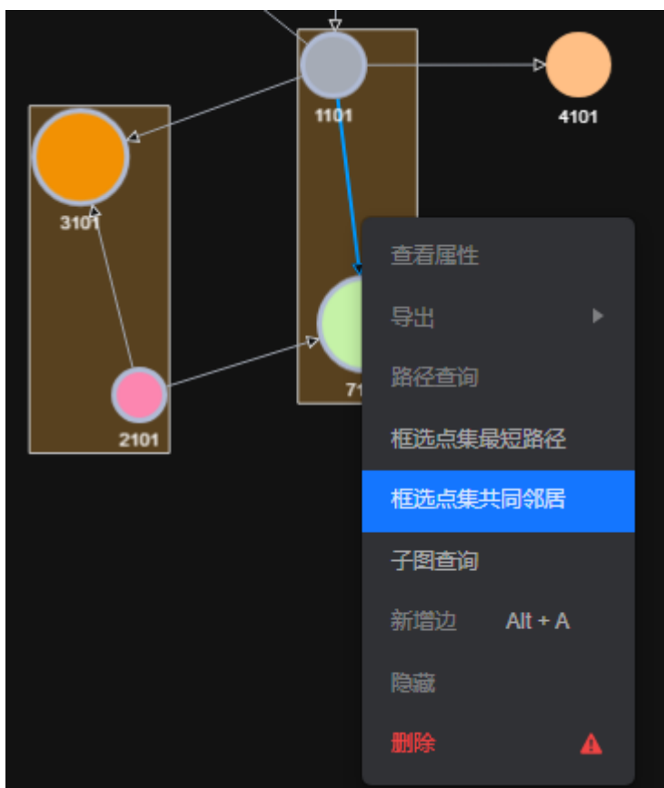
图 8-81 框选点集共同邻居
