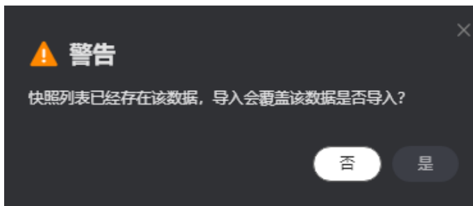
图 8-60 快照提示
