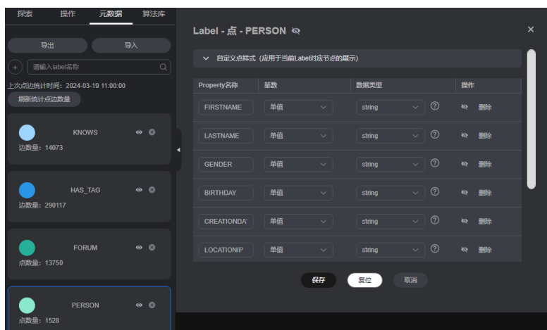
图 8-39 修改 label
