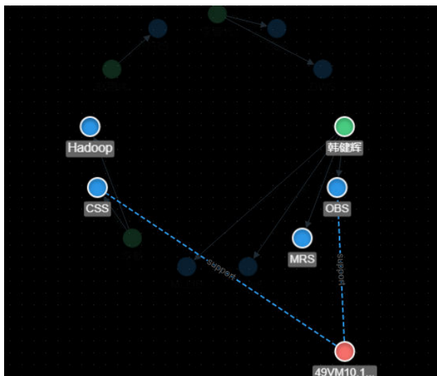
图 8-83 图展示
