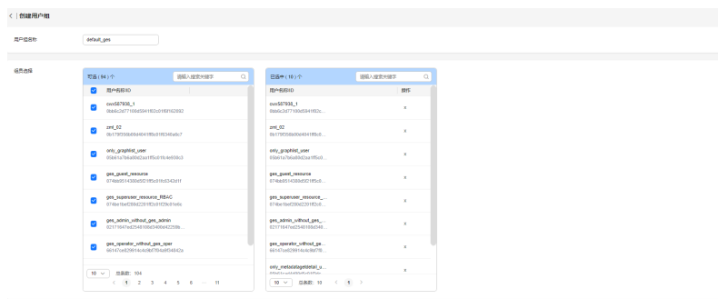
图 10-9 创建用户组
