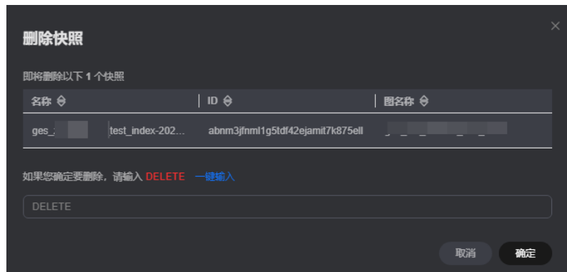
图 8-58 删除快照
