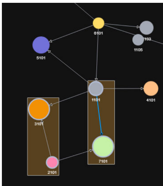
图 8-80 框选点集
