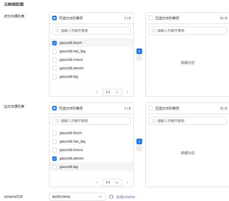
图 7-9 元数据配置
