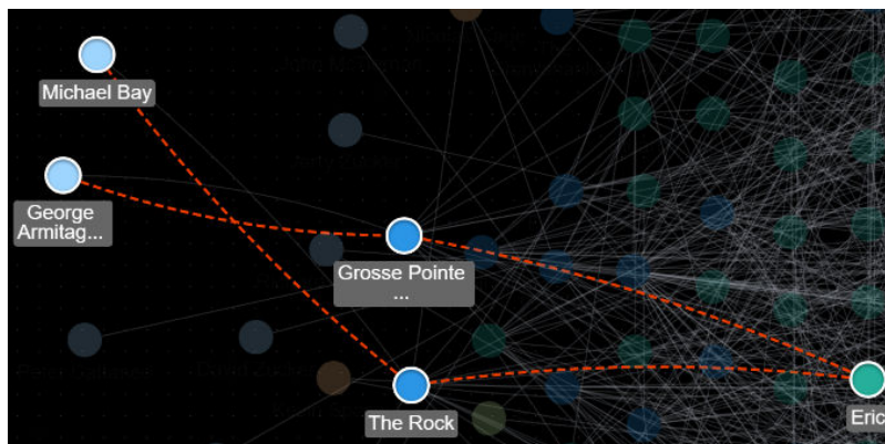
图 8-79 路径查询
