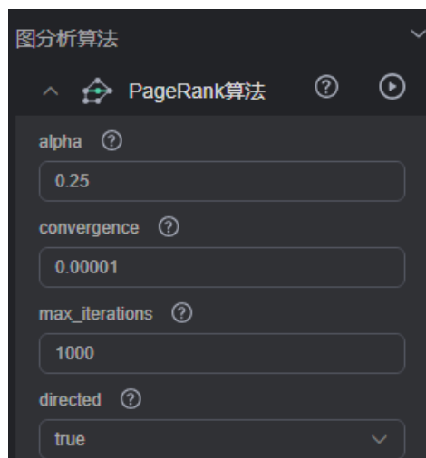
图 8-74 调整参数
