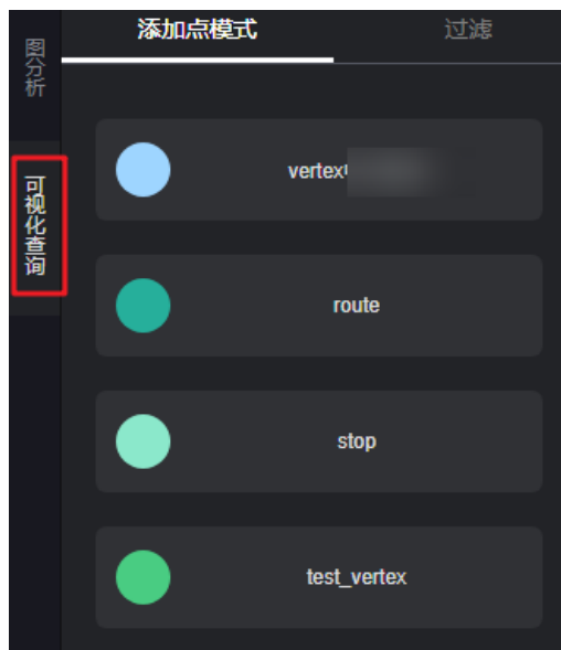
图 8-47 可视化查询
