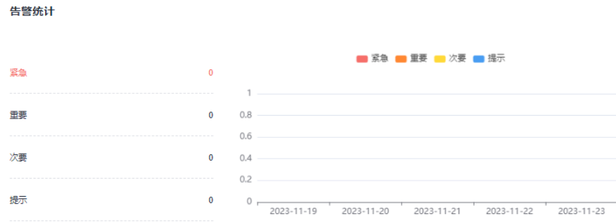
图 11-3 告警统计
