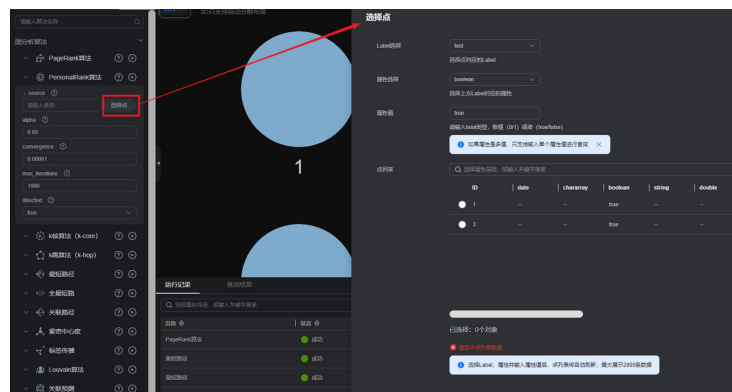
图 8-72 查询点
