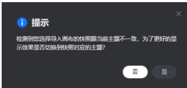
图 8-57 主题切换
