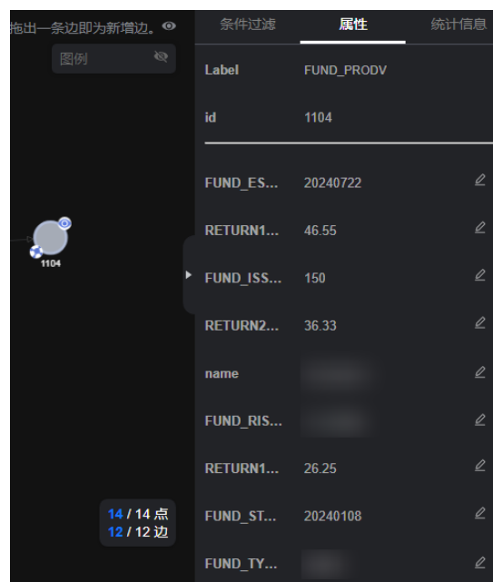
图 8-89 属性信息
