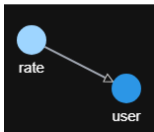
图 8-52 添加边
