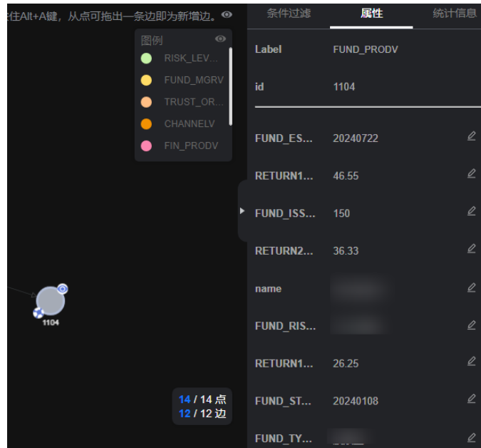
图 8-78 查看属性
