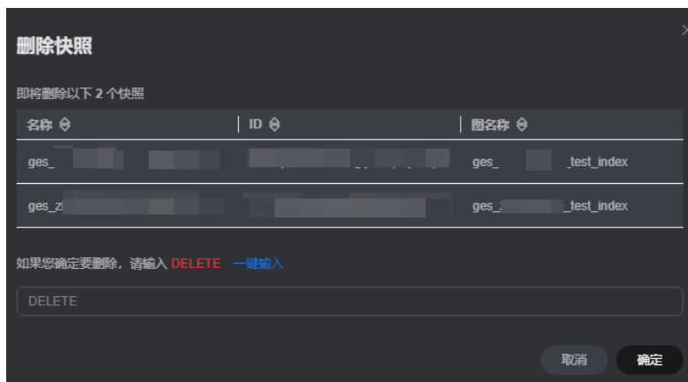
图 8-62 批量删除
