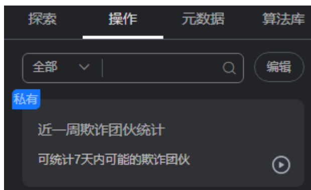
图 8-36 操作集
