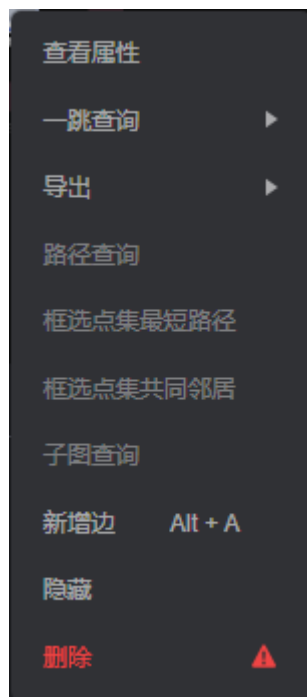
图 8-77 右键选项
