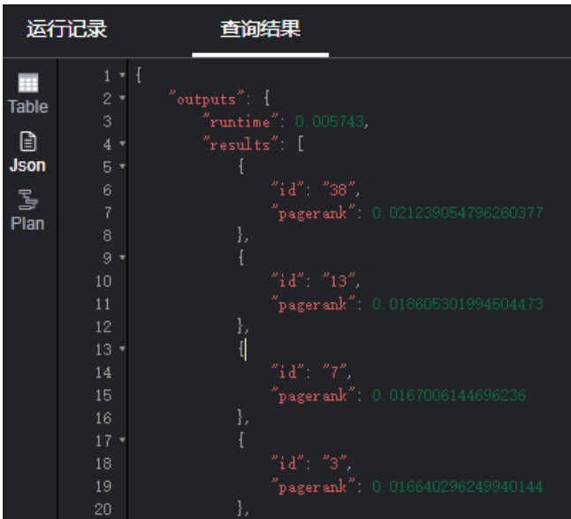
图 8-71 查询算法结果
