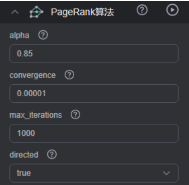
图 8-20 设置算法参数
