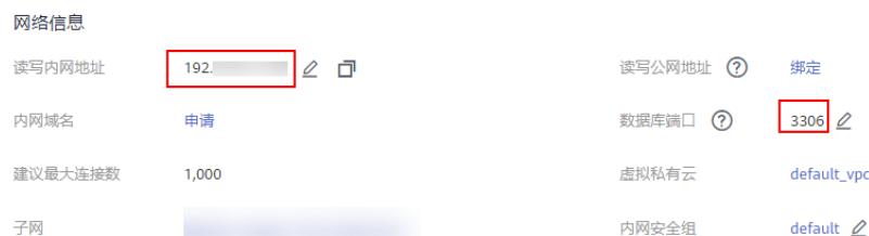
图 3-23 读写内网地址和数据库端口
