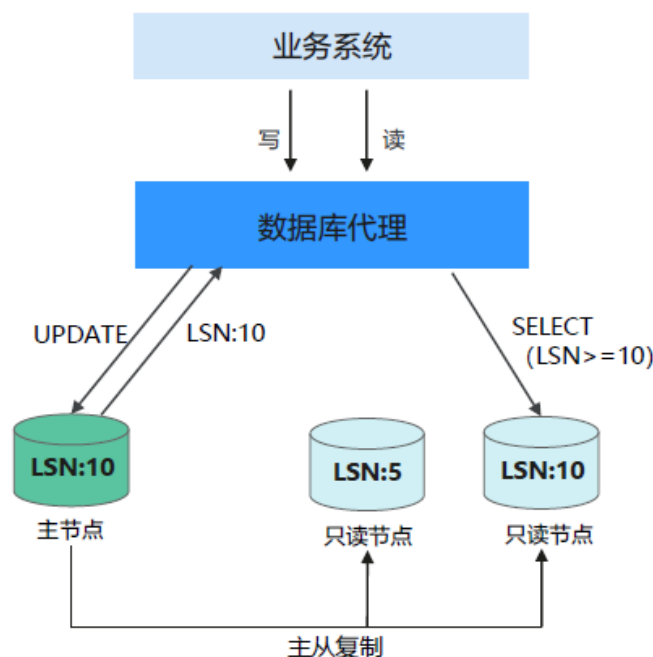
图 11-7 会话一致性实现原理
