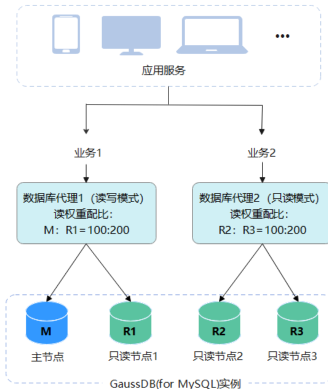
图 11-16 多代理下的读写分离（权重负载模式）
