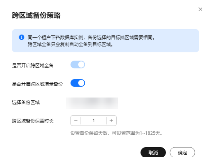
图 7-13 关闭跨区域备份方法一
