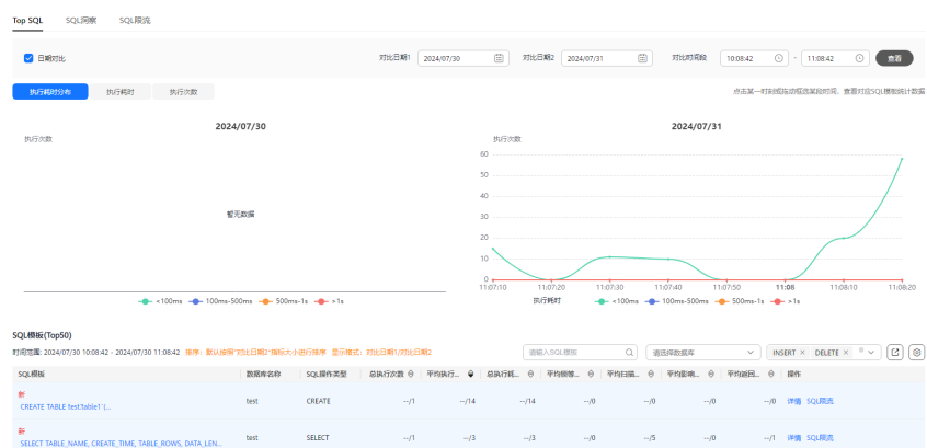
图 12-25 对比 TOP SQL
