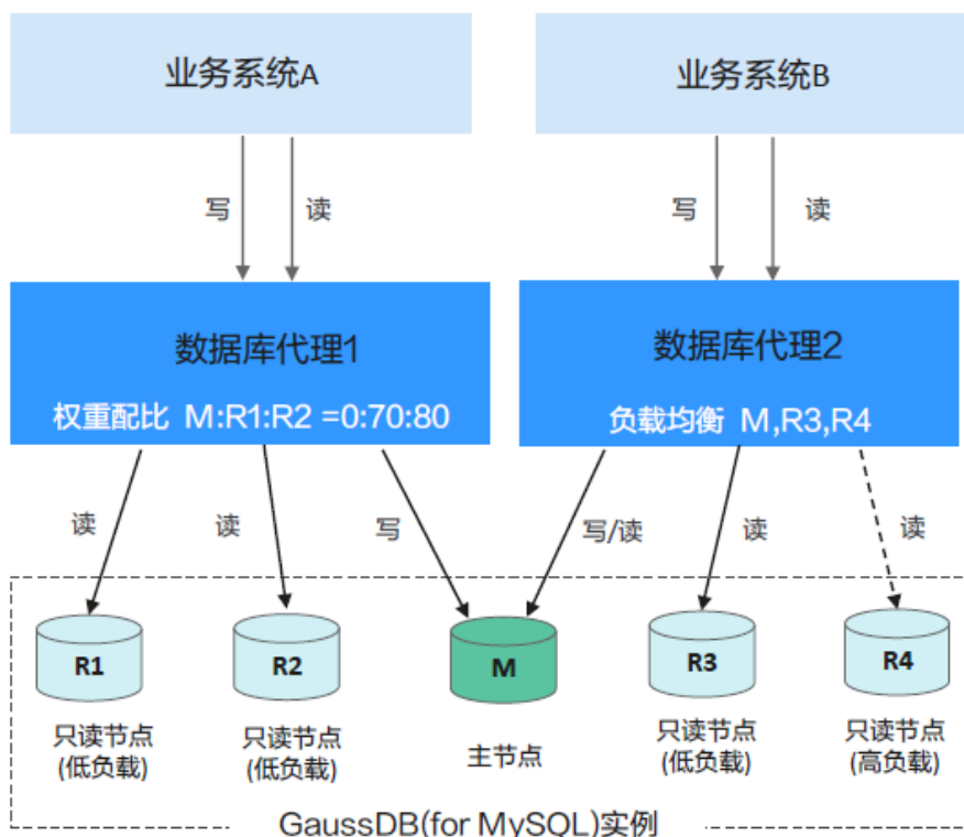
图 11-11 路由模式工作原理
