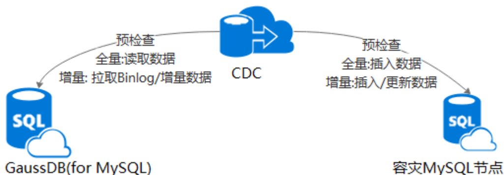
图 6-10 异构容灾实例
