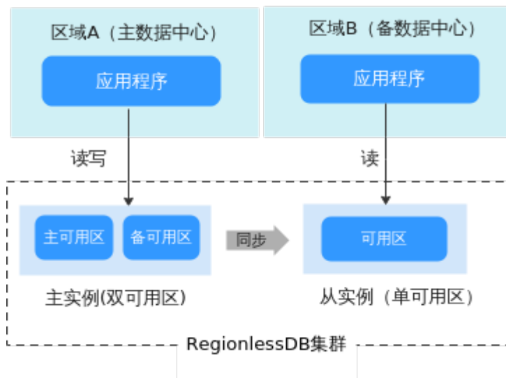
图 17-11 异地灾备原理图
