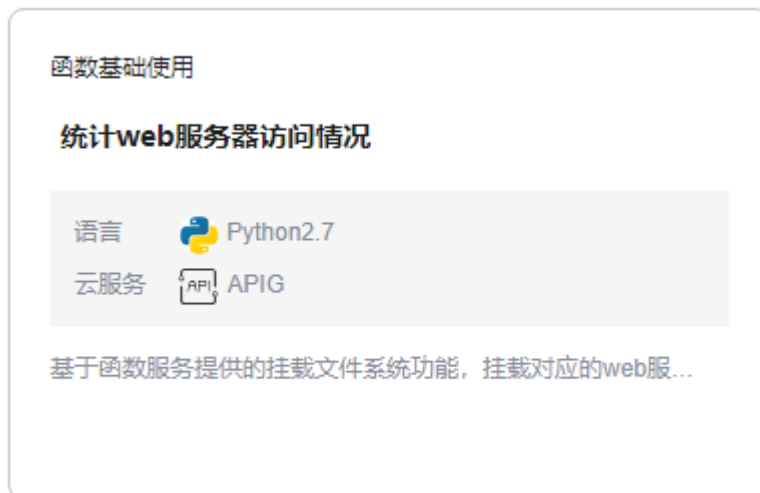
图 6-3 函数模板
