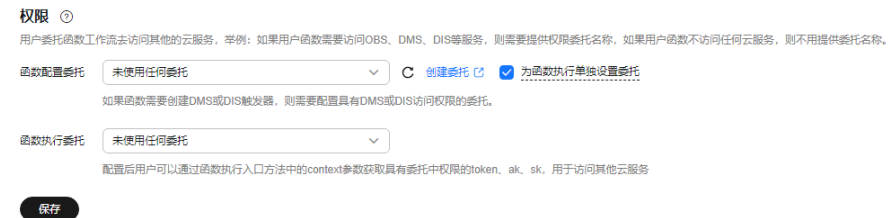
图 4-23 设置委托
