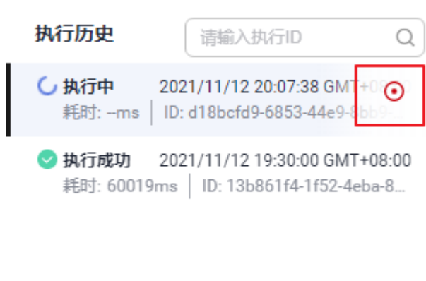
图 7-59 执行终止
