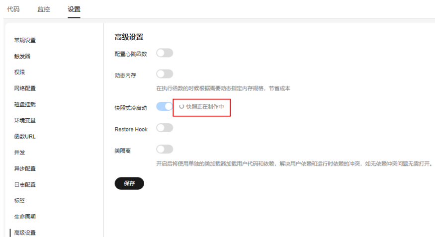
图 6-27 快照制作中
