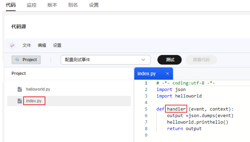
图 4-5 文件名和执行函数名
