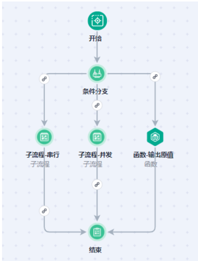
图 7-10 包含子流程的函数流
