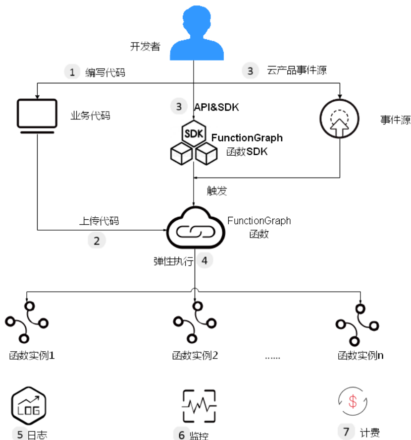
图 4-1 函数使用流程
