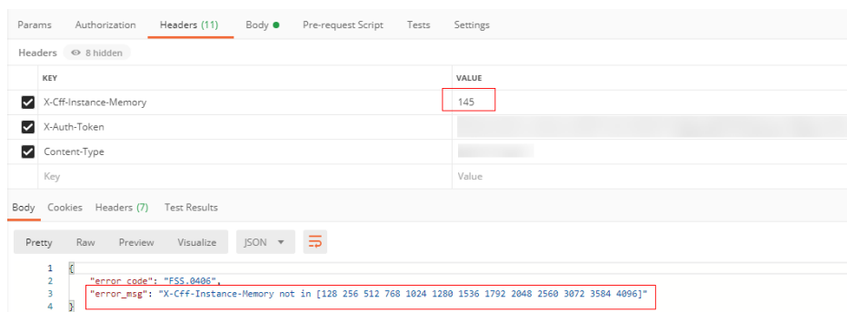
图 6-16 调用失败
