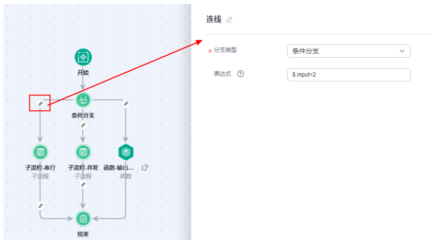
图 7-14 子流程-串行
