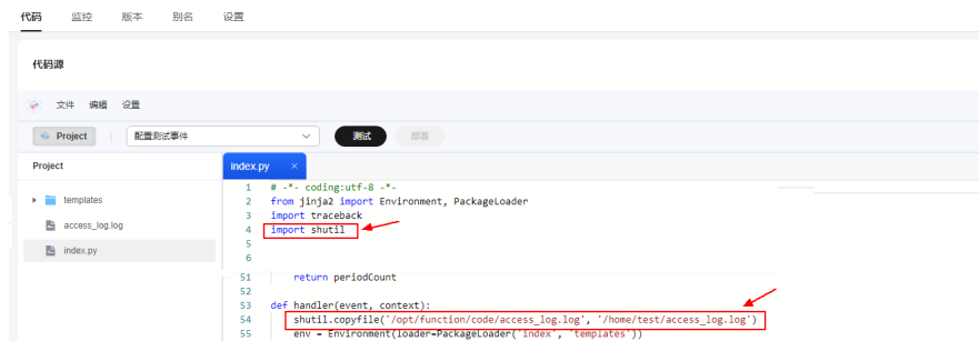
图 6-3 添加代码
