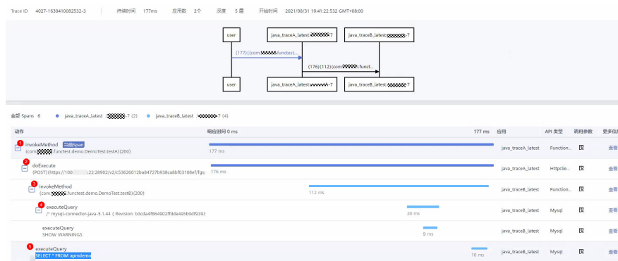
图 11-19 函数 A 调用函数 B 详情
