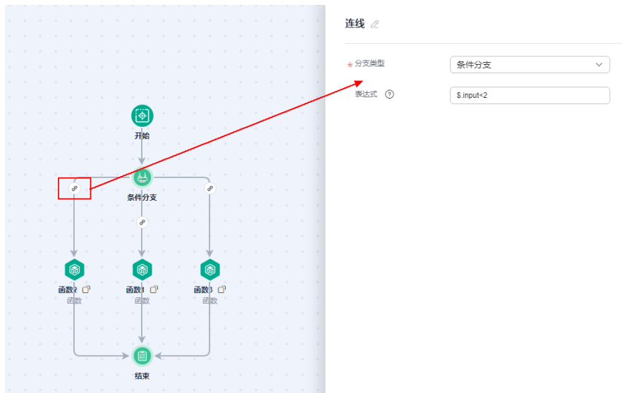
图 7-49 函数 2 条件分支
