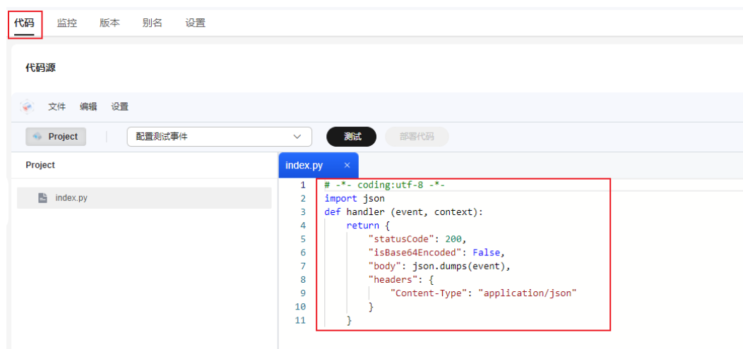
图 4-2 在线编辑函数代码
