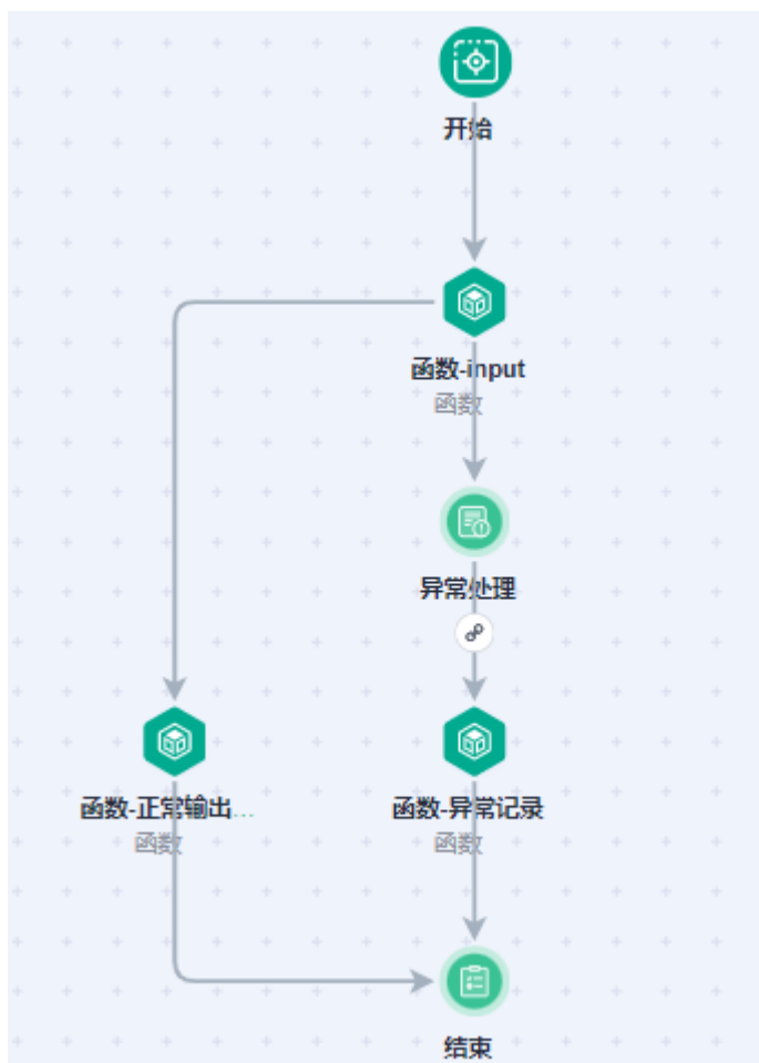
图 7-26 异常处理函数流编排
