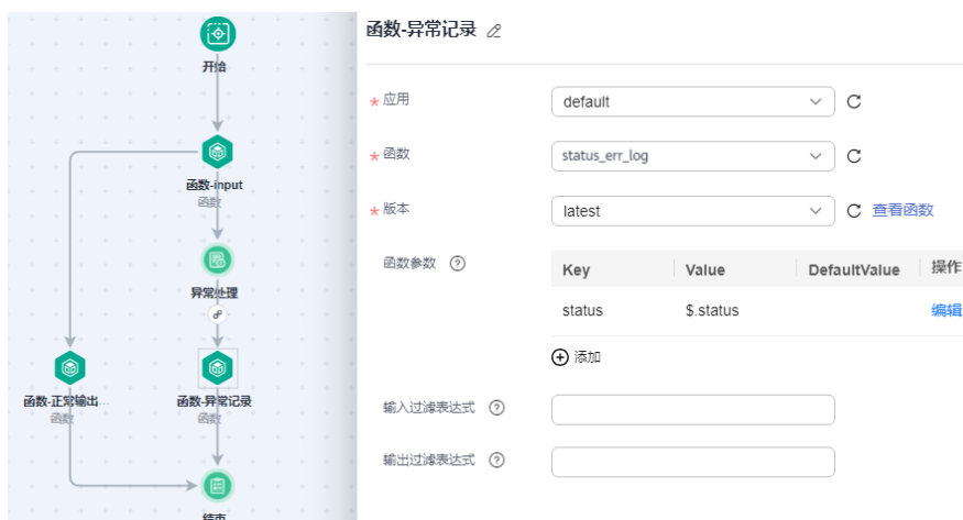
图 7-29 配置异常处理
