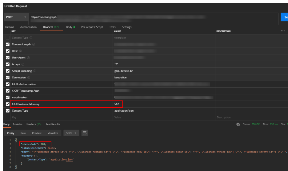
图 6-18 添加请求头并调用
