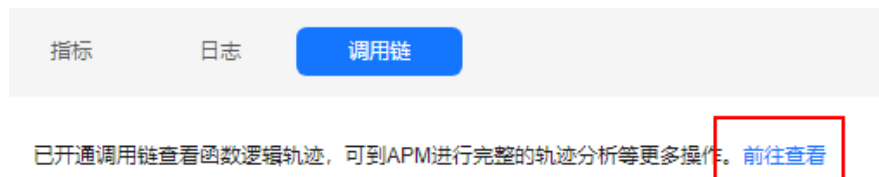
图 11-18 前往 APM
