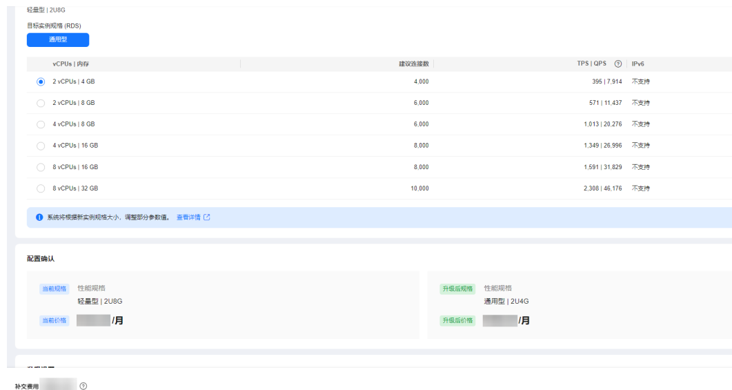
图 6-1 升级至 RDS
