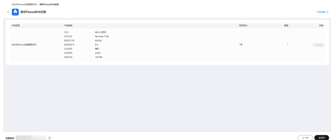
图 2-3 订单确认
