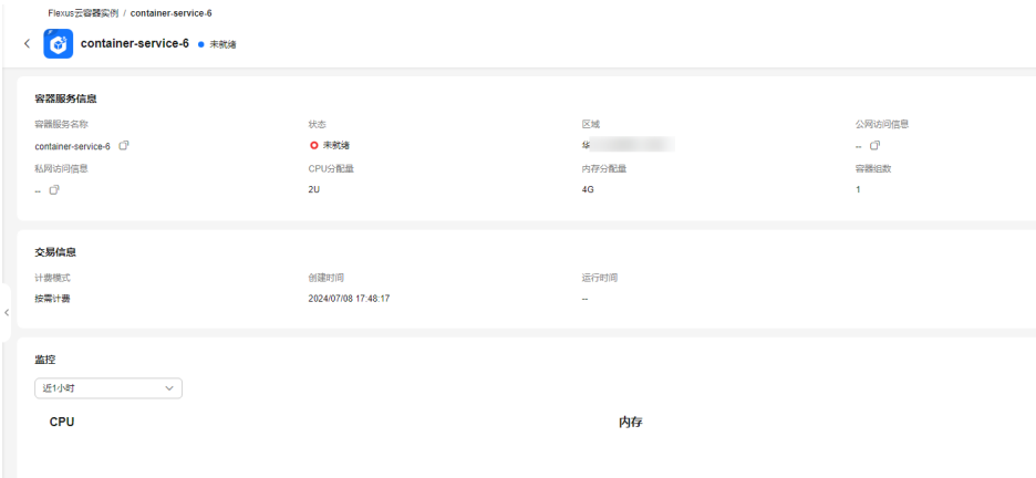
图 3-1 实例详情
