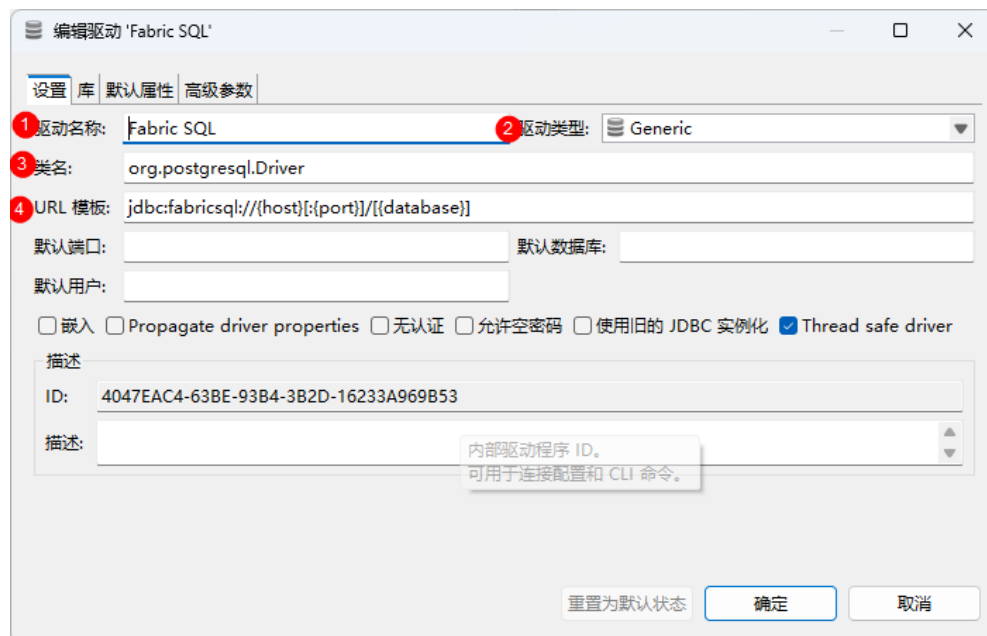
图 3-10 设置 DataArtsFabric SQL 驱动
