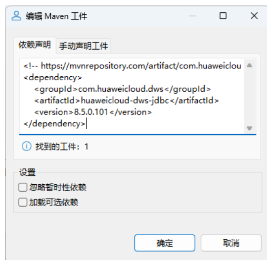
图 3-7 添加 Maven 依赖
