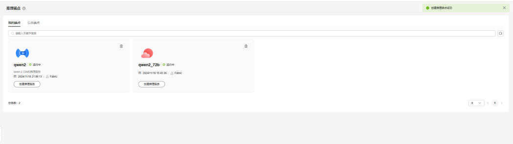
图 4-21 推理端点
