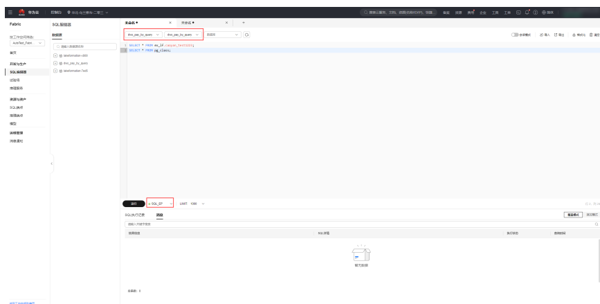
图 3-1 运行 SQL
