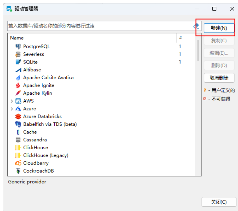
图 3-6 驱动管理器
