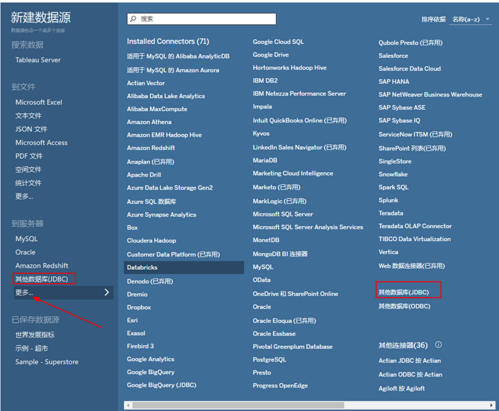
图 3-15 JDBC 方式连接 DataArtsFabric SQL
