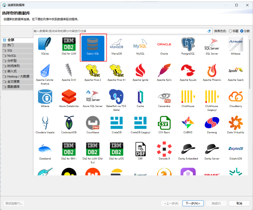
图 3-12 选择数据库
