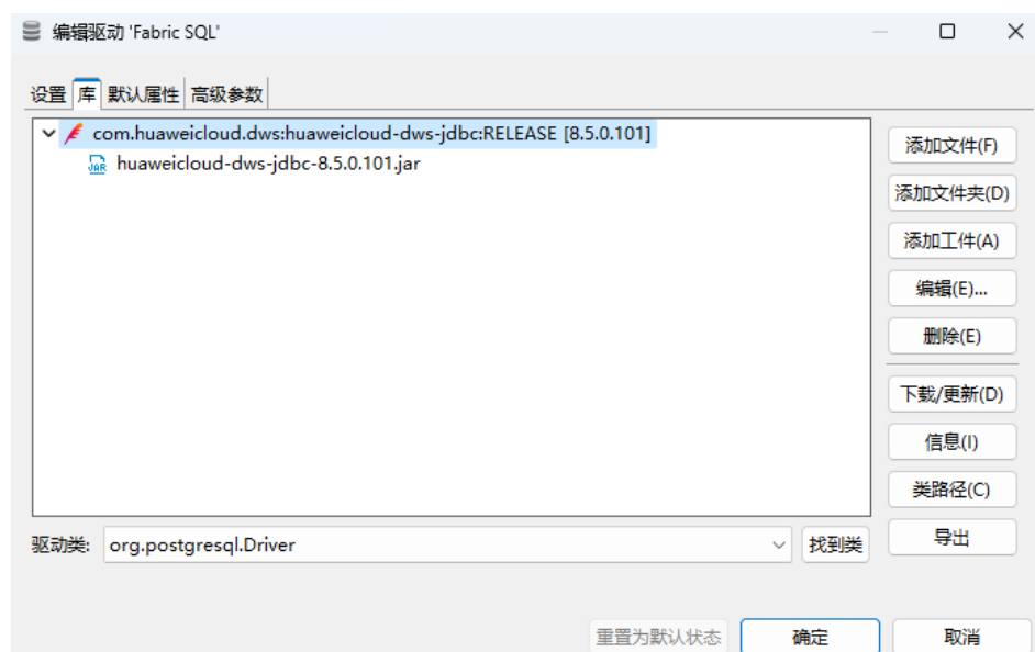
图 3-9 设置驱动类
