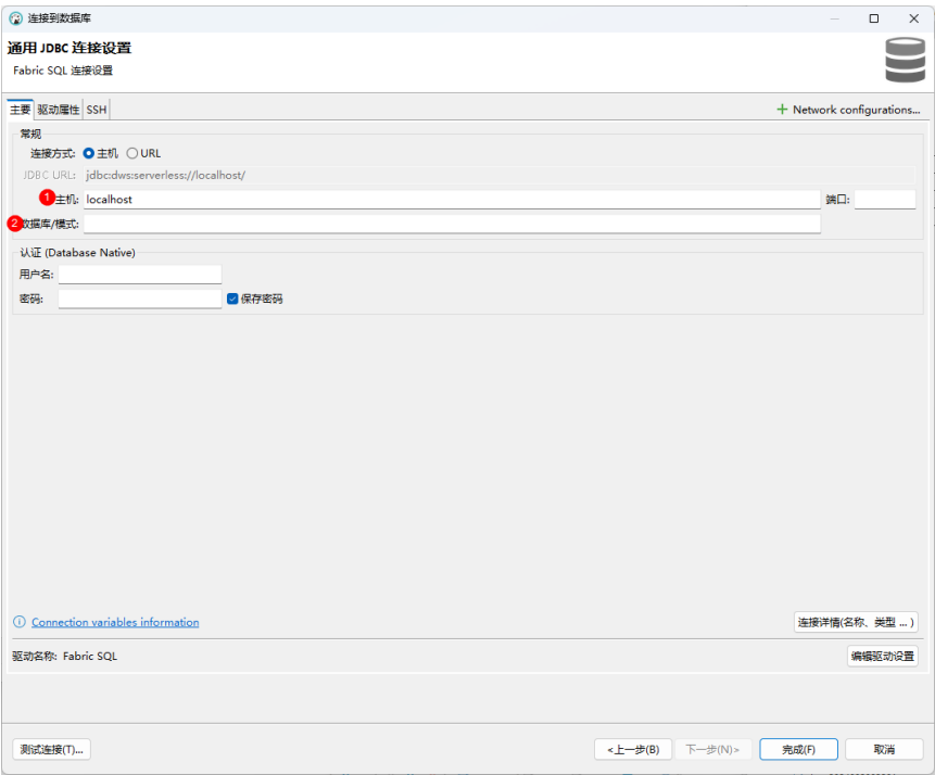
图 3-13 “主要”页签
