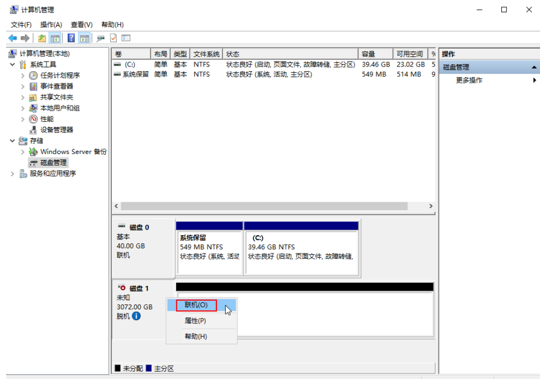
图 6-14 磁盘联机
