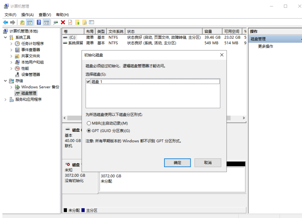
图 6-11 磁盘列表
