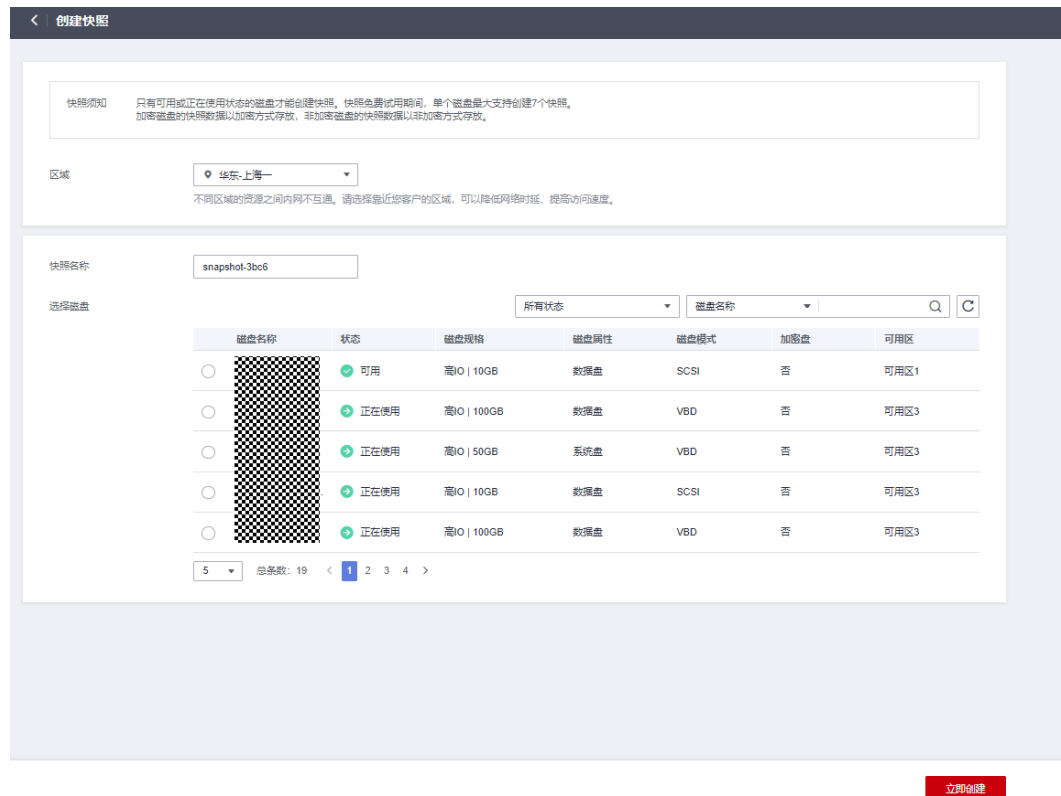
图 9-2 创建快照
