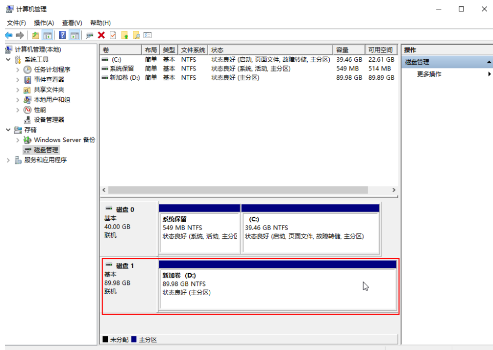
图 6-8 扩容成功
