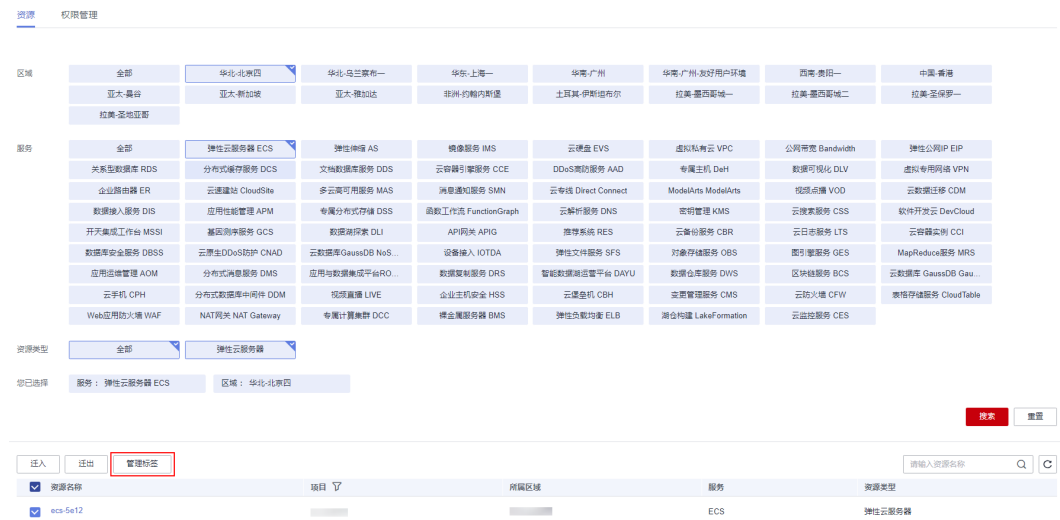
图 2-58 管理标签
