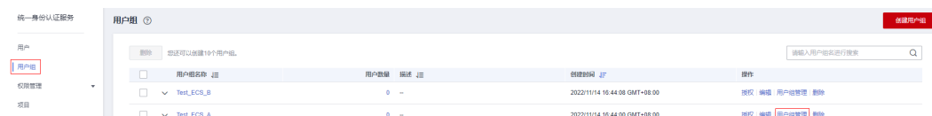
图 2-14 用户组管理
