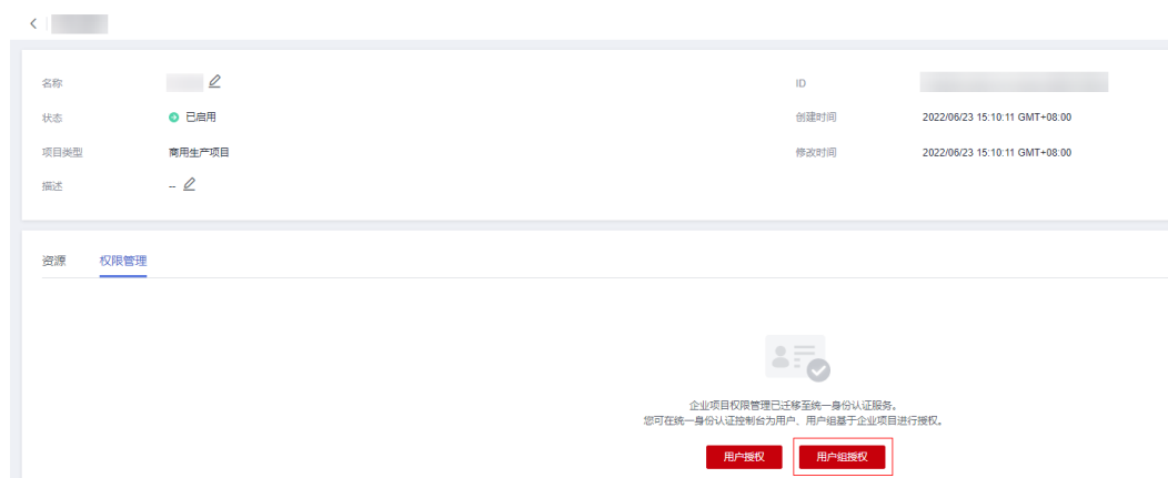
图 2-64 用户组授权
