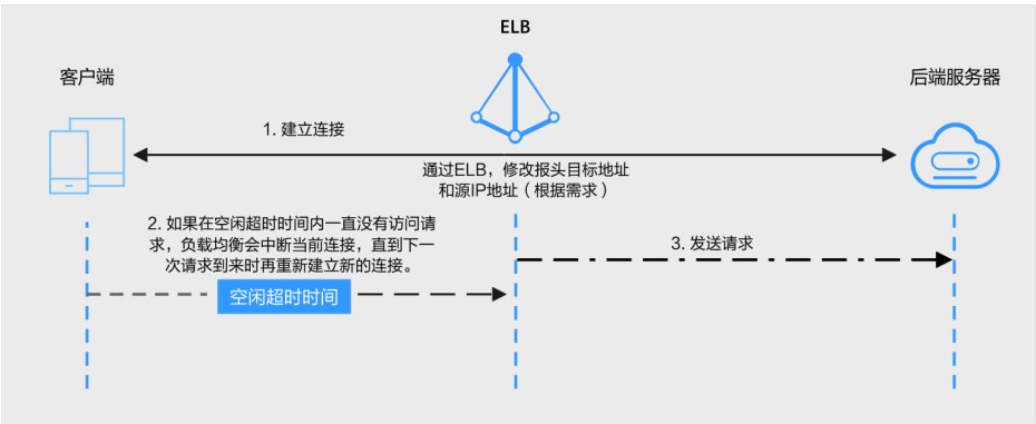
图 1-12 四层监听器超时时间示意图
