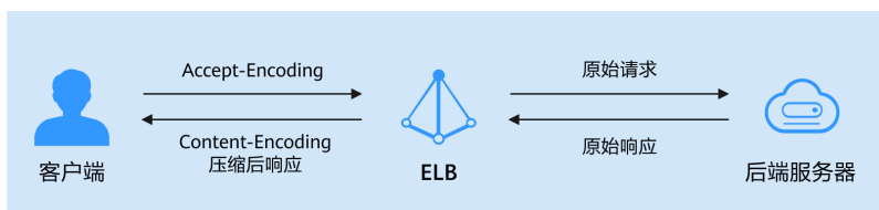
图 1-17 负载均衡器进行压缩示意图
