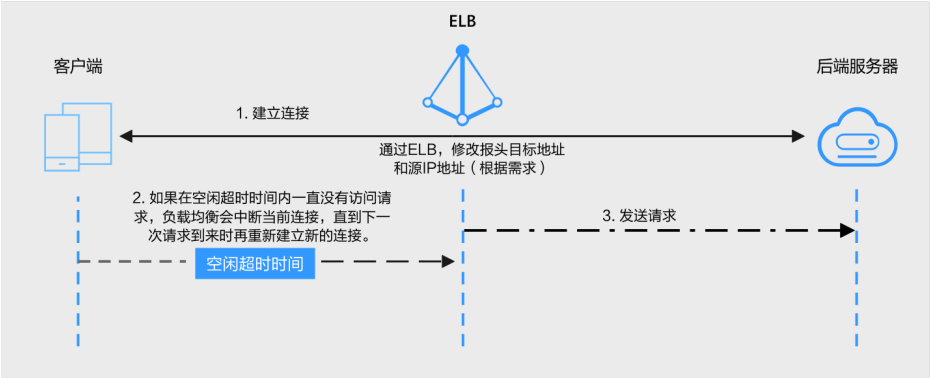
图 1-11 四层监听器超时时间示意图
