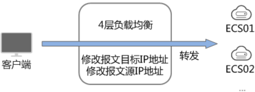
图 1-4 网络型负载均衡
