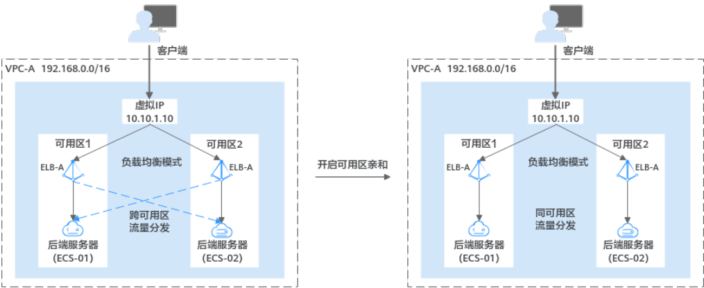
图 1-28 开启可用区亲和转发示意图
