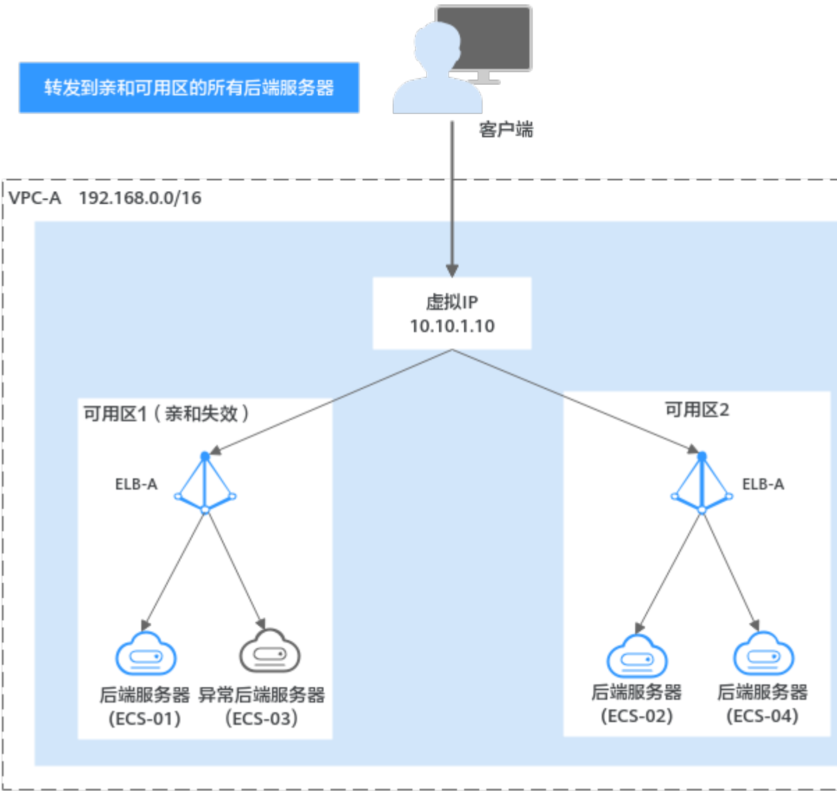
图 1-31 转发亲和可用区的所有后端服务器示意图
