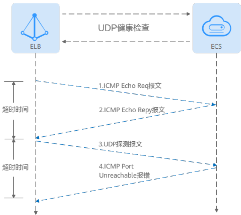
图 2-18 UDP 健康检查
