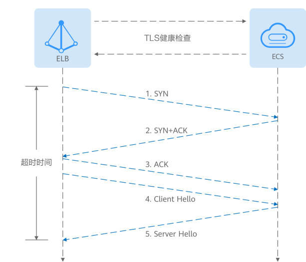
图 1-38 TLS 健康检查
