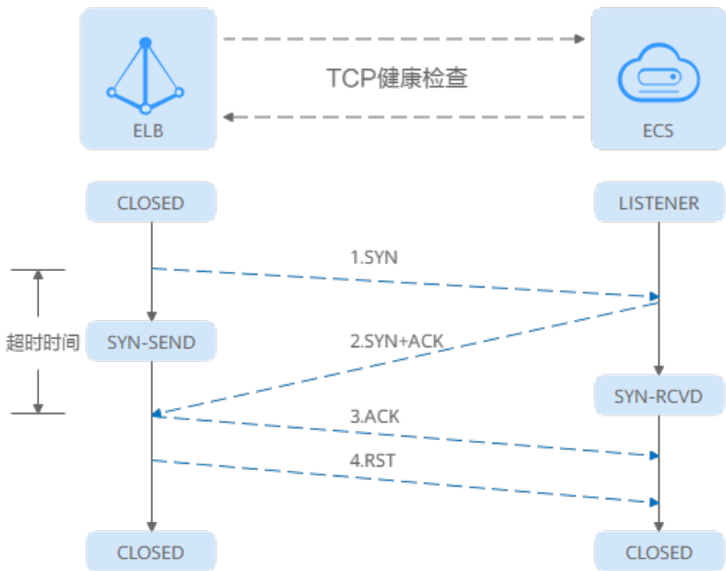
图 2-17 TCP 健康检查
