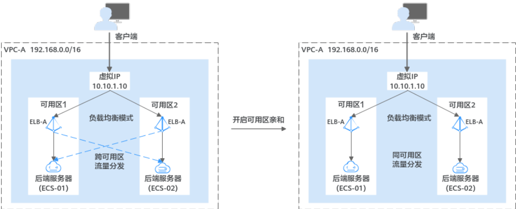
图 1-28 开启可用区亲和转发示意图
