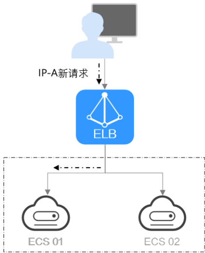
图 1-25 源 IP 算法流量分发
