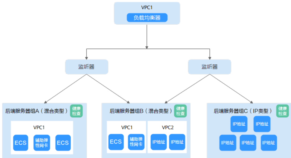
图 1-22 后端服务器组使用架构图
