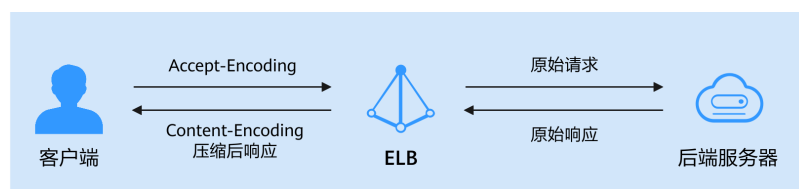
图 1-17 负载均衡器进行压缩示意图
