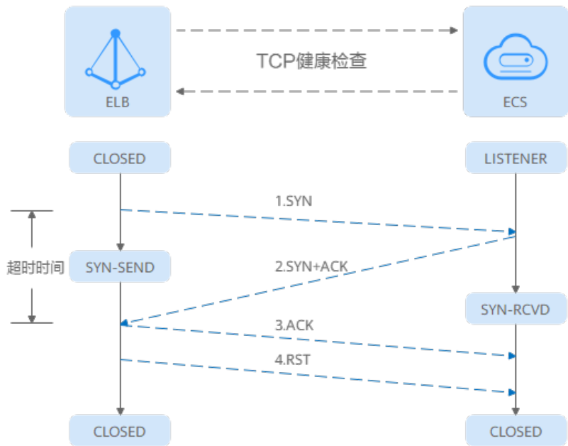
图 1-34 TCP 健康检查
