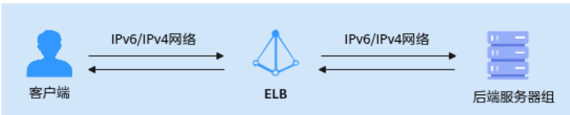
图 1-7 TCP 和 UDP 协议开启 IPv4/IPv6 地址转换业务架构图
