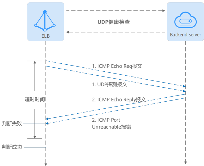
图 1-35 UDP 健康检查
