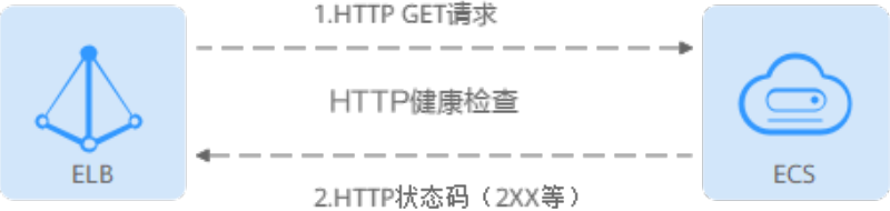
图 2-19 HTTP 健康检查
