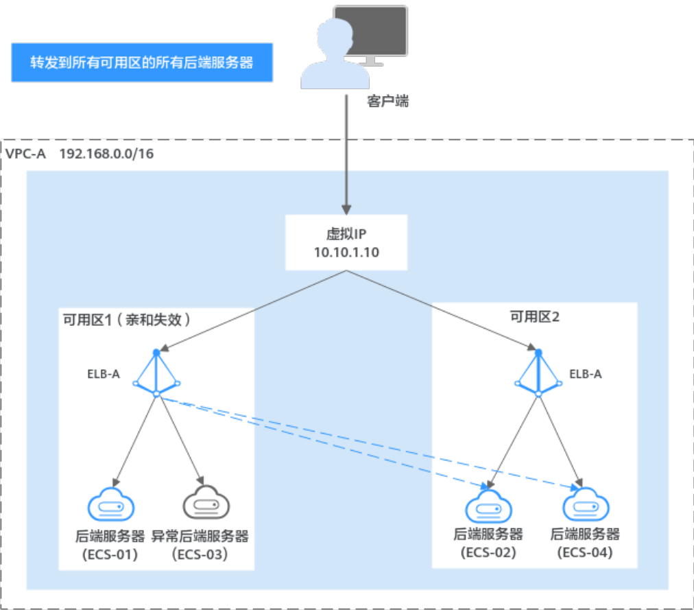
图 1-32 转发所有可用区的所有后端服务器示意图
