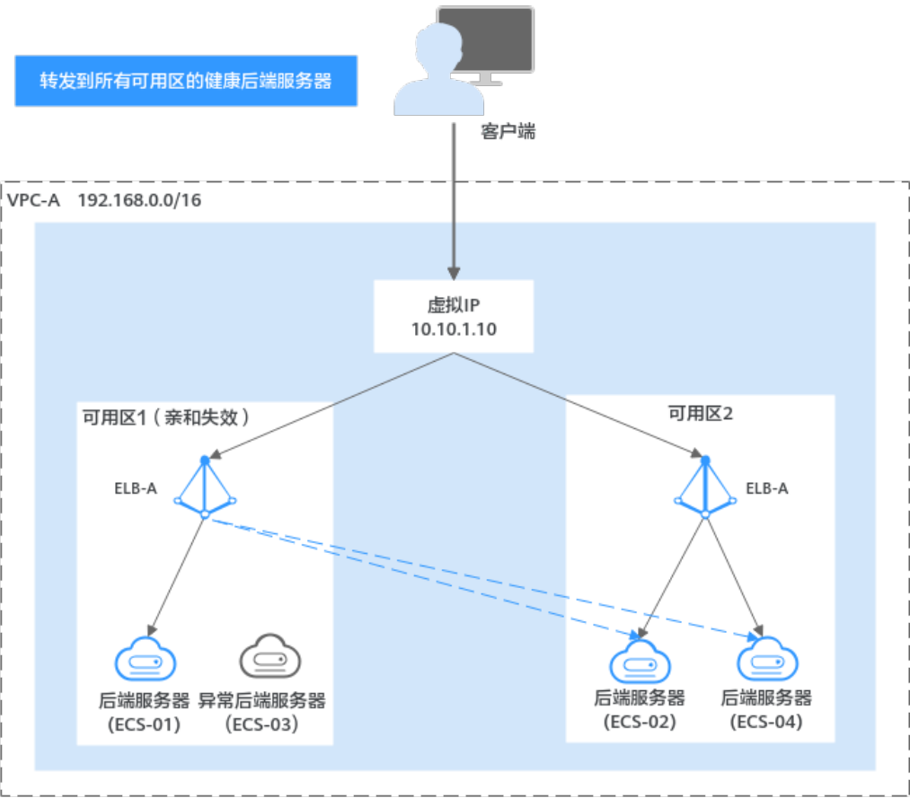
图 1-29 转发到所有可用区的健康后端服务器示意图
