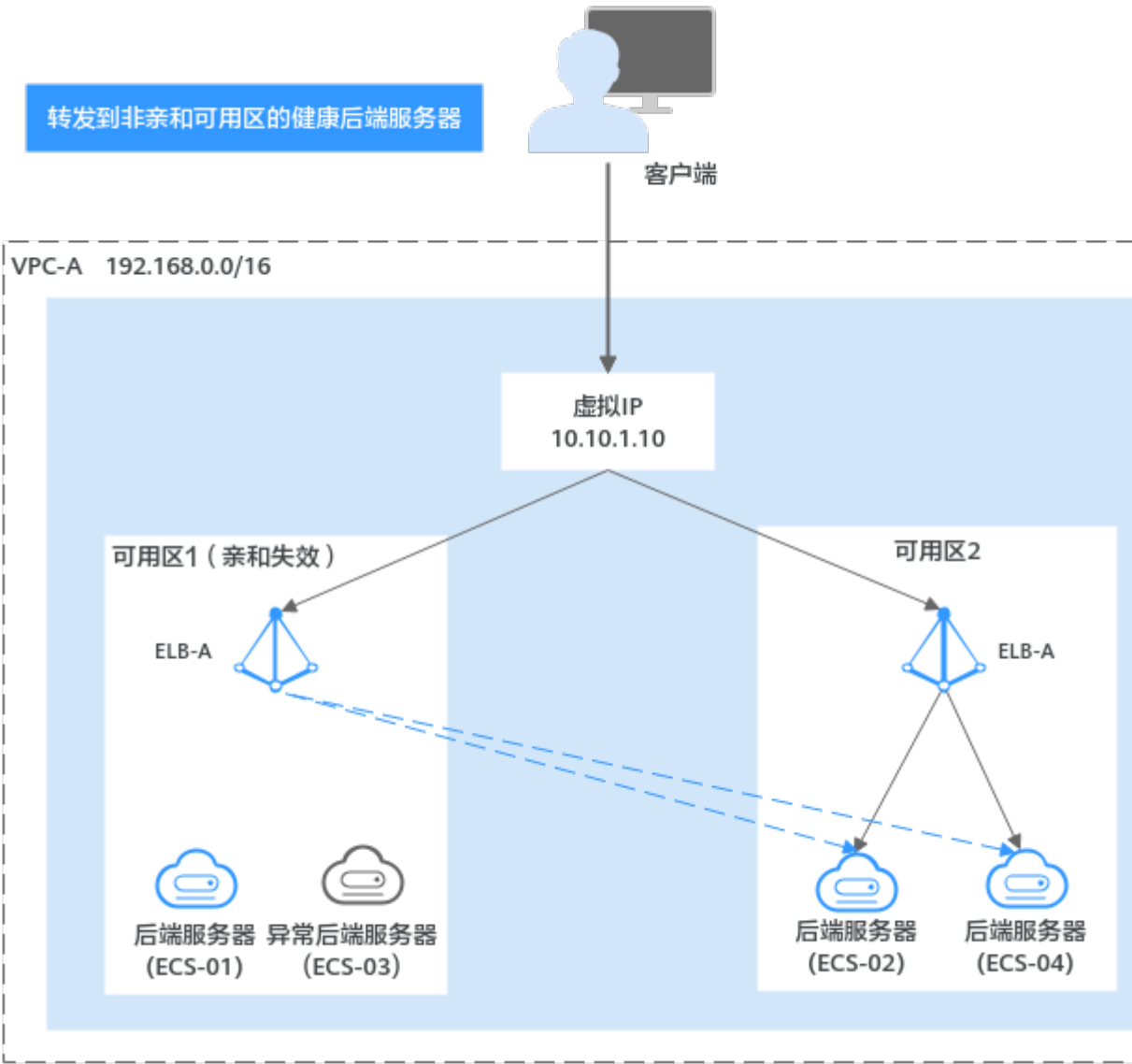
图 1-30 转发非亲和可用区的健康后端服务器示意图
