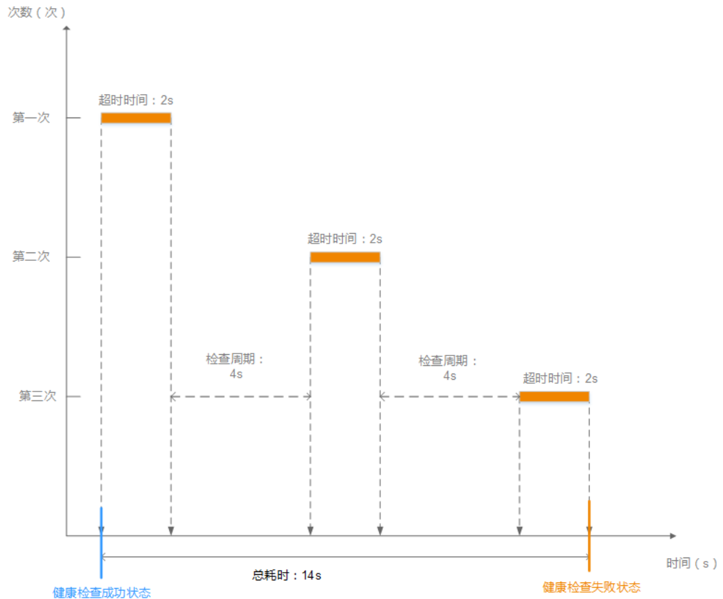
图 2-20 健康检查失败时间窗
