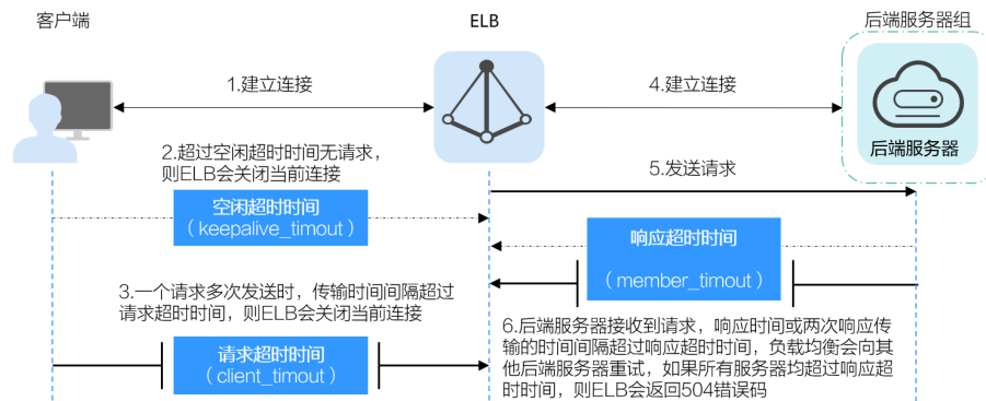
图 1-7 七层监听器超时时间示意图
