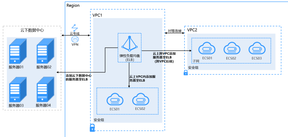
图 1-20 ELB 支持添加云上、云下的服务器
