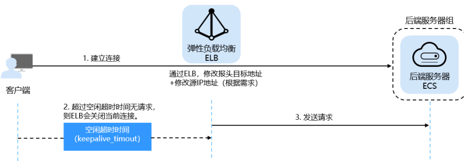
图 1-4 四层监听器超时时间示意图
