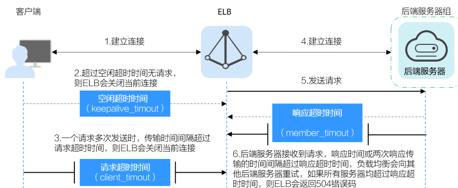
图 1-5 七层监听器超时时间示意图
