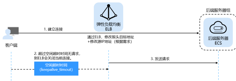
图 1-5 四层监听器超时时间示意图
