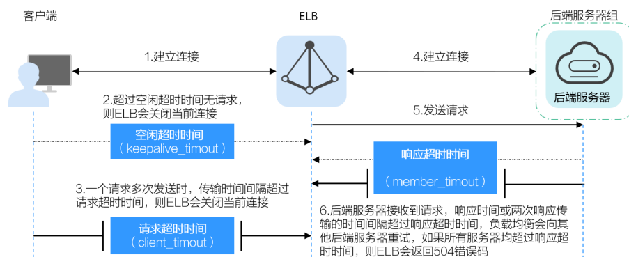
图 1-6 七层监听器超时时间示意图
