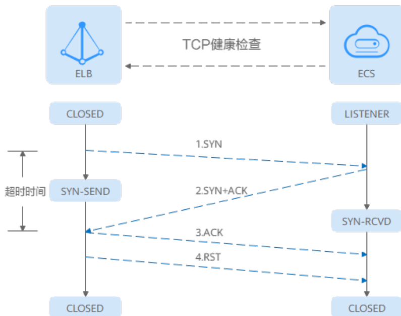
图 1-13 TCP 健康检查
