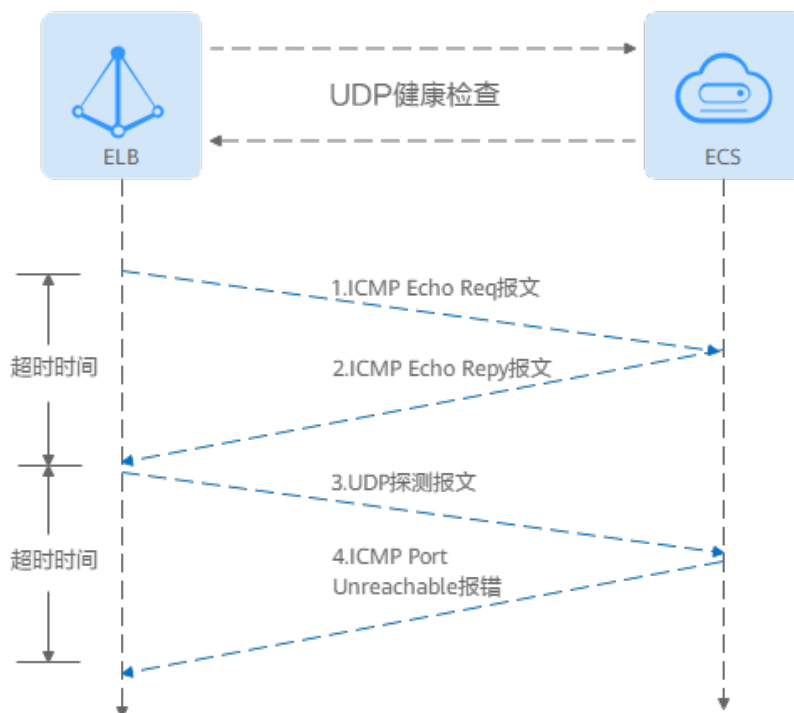
图 2-8 UDP 健康检查
