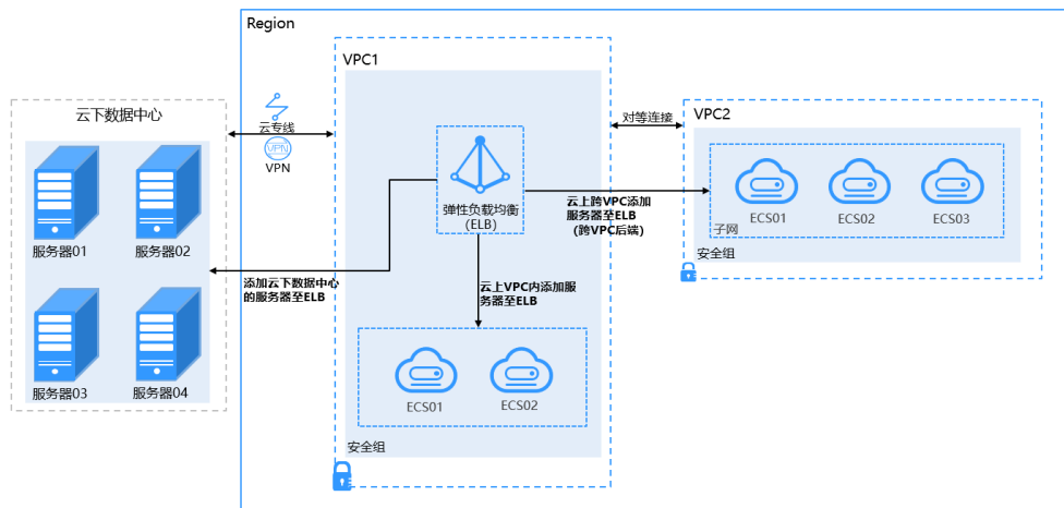
图 1-25 ELB 支持添加云上、云下的服务器
