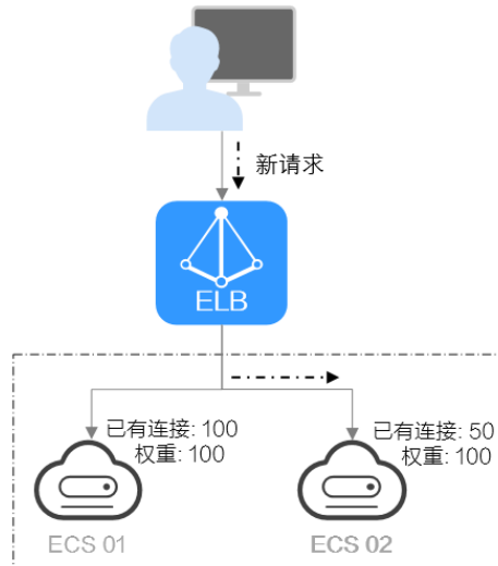
图 2-12 加权最少连接算法流量分发
