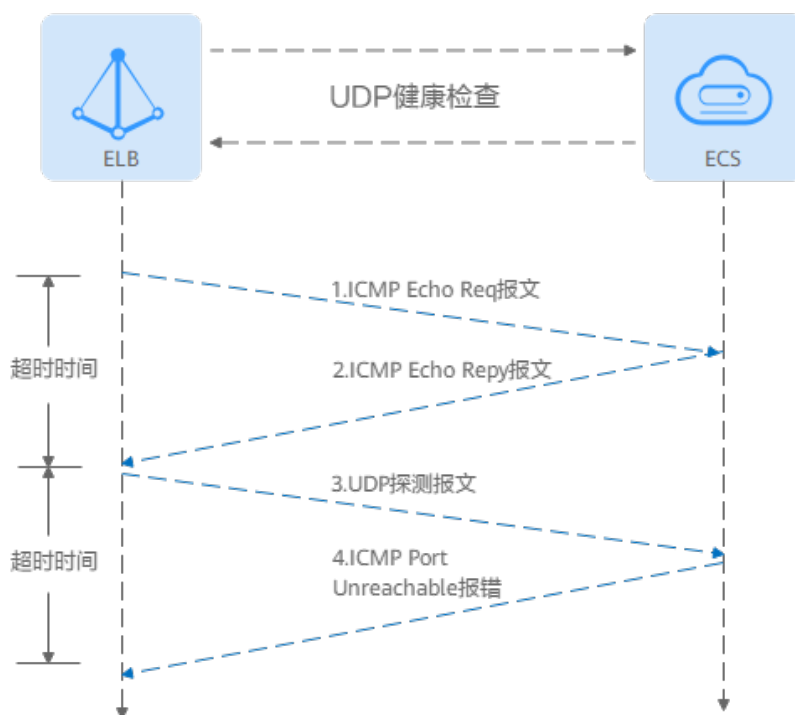
图 1-14 UDP 健康检查
