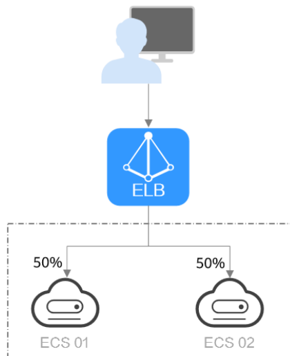
图 1-20 加权轮询算法流量分发
