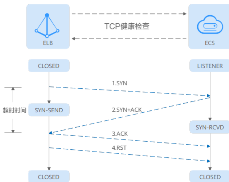
图 2-7 TCP 健康检查
