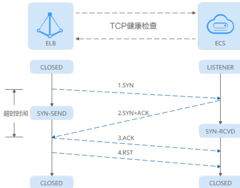
图 1-22 TCP 健康检查
