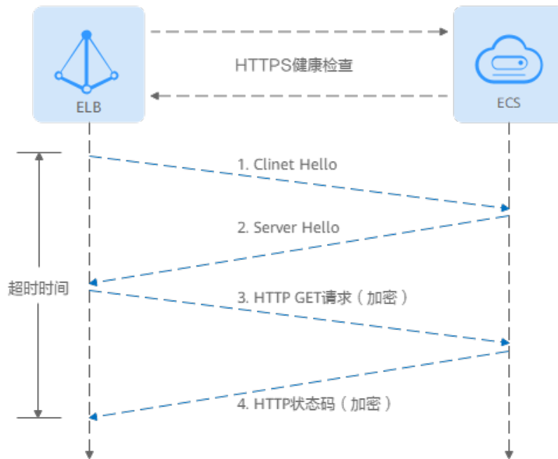
图 1-25 HTTPS 健康检查
