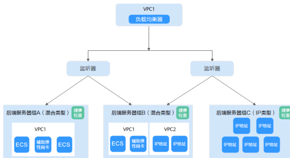
图 1-15 后端服务器组使用架构图
