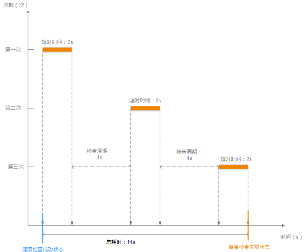
图 1-28 健康检查失败时间窗
