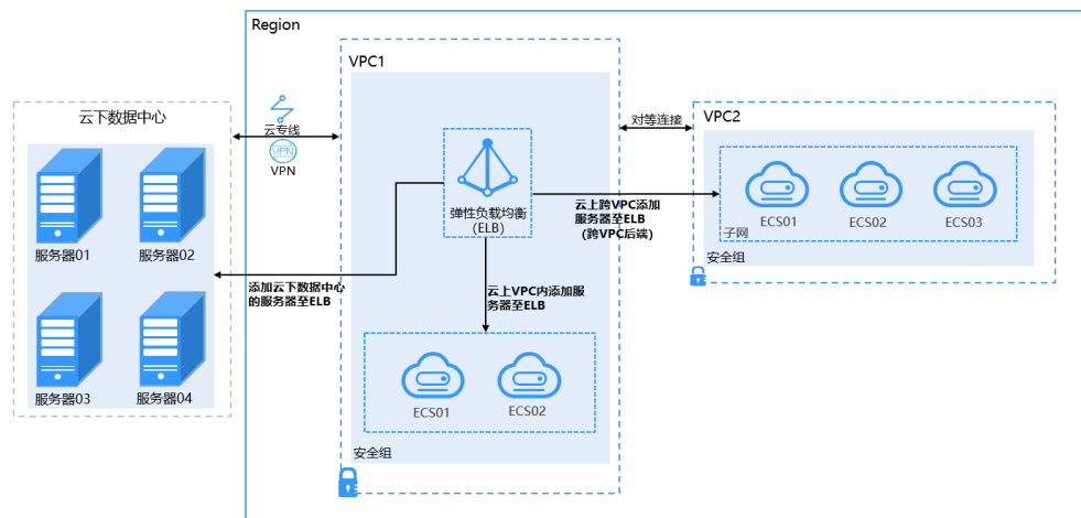
图 1-21 ELB 支持添加云上、云下的服务器
