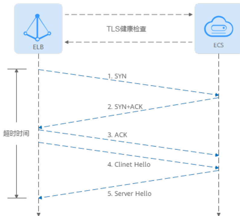
图 1-26 TLS 健康检查
