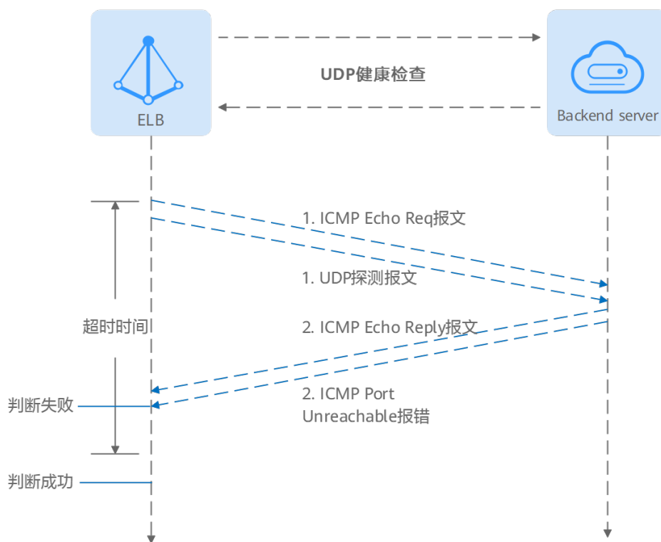
图 1-23 UDP 健康检查
