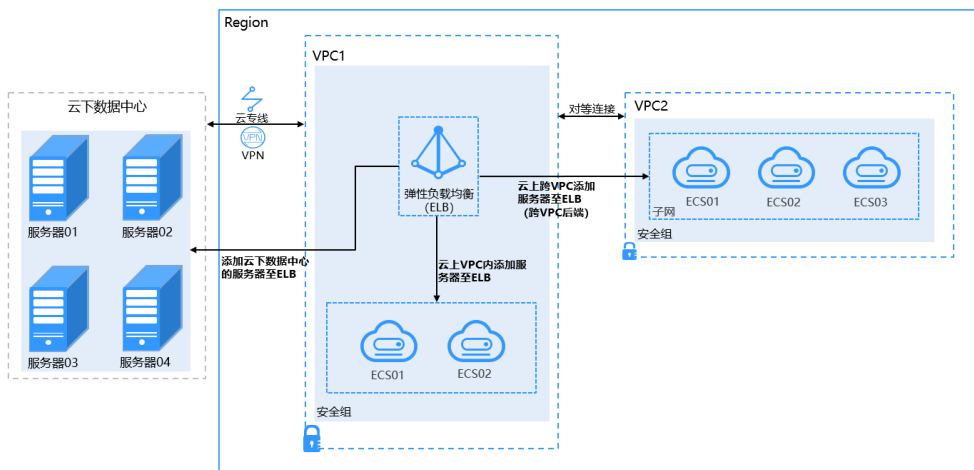
图 1-23 ELB 支持添加云上、云下的服务器
