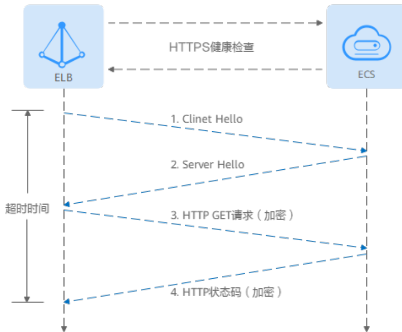
图 1-14 HTTPS 健康检查
