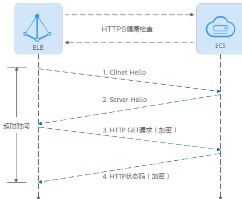
图 2-10 HTTPS 健康检查
